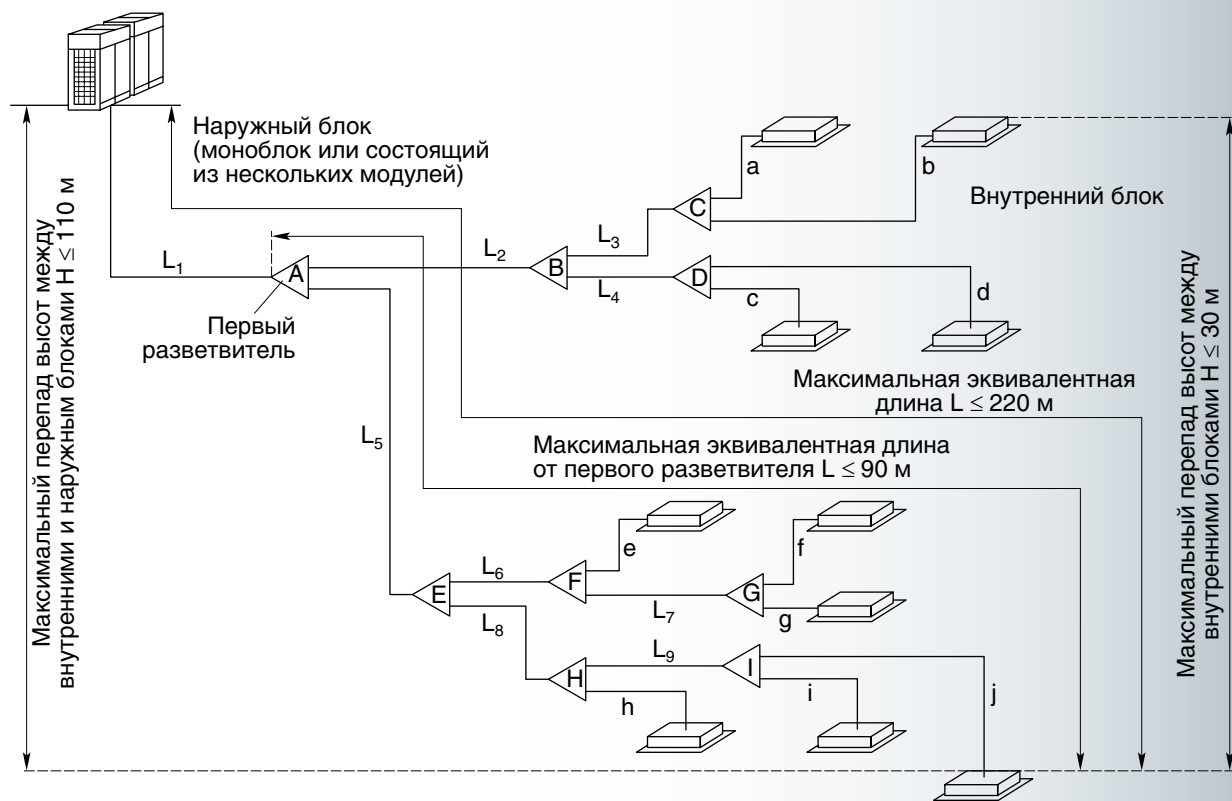
Рис. 1. Система трубопроводов мультизональной системы кондиционирования CMV
