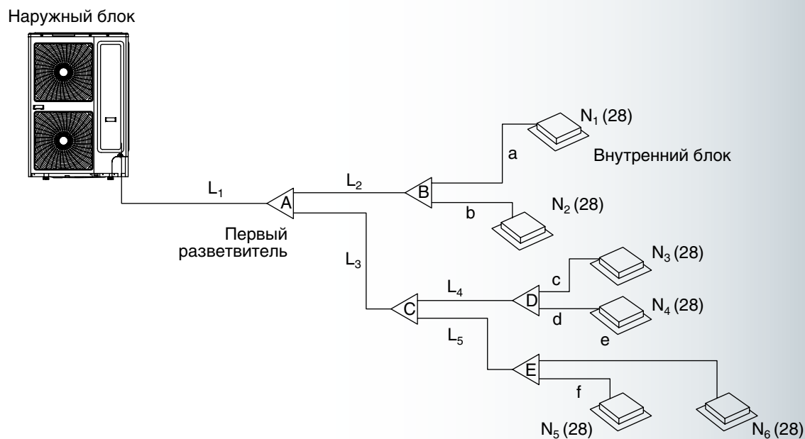
Рис. 2. Система трубопроводов мультizonальной системы кондиционирования CMV с модульным наружным блоком
