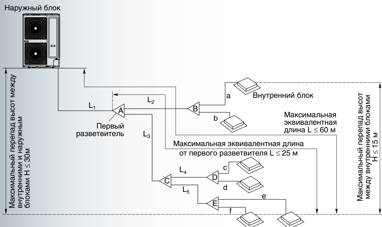
Рис. 1. Система трубопроводов мультizonальной системы кондиционирования MINI CMV
