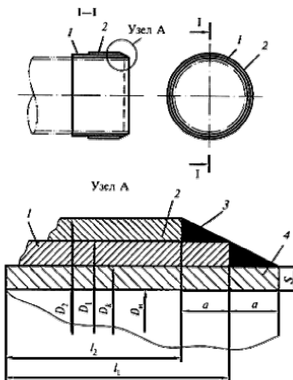
Рисунок 11 - Устройство кольцевого ножа на конце футляра
