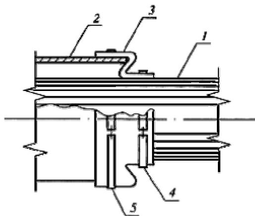
1 - трубная плетя; 2 - защитный футляр; 3 - резиновая манжета; 4 - малый хомут; 5 - большой хомут
