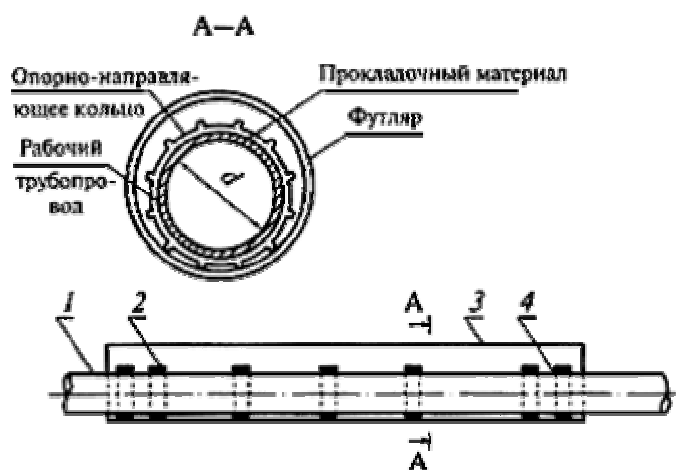
Рисунок 3 - Прокладка газопровода в футляре
