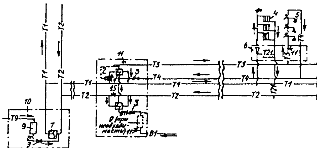
Рис. 1. Схема закрытой системы теплоснабжения
