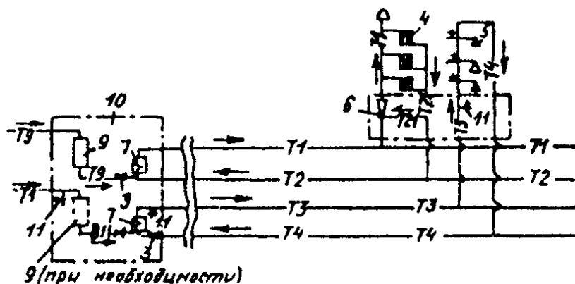
Рис. 3. Схема теплоснабжения с отдельными сетями горячего водоснабжения
