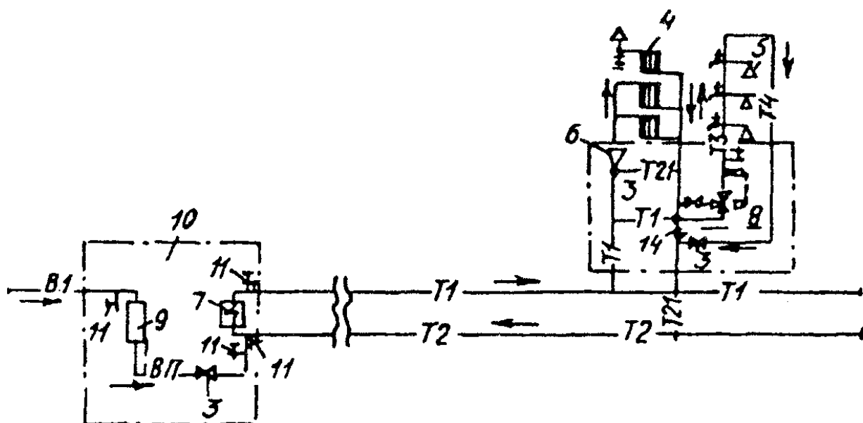
Рис. 2. Схема открытой системы теплоснабжения
