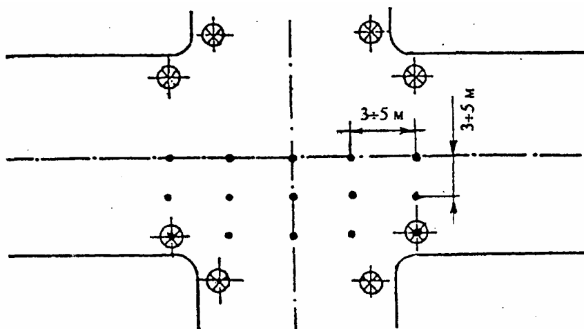
Рисунок А9 — Расположение контрольных точек при измерении средней освещенности улиц на перекрестке
