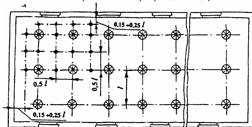
Расположение контрольных точек при проведении измерений
