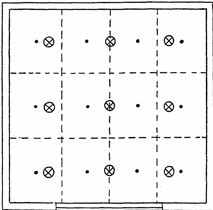
Рисунок А2 — Расположение контрольных точек при измерении минимальной освещенности помещения от светильников, принимаемых за линейные излучатели
