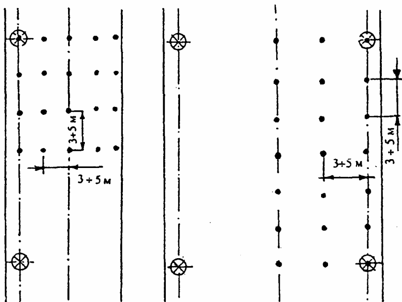
Рисунок А3 — Расположение контрольных точек при измерении средней освещенности в помещении
