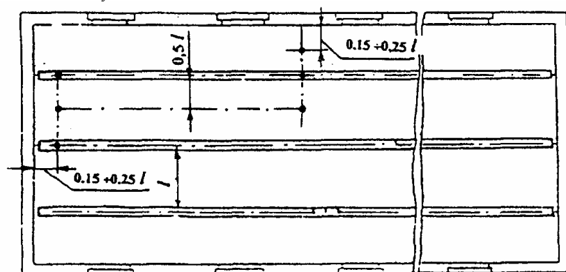
Рисунок А1 — Расположение контрольных точек при измерении минимальной освещенности помещения от светильников, принимаемых за точечные излучатели
