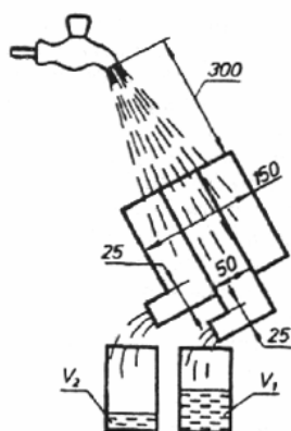
Рисунок 1 - Схема определения компактности струи
