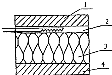
Рисунок А.1 — Схема прибора с одним тепломером
