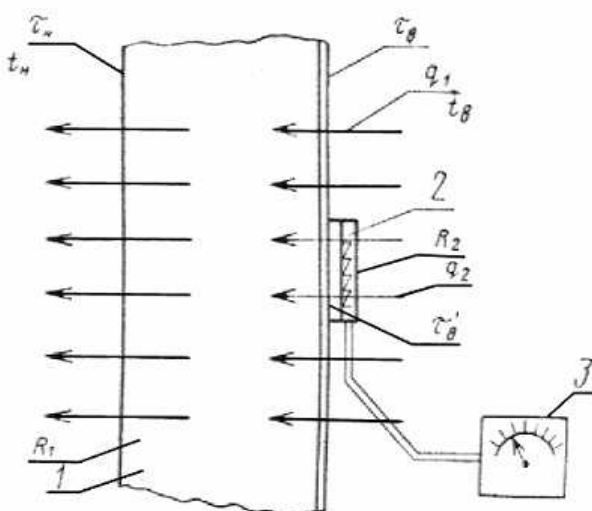
Схема измерения плотности теплового потока
