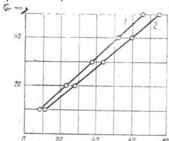
Чертеж В.1 - Градуировочные зависимости для продольных стержней диаметром 16 мм
