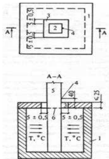
Черт. 3. Схема установки на огневую печь
