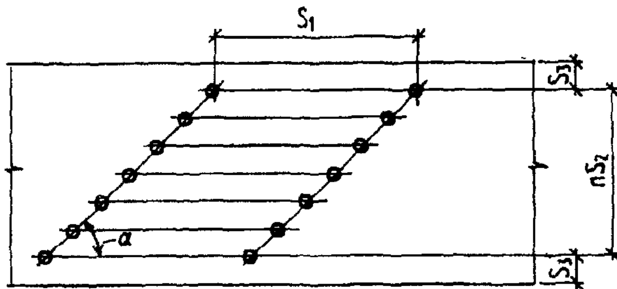
Рис. 12. Расстановка гвоздей косыми рядами
