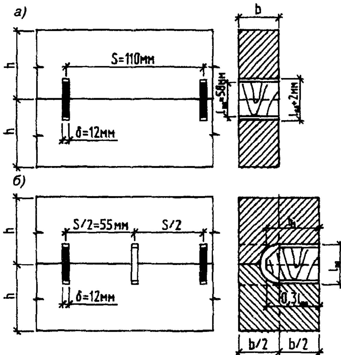
Рис. 13. Соединение на пластинчатых нагелях
