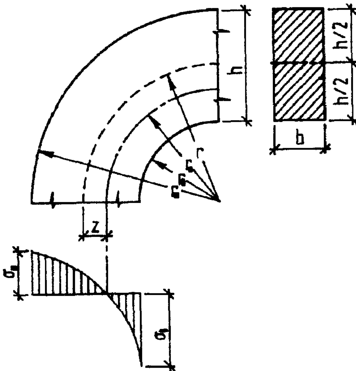
Рис. 16. Расчетная схема к определению напряжений в криволинейной части клееной рамы
