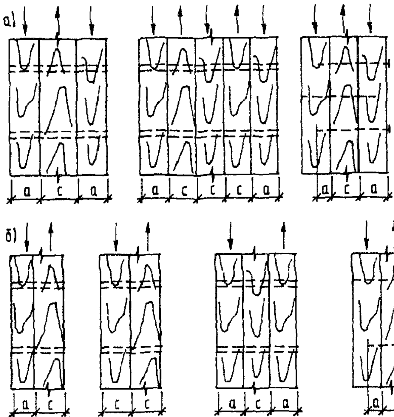
Рис. 8. Нагельные соединения
