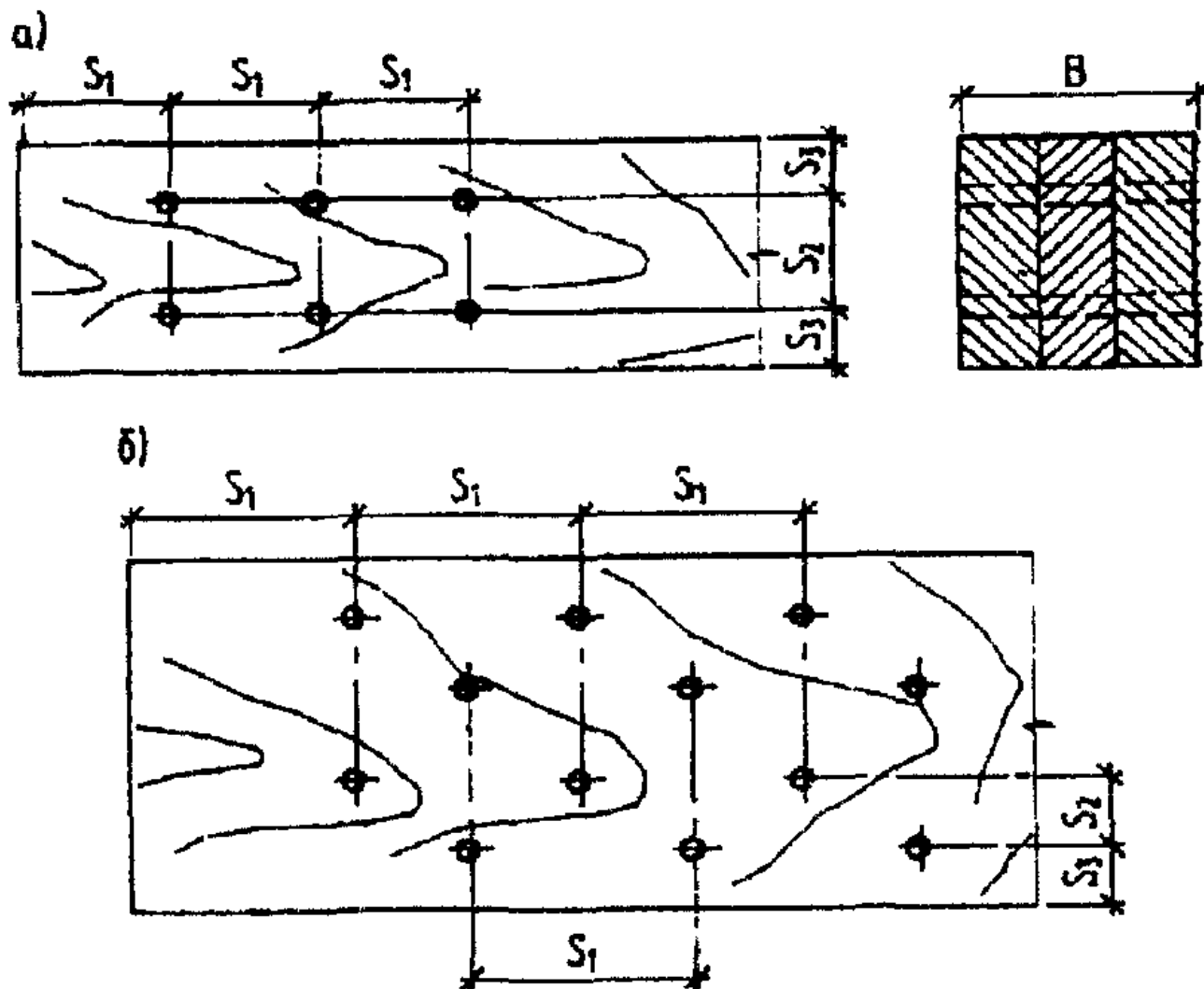
Рис. 10. Расстановка нагелей
