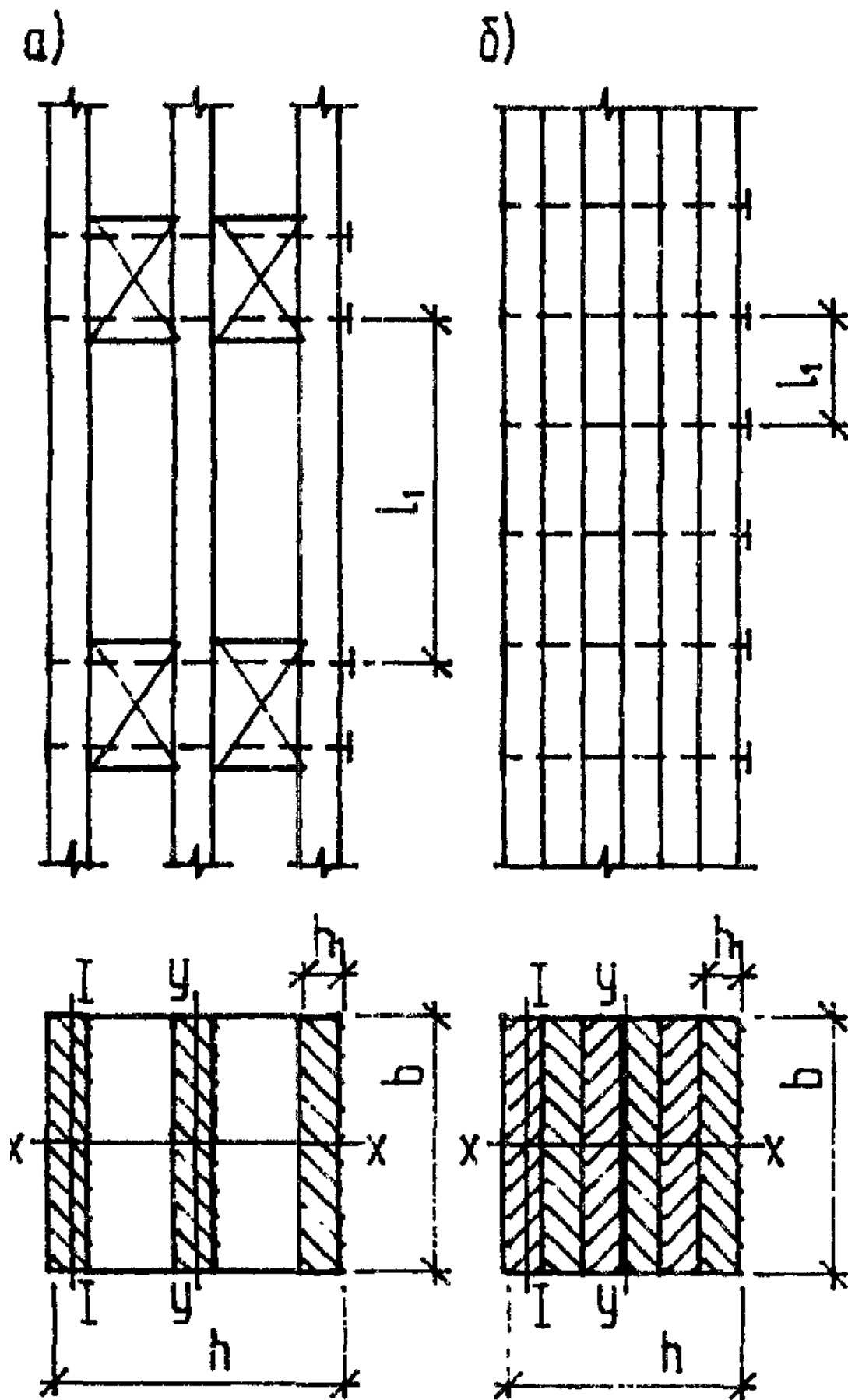
Рис. 2. Составные элементы
