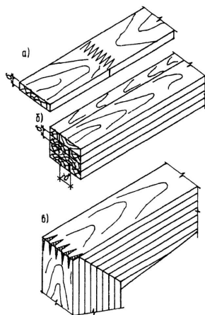
Рис. 6. Клеевые соединения
