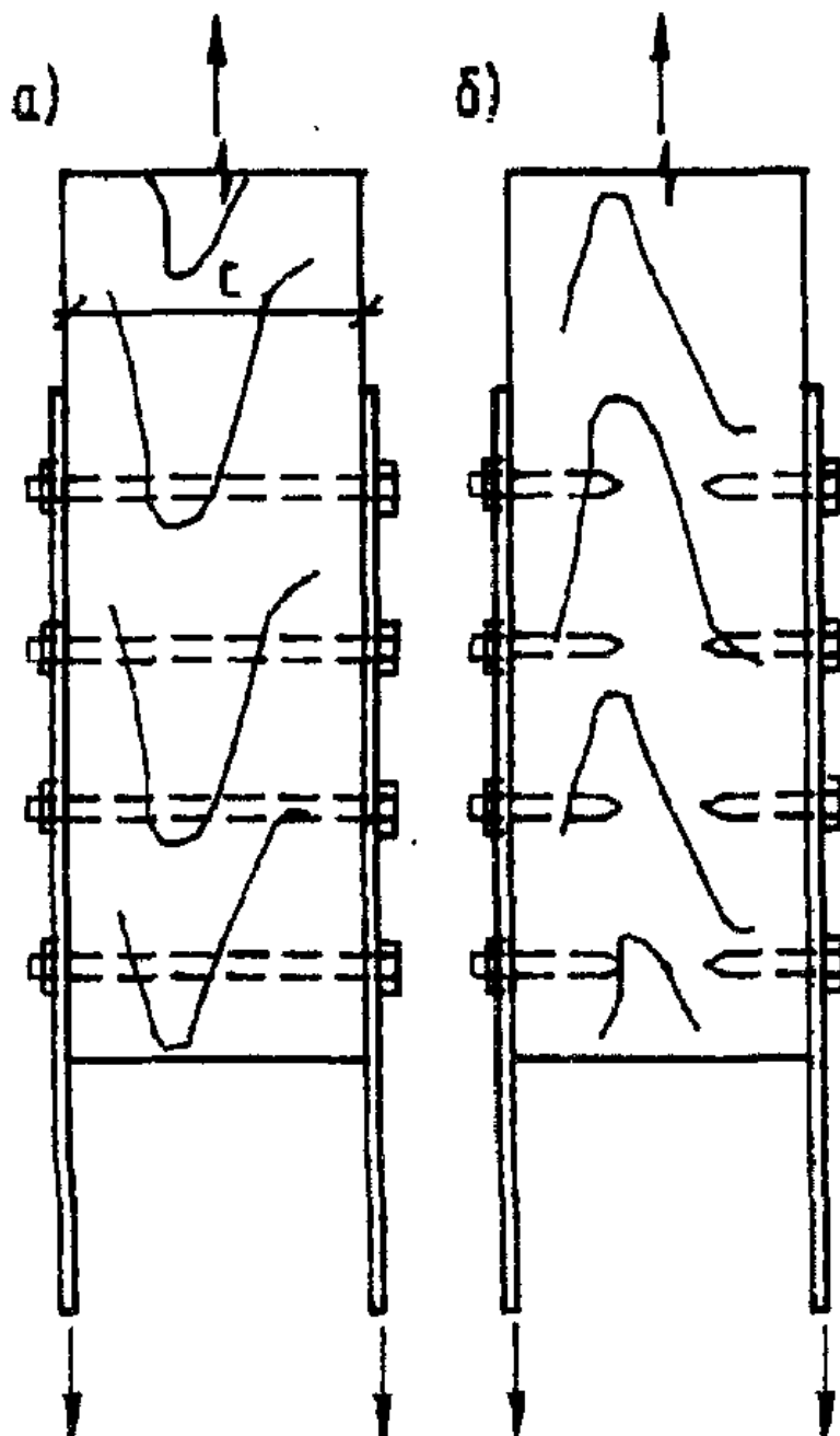
Рис. 9. Нагельные соединения со стальными накладками
