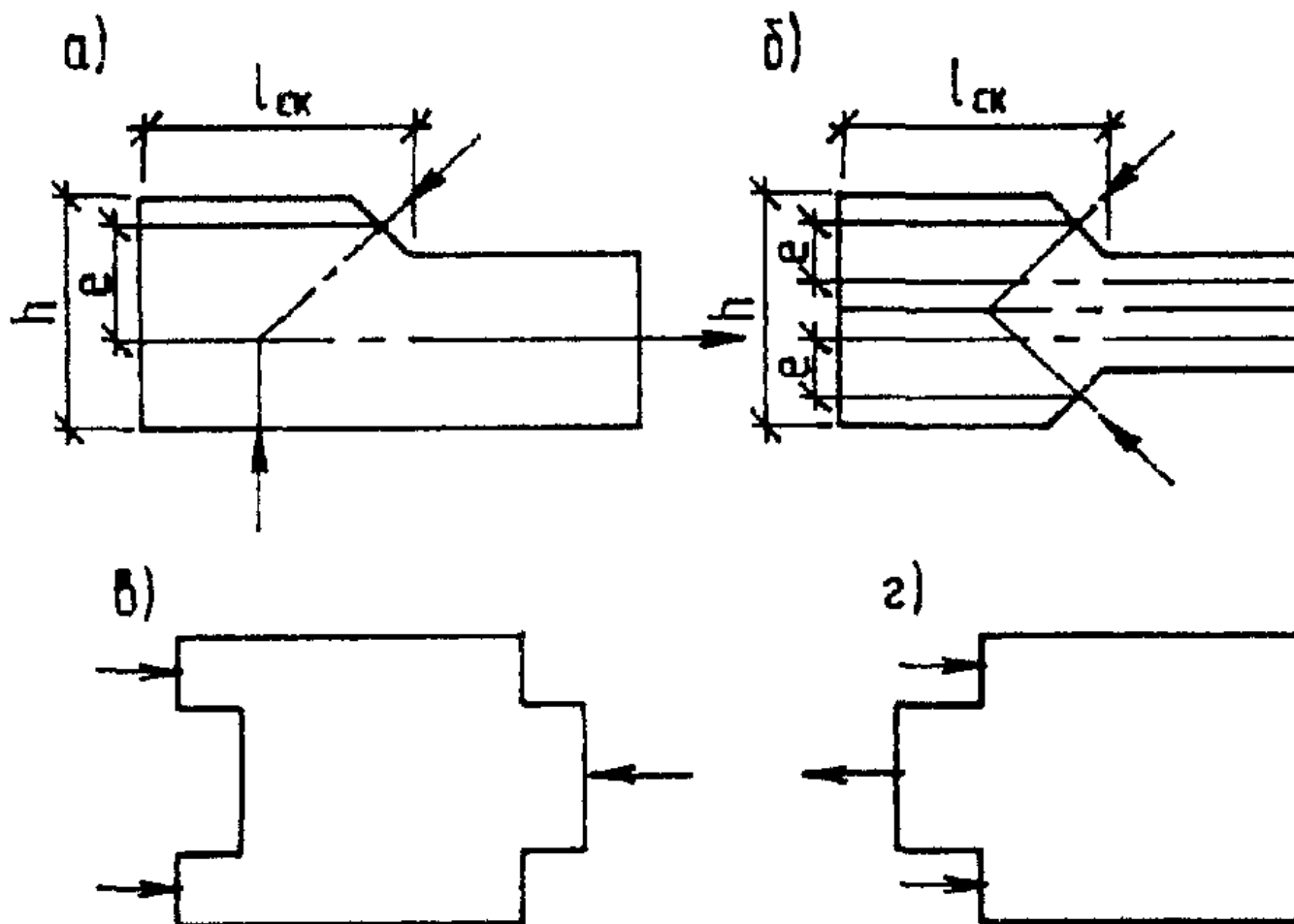
Рис. 5. Врезки в элементах соединений
