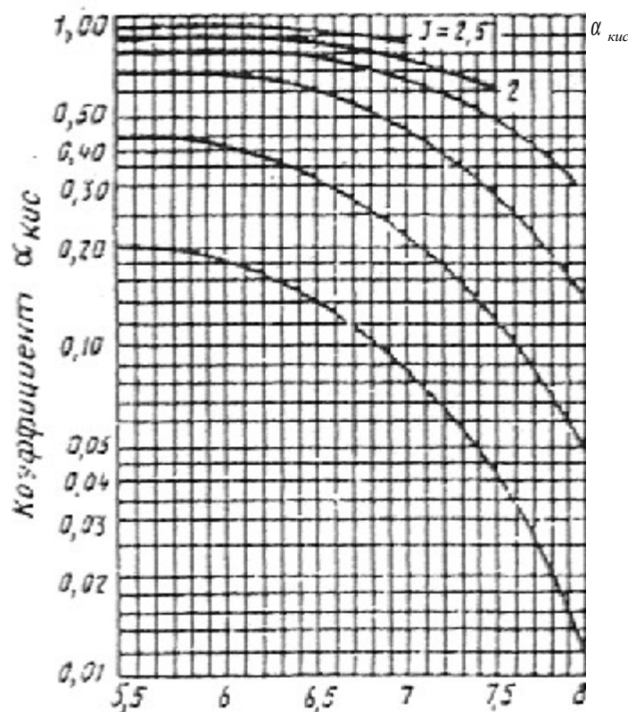
Рис. 3. Номограмма для определения коэффициента при расчете дозы кислоты
