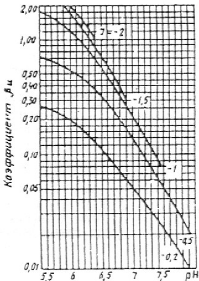
Рис. 4. Номограмма для определения коэффициента
