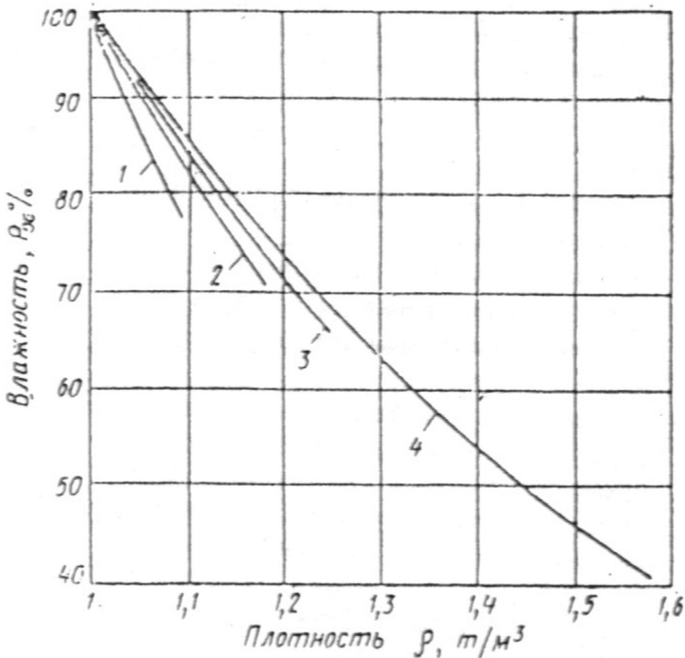
Рис. 5. Значения плотности в зависимости от влажности осадка станций осветления и обесцвечивания воды
