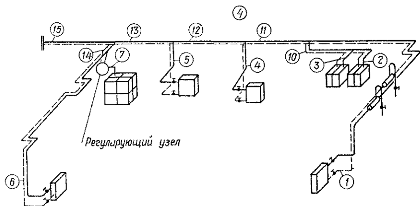
Лист Х.2. Схемы установки и подключения калориферов и схема системы теплоснабжения:
