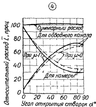
Лист VIII. 4. Оросительные камеры, расчетные графики и схемы:
