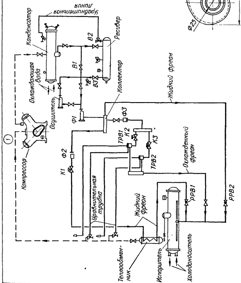
Лист VIII.20. Принципиальные схемы:
