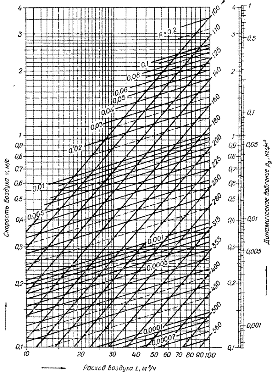
Лист VII.7. Номограмма для расчета круглых стальных воздуховодов при расходах воздуха до 100 м³/ч (при K = 0,1 ; \gamma = 1,2 кг/м³).
