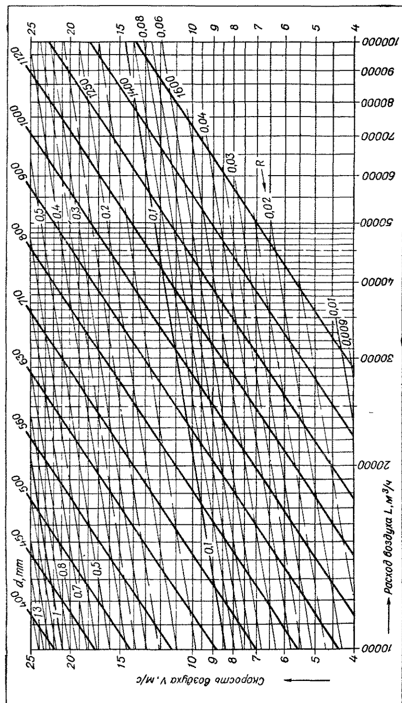
Лист VII.10. Номограмма для расчета круглых стальных воздухопроводов при расходах воздуха от 10 000 до 100 000 m^3/ч и скорости воздуха от 4 до 25 m/c (при K = 0,1 , \gamma = 1,2 \text{ кг}/m^3 ).
