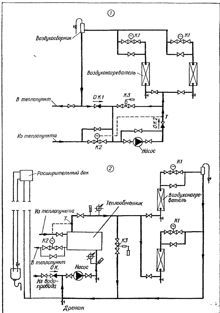
Лист VIII.18. Принципиальные схемы теплоснабжения калориферов второго, местного и зонального подогрева:
