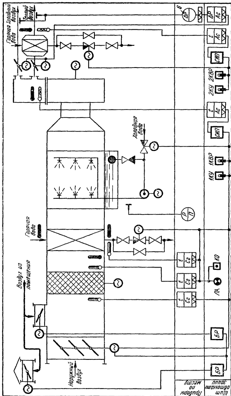
Лист IX.16. Функциональная схема автоматического регулирования двухканальной СКВ с электроавтоматикой.
