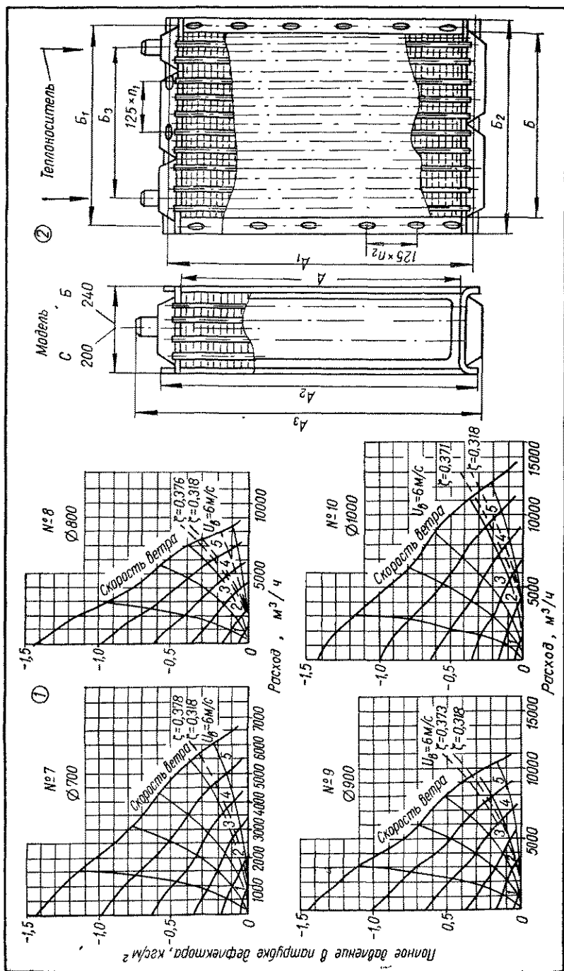
Лист VII.18. Аэродинамические характеристики дефлекторов УкрНИИСТ ДВК-5 № 7—10 (рис. 1) и многоходовых калориферов типа КВС, КВБ, КМС и КМБ (рис. 2).
