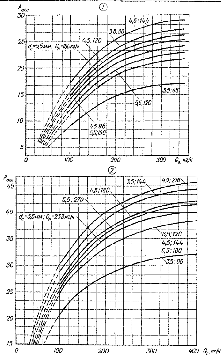
Лист VIII. 13. Удельный показатель A_{oxl} в двухрядном теплообменнике ЭКД: 1 — типа КНЭ-У-0,8А; 2 — типа КНЭ-У-1,2.
