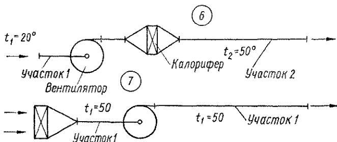
Лист VII.24. Вентилятор Ц4-70 № 16, исполнение 6:
