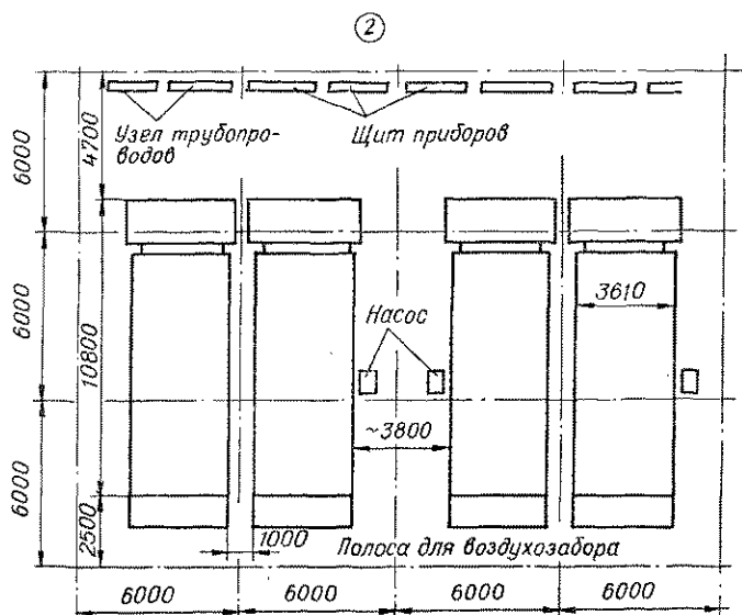
Лист VIII.8. Размещение прямоточных кондиционеров; 1 — КТ-30 и КТ-40; 2 — КТ-60 и КТ-80.
