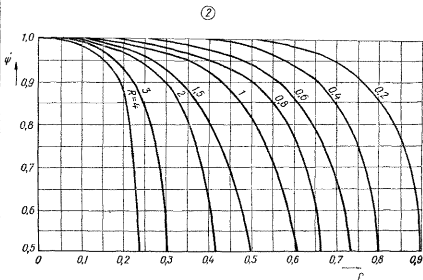
Лист VIII.6. К расчету поверхностных воздухоохладителей:
