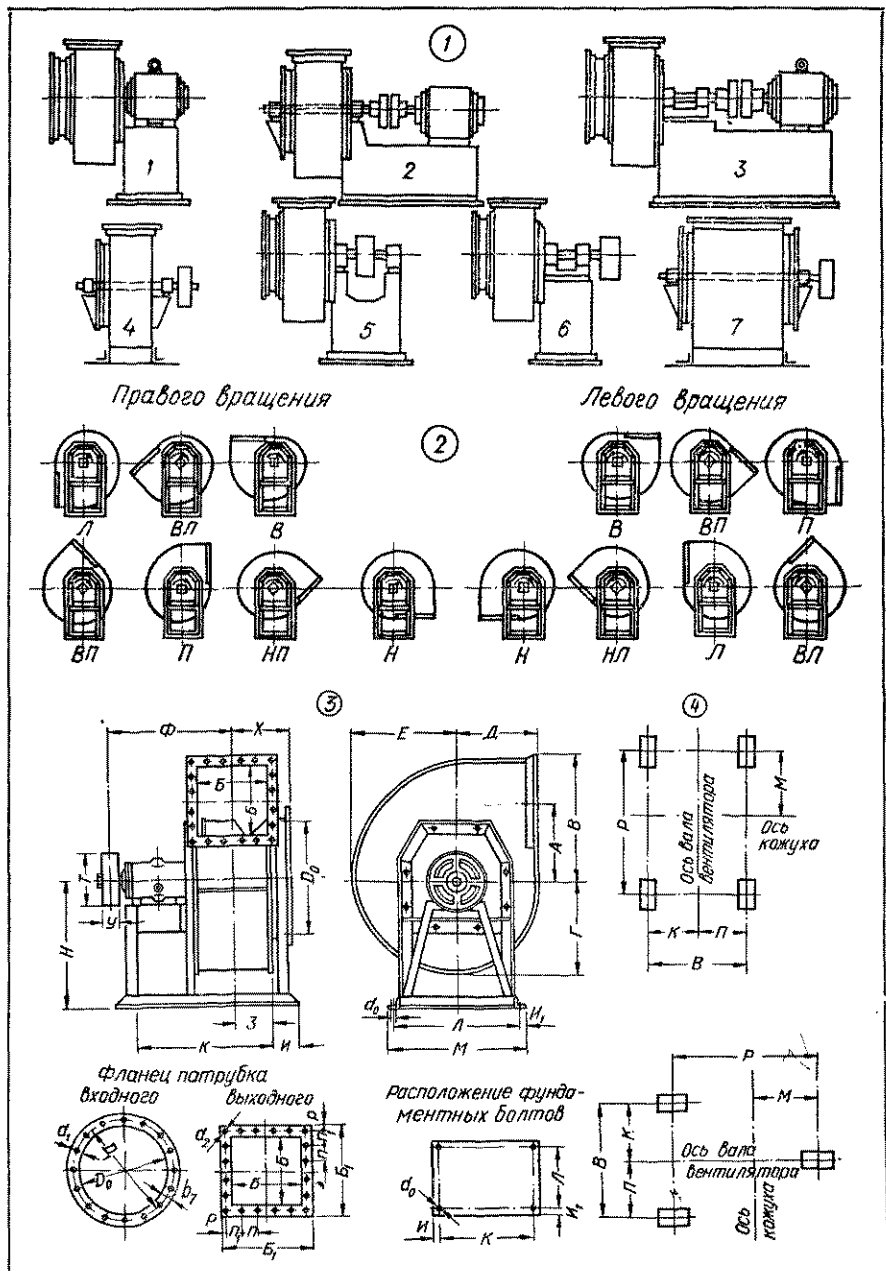
Лист VII.21. Принципиальные схемы конструктивного исполнения центробежных вентиляторов:
