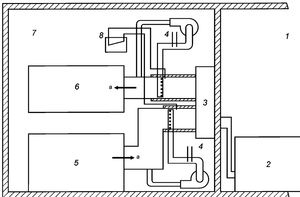
1 — отсек наружной стороны; 2 — наружный блок испытываемого оборудования; 3 — внутренний блок испытываемого оборудования; 4 — измерительные приборы температуры и влажности; 5 — аппарат повторного кондиционирования; 6 — аппаратура измерения воздушного потока; 7 — отсек внутренней стороны; 8 — аппаратура измерения перепада давления; а — воздушный поток
