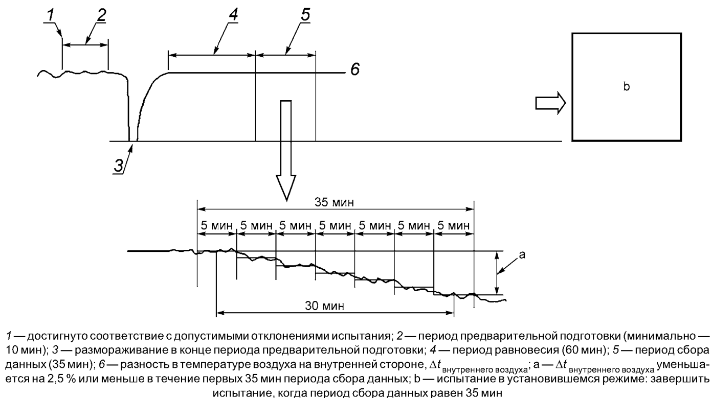
Рисунок Н.2 — Испытание теплопроизводительности в установившемся режиме
