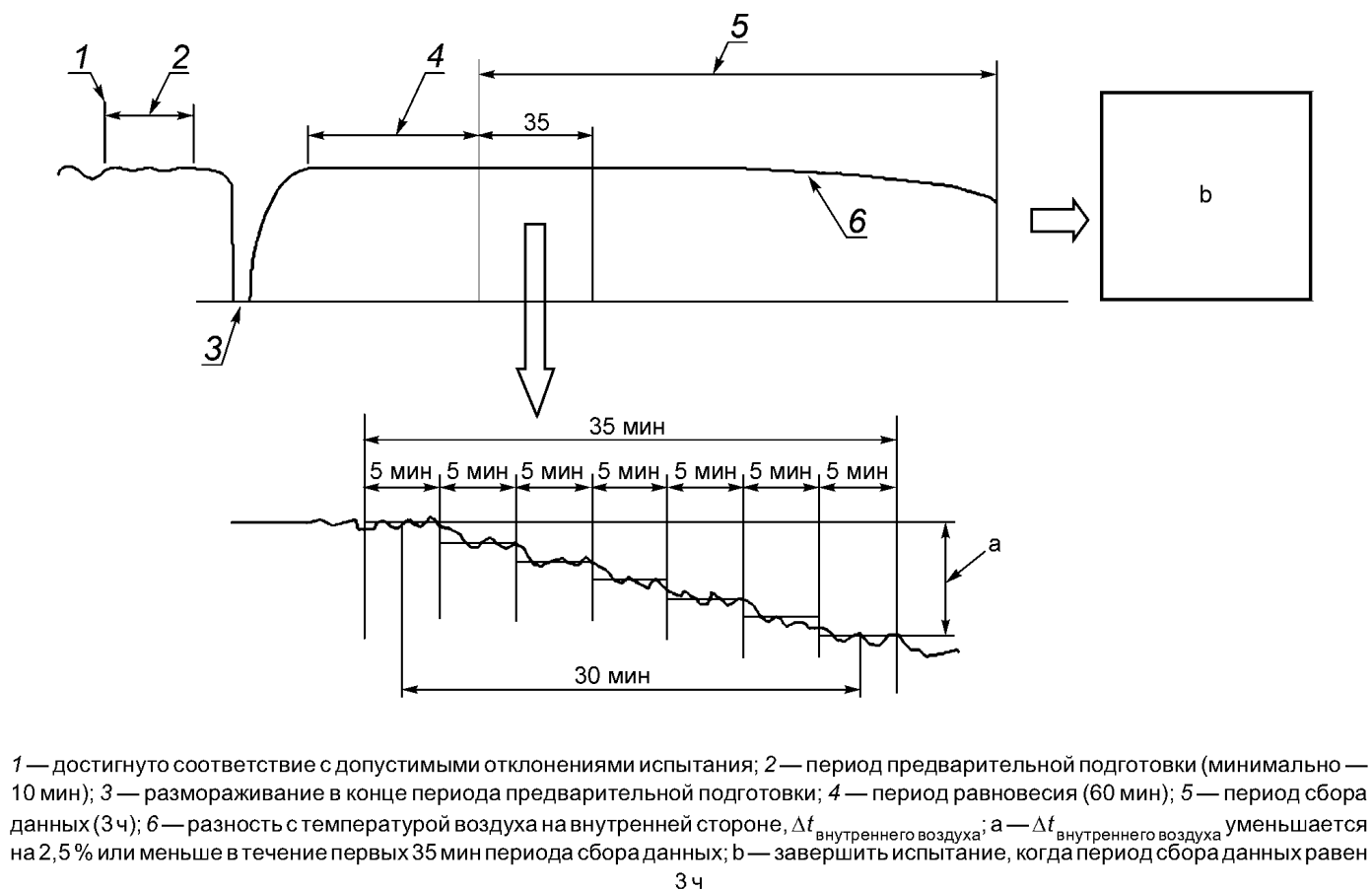
Рисунок Н.3 — Испытание теплопроизводительности в режиме переходного процесса без циклов размораживания
