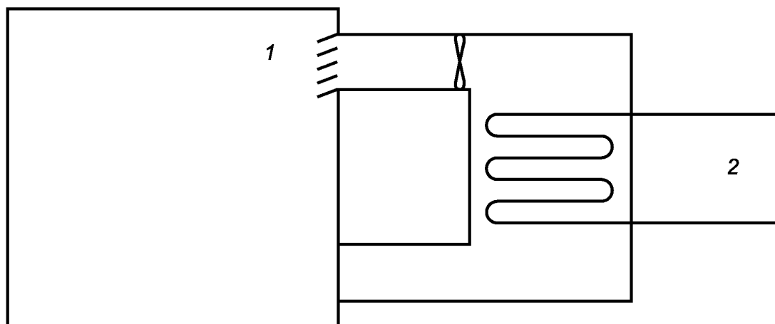
Рисунок 3 — Система непосредственного охлаждения с воздухопроводом
