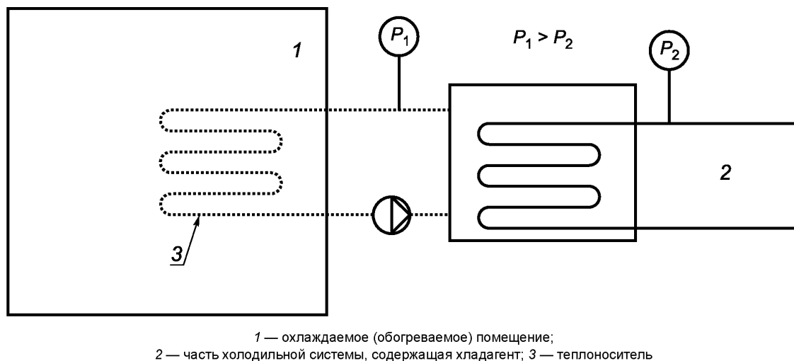
Рисунок 9 — Промежуточная система высокого давления
