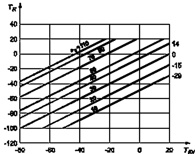
T_R — расчетная эталонная температура; T_KV — температура испытания материала на удар; e_s — эталонная толщина Рисунок Г.5 — Расчетная эталонная температура и температура испытания на удар, условия термообработки после сварки PWHT, для Y_s 460 МПа и KV 2 40 Дж
