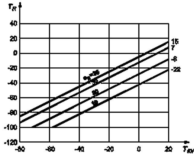
T_R — расчетная эталонная температура; T_{KV} — температура испытания материала на удар; e_s — эталонная толщина Рисунок Г.4 — Расчетная эталонная температура и температура испытания на удар в состоянии после сварки AW для Y_s S 355 МПа и KV 27 Дж
