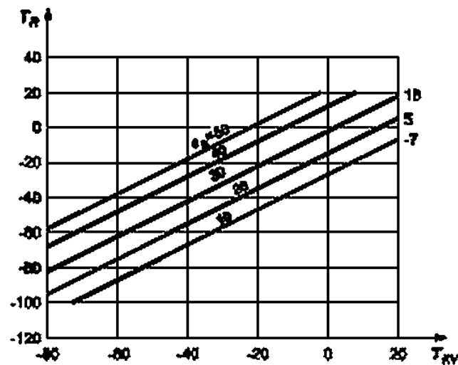
Рисунок Г. 10 — Расчетная эталонная температура и температура испытания на удар аустенитно-ферритных сталей в состоянии после сварки AW. для R_e \leq 485 МПа и KV \geq 40 Дж
