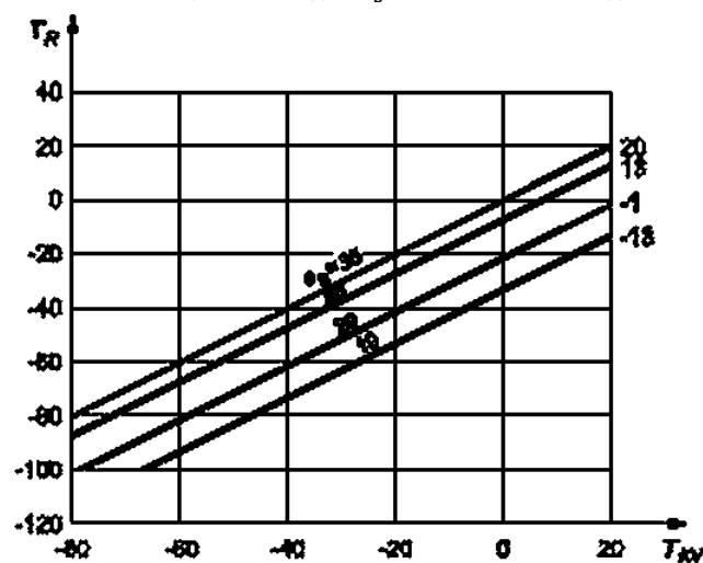
T_R — расчетная эталонная температура; T_{KV} — температура испытания материала на удар; e_s — эталонная толщина Рисунок Г.6 — Расчетная эталонная температура и температура испытания на удар в состоянии после сварки AW для Y_s 460 МПа и KV 2 40 Дж
