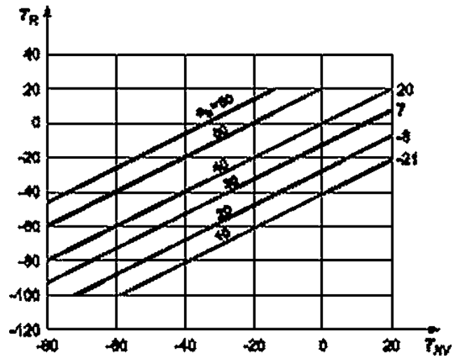
Рисунок Г.7 — Расчетная эталонная температура и температура испытания на удар, условия термообработки после сварки PWHT. для R_e \leq 500 МПа и KV 2 40 Дж
