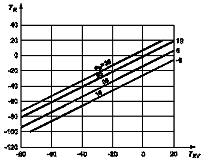
Рисунок Г.в — Расчетная эталонная температура и температура испытания на удар в состоянии после сварки AW для R_e \leq 500 МПа и КУ г 40 Дж
