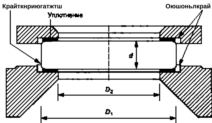
Рисунок Е.1 — Определение и D_2
