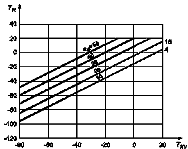
Рисунок Г.11 — Расчетная эталонная температура и температура испытания на удар аустенижно-ферритных сталей в состоянии после сварки AW. для R_y S 550 МПа и KV 2 40 Дж
