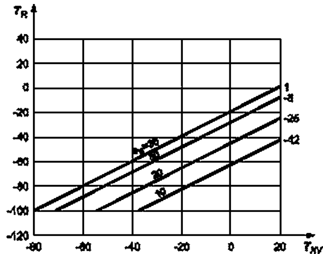
Рисунок Г.2 — Расчетная эталонная температура и температура испытания на удар в состоянии после сварки AW для R_e S 265 МПа и KV_i 27 Дж
