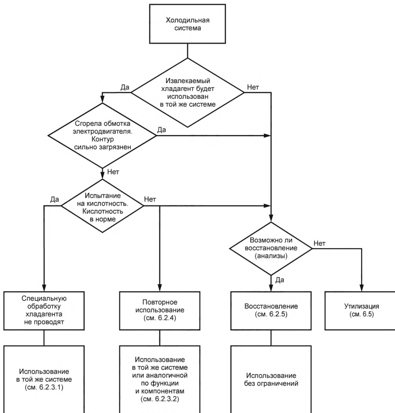
Рисунок 2 — Операции с извлекаемым хладагентом
