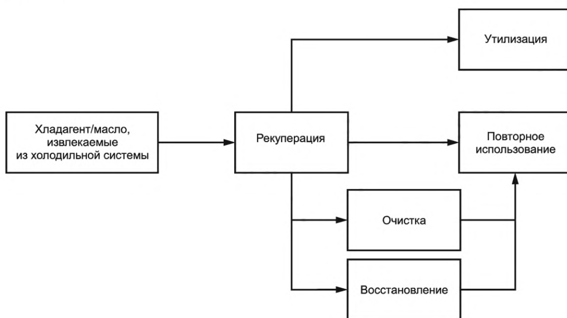
Рисунок 1 — Упрощенная схема взаимосвязи между процессами
