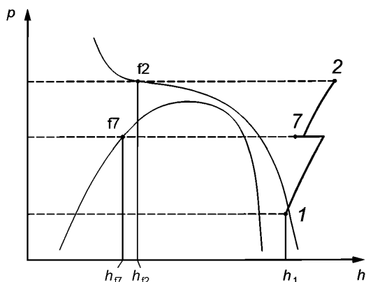
c — Диаграмма давление-энтальпия (сверхкритический режим)
