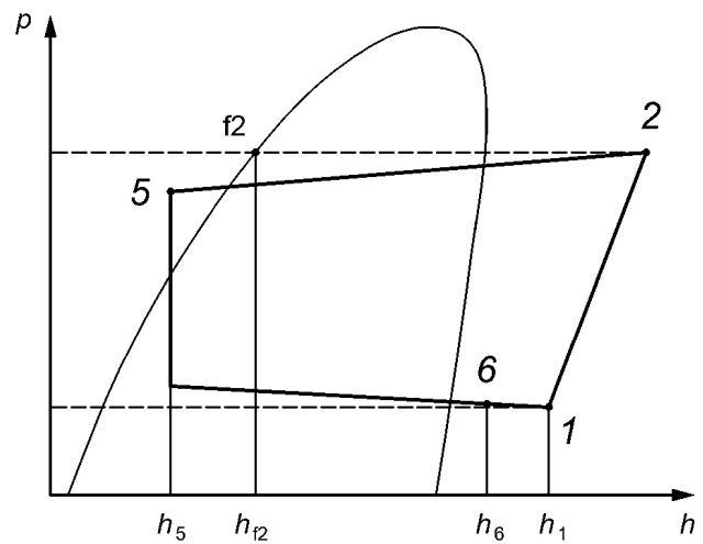
б – Диаграмма давление–энтальпия (докритический режим)
