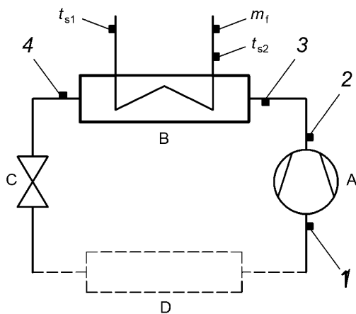
а – Схема цикла
