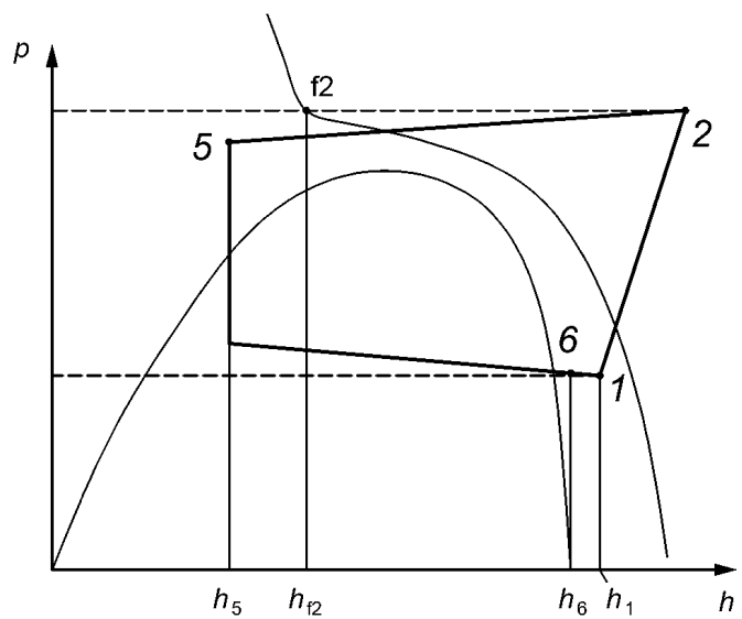
с – Диаграмма давление–энтальпия (сверхкритический режим)
