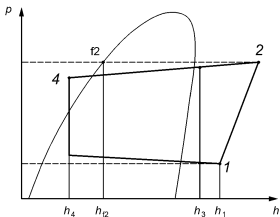
b – Диаграмма давление–энтальпия (докритический режим)
