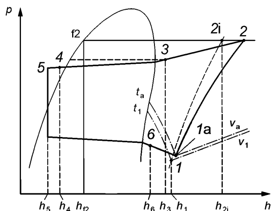
b — Диаграмма давление — энтальпия
