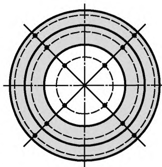
Рисунок 2 — Пример секционирования измеряемой зоны (круговая зона)
