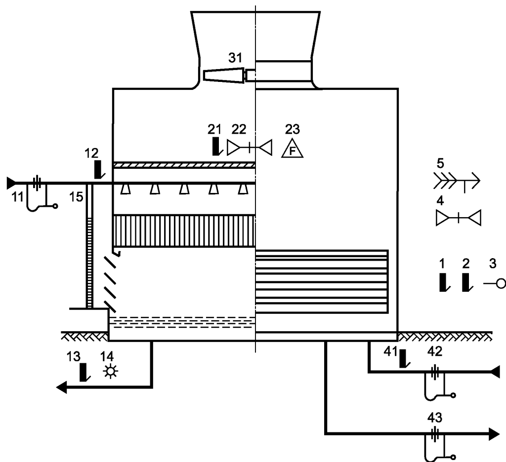
Рисунок 4 — Расположение точек измерений в вентиляторной градирне
