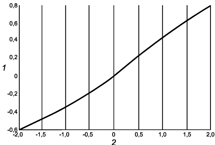
Рисунок 6 — Влияние градиента на температуру холодной воды
