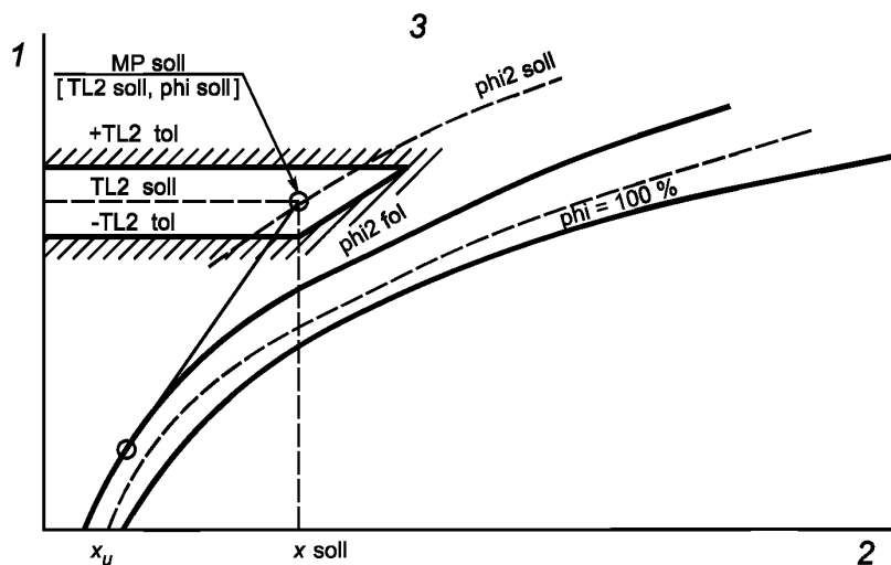
1 — массовая энтальпия воздуха h ; 2 — абсолютная влажность окружающего воздуха x ; 3 — диаграмма Мольера
