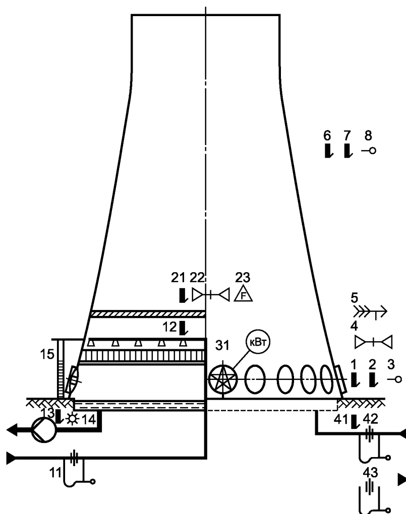
Рисунок 3 — Расположение точек измерения для градирни с естественной тягой, усиленной вентилятором
