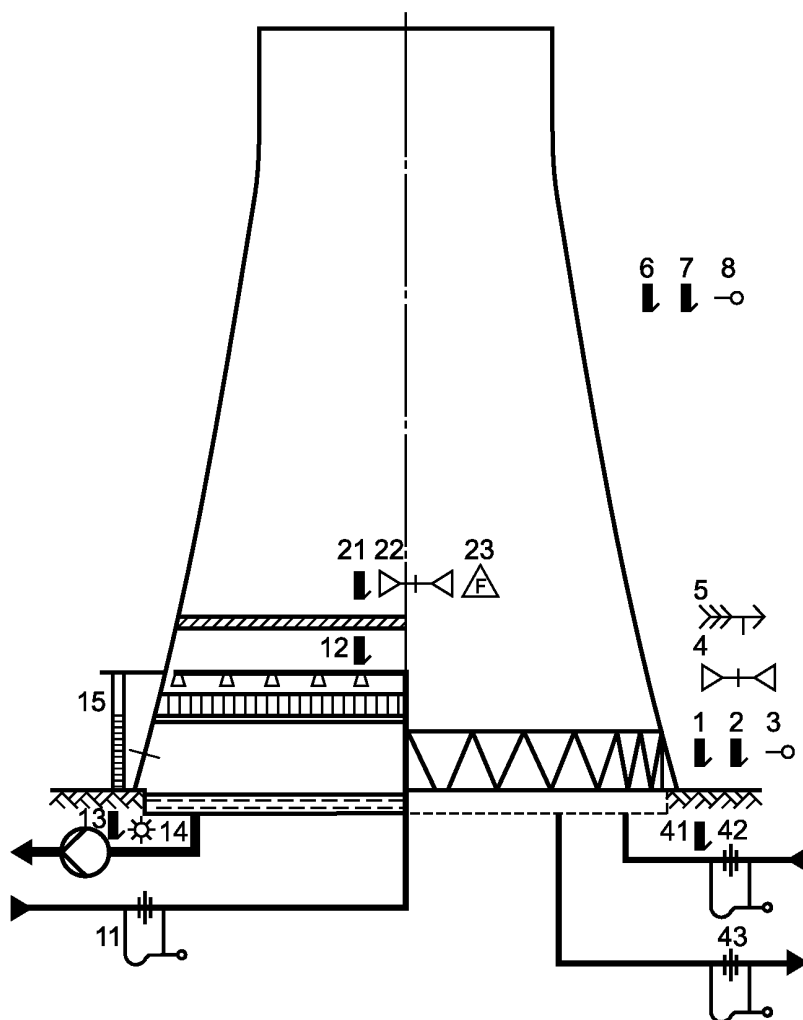
Рисунок 5 — Расположение точек измерений в испарительной градирне с естественной тягой
