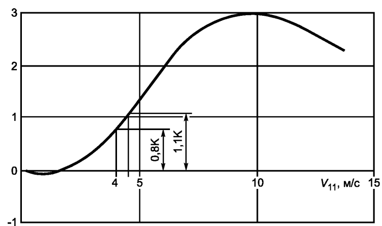
Рисунок А.2 — Пример воздействия ветра на гравирню с противотоком и естественной тягой
