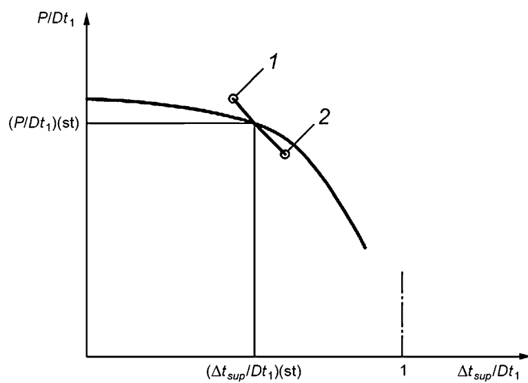
Рисунок Г.1 — Перегрев и холодопроизводительность
