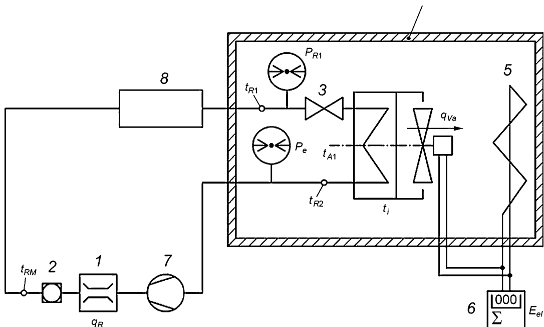
Рисунок Б.1 — Испытательное оборудование для работы в режиме прямого расширения
