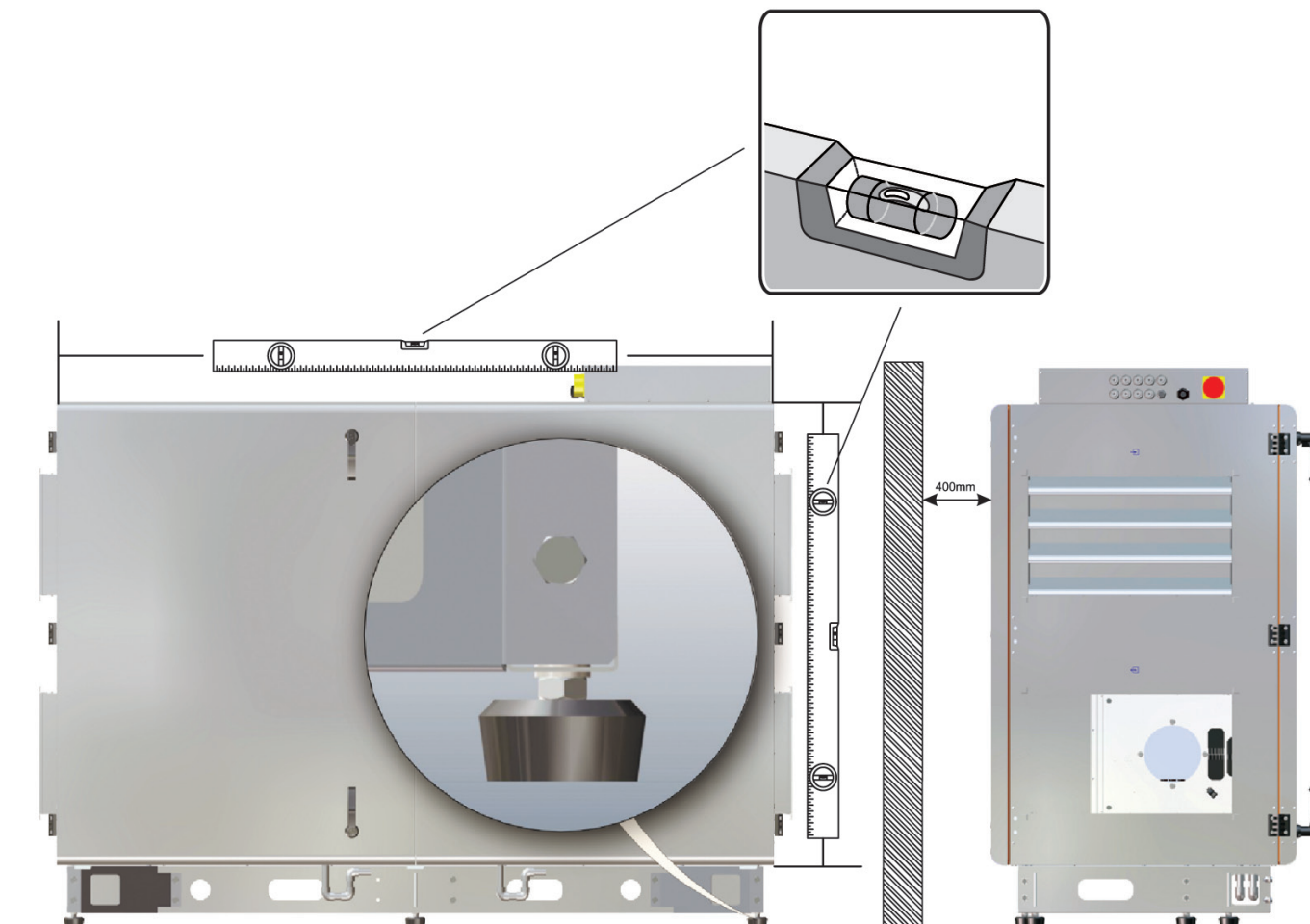
Рис. 1 Монтаж вентагрегата.
