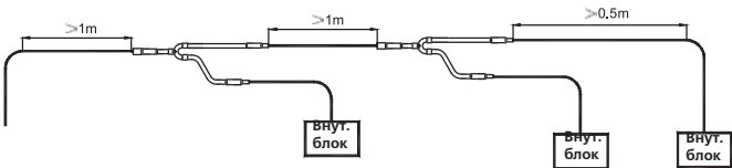
Протяженность горизонтальных участков фреонопровода
