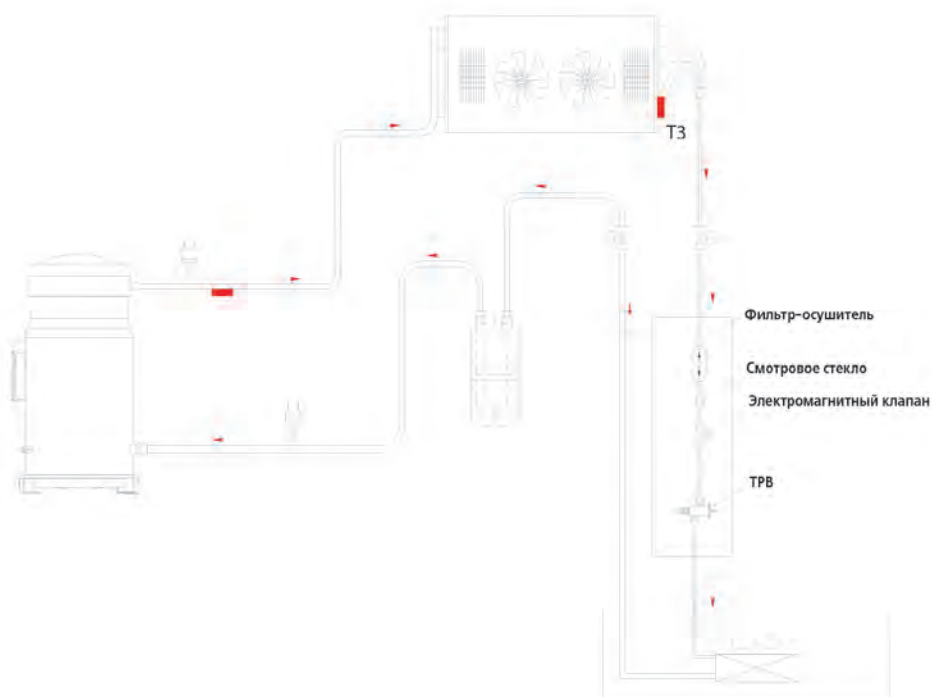
Схема подключения компрессорно-конденсаторного блока с секцией воздухоохладителя центрального кондиционера
