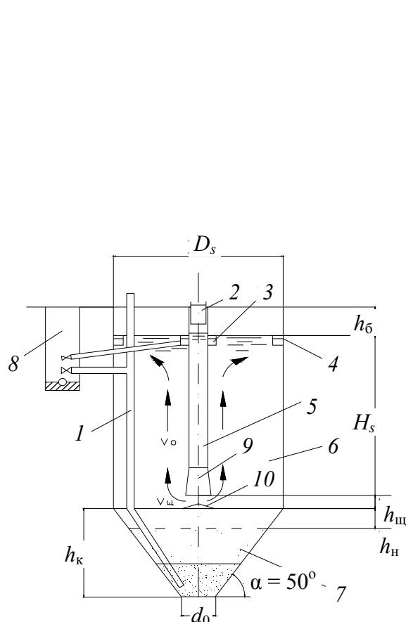
Рис. 3.2.8. Вертикальный отстойник: 1 – иловая труба для удаления осадка; 2 – подводящий лоток сточных вод; 3 – лоток круговой для сбора корки с поверхности воды; 4 – кольцевой сборный лоток; 5 – центральная труба; 6 – отстойная часть; 7 – коническая часть для сбора осадка; 8 – иловый колодец; 9 – раструб на центральной трубе; 10 – щель для выпуска воды
