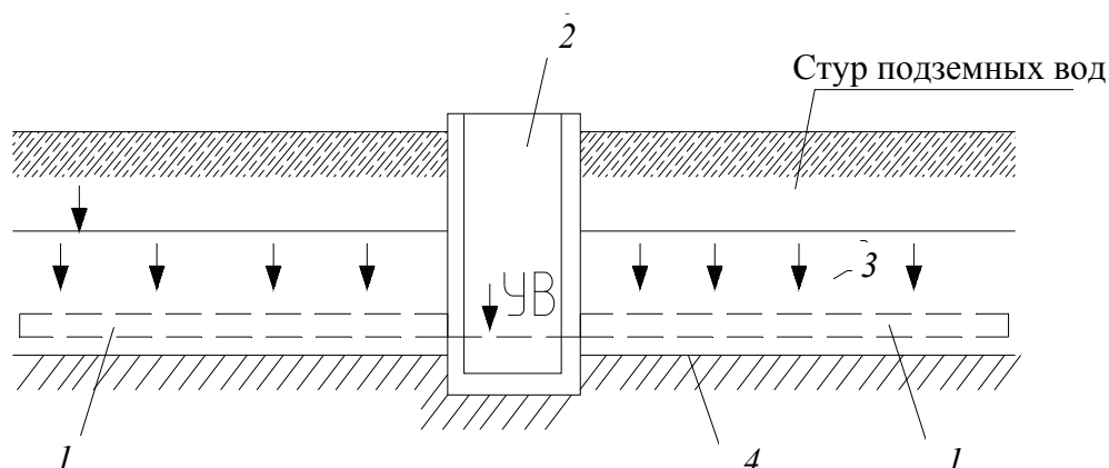
Рис. 1.7.2. Горизонтальный водозабор: 1 – горизонтальные водосборники; 2 – сборный колодец; 3 – водоносный пласт; 4 – водоупор
