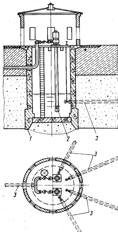
Рис. 1.7.1. Схема устройства лучевого водозабора: 1 – колодец (водоприемная камера); 2 – насос; 3 – дренажные трубы (горизонтальные скважины)
