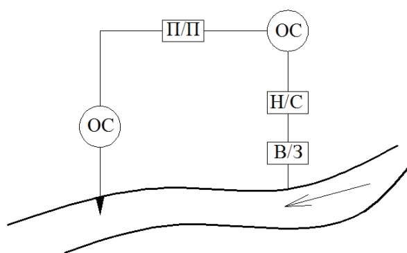
Рис. 1.1.3. Прямоточная схема водоснабжения промышленного предприятия: П/П – промышленное предприятие; В/З – водозаборные сооружения; Н/С – насосная станция; ОС – очистные сооружения
