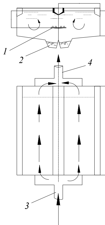
Рис. 3.2.6. Аэрируемая песколовка: 1 – пористые или дырчатые трубы; 2 – прямок; 3 – впуск воды; 4 – выпуск очищенной воды
