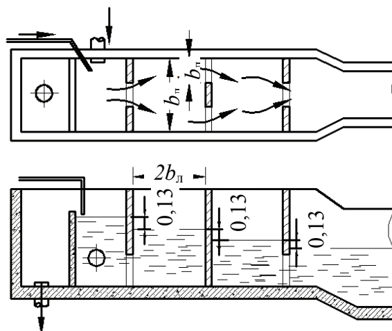
Рис. 1.8.3. Перегородчатый смеситель
