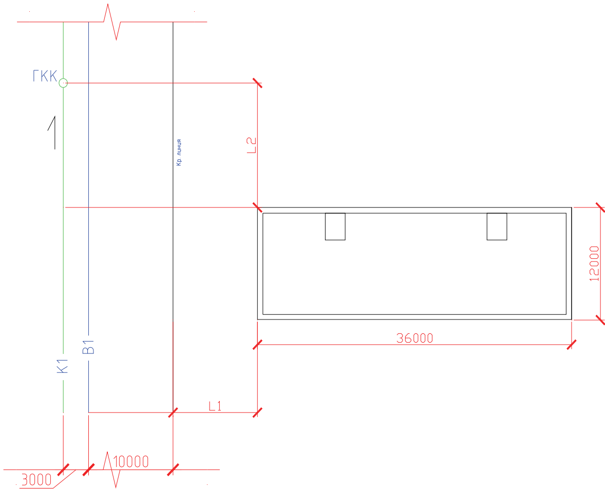
Рис. 1. Генплан участка
