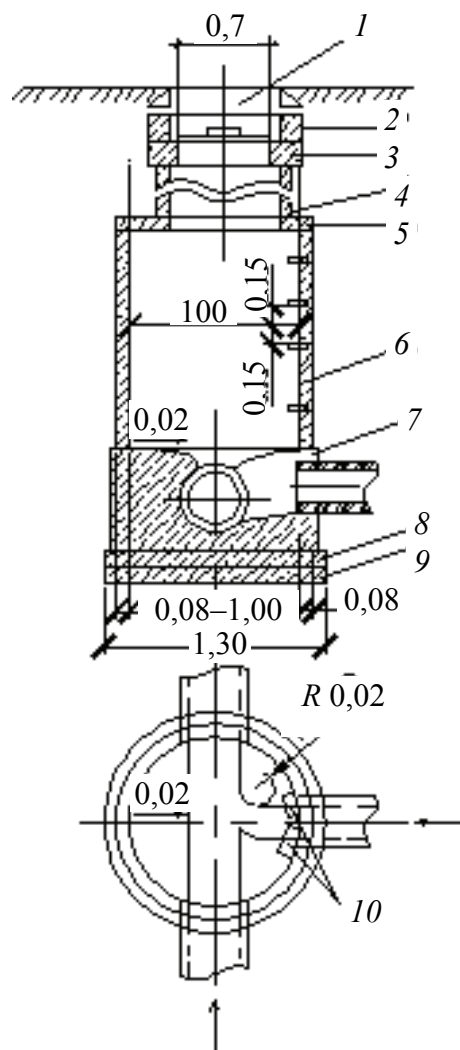
Рис. 3.1.3. Узловой колодец диаметром до 400 мм: 1 – чугунный люк с крышкой; 2, 3 – кольца регулировочное и опорное; 4, 6 – железобетонные кольца диаметром 700 и 1000 мм; 5 – плита перекрытия; 7 – регулировочные блоки; 8 – основание; 9 – подготовка; 10 – скобы
