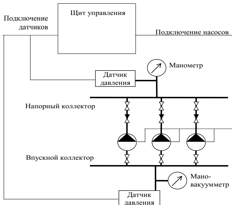
Рисунок 4.4 – Типовая структурная схема МАНС (на базе трех насосов)
