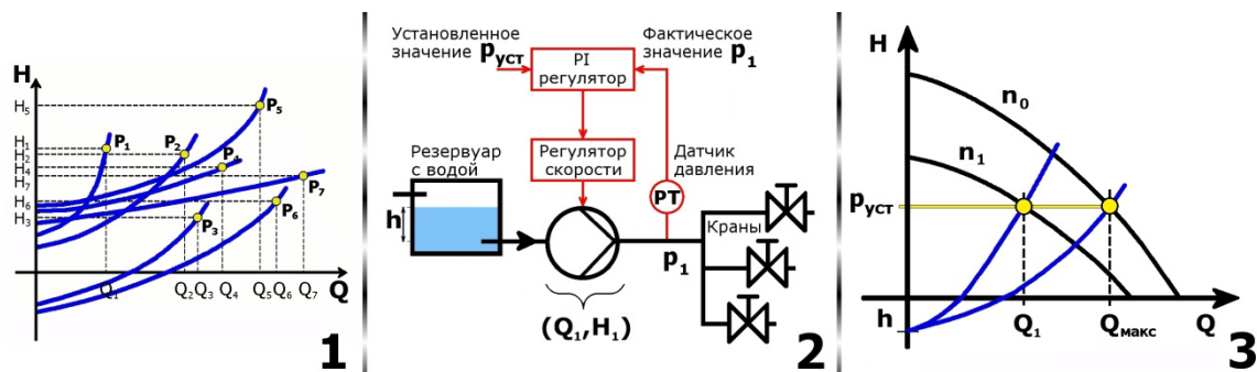
Рисунок В.4 – Регулирование скорости насоса по критерию постоянного давления
