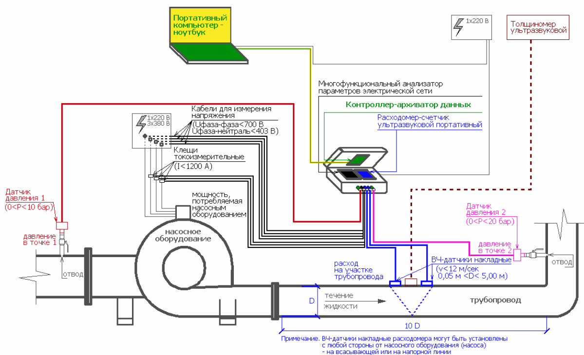
Рисунок Г.1 – Компоновка и принципиальная схема работы МИК
