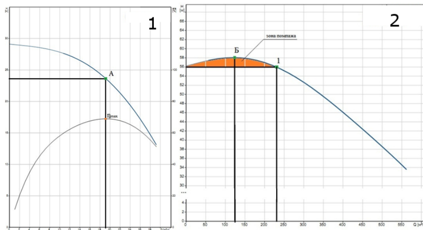
1 – стабильно нисходящая кривая; 2 – восходящая кривая
