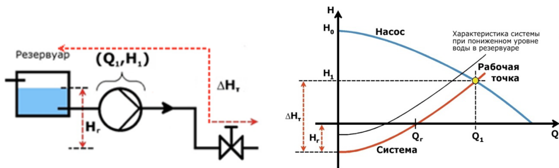
Рисунок Б.2 – Открытая система водоснабжения с насосом (ПНУ) выше точки разбора
