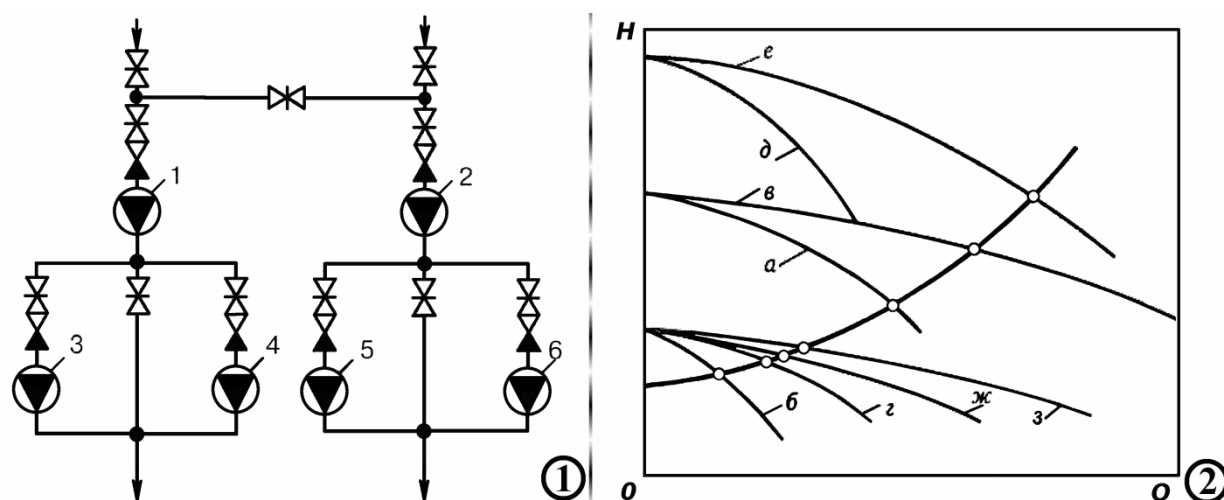
1 – схема соединения насосов; 2 – график совместной работы насосов и водовода
