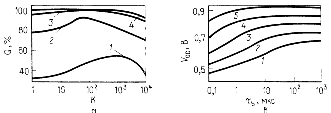
Рис. 8.3. Расчетные характеристики многопереходных кремниевых солнечных элементов с V-образными канавками, [16]. а) Зависимости внутреннего коэффициента собирания носителей заряда Q от коэффициента концентрации K солнечного излучения при различных значениях объемного времени жизни носителей: 1 — 0,1 мкс, 2 — 1 мкс, 3 — 10 мкс, 4 — 100 мкс; б) Зависимости напряжения холостого хода V_{oc} от объемного времени жизни носителей \tau_b при различных значениях коэффициента концентрации излучения: 1 — 1, 2 — 10, 3 — 10^2 , 4 — 10^3 , 5 — 10^4 ; в) Зависимости КПД от объемного времени жизни носителей \tau_b при различных значениях коэффициента концентрации излучения: 1 — 1, 2 — 10, 3 — 10^2 , 4 — 10^3 , 5 — 10^4 .
