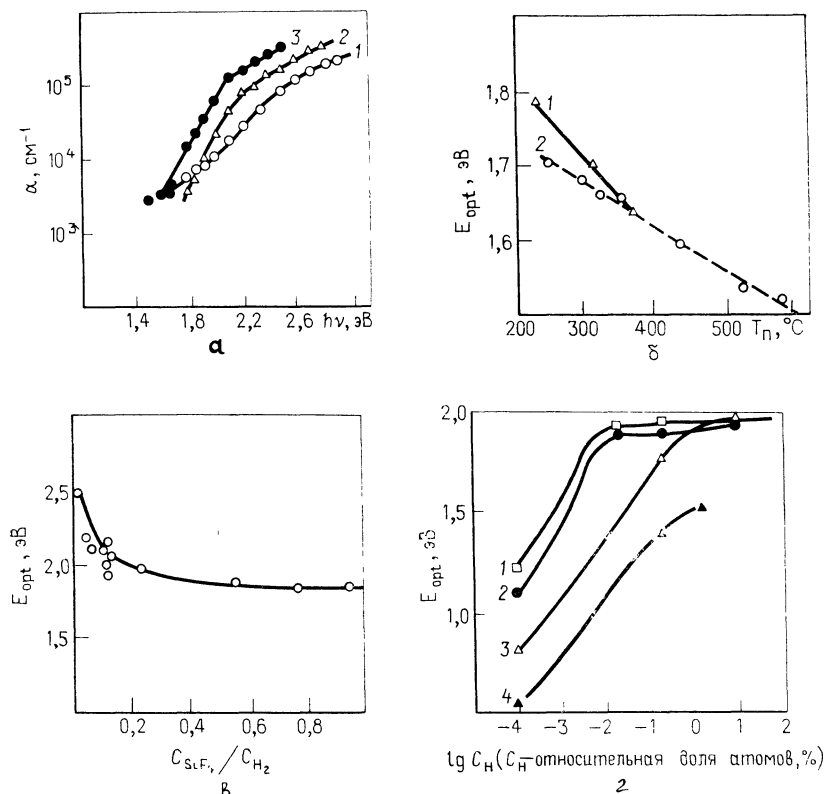
Рис. 6.3. а) Зависимости оптического коэффициента поглощения \alpha пленок а-Si : Н, осаждаемых в тлеющем разряде при различных температурах подложки T_p , от энергии фотонов h\nu [37]. 1 — T_p = 210 °C; 2 — T_p = 325 °C; 3 — T_p = 415 °C; б) Зависимости оптической ширины запрещенной зоны E_{opt} пленок а-Si : Н, осаждаемых в тлеющем разряде постоянного тока (1) и в высокочастотном разряде (2), от температуры подложки T_p [37]; в) Зависимость E_{opt} пленок а-Si : F : Н, осаждаемых в тлеющем разряде, от отношения концентраций газов SiF_4 и H_2 C_{SiF_4}/C_{H_2} в разрядной камере [6]; г) Зависимости E_{opt} пленок а-Si : Н, получаемых методом высокочастотного ионного распыления при различных давлениях p распыляющего газа, от концентрации атомов водорода C_H в плазме [24]. 1 — p = 10 Па; 2 — p = 5,3 Па; 3 — p = 2,7 Па; 4 — p = 0,7 Па.
