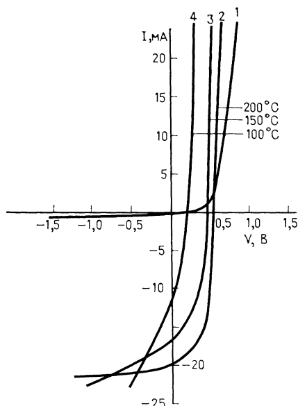
Рис. 4.11. Изменение формы вольт-амперных характеристик тонкопленочных солнечных элементов на основе \text{Cu}_2\text{S} — \text{CdS} в процессе термообработки. 1 — темновая характеристика, 2—4 — световые характеристики.
