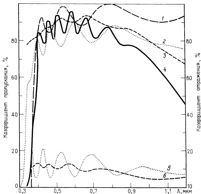
Рис. 3.31. Спектральные зависимости параметров различных прозрачных проводящих пленок. Коэффициент пропускания: 1 — ZnO [251], 2 — ITO [225], 3 — SnO 2 , легированный фтором [219], 4 — Cd 2 SnO 4 [252]. Коэффициент отражения: 5 — ITO [225], 6 — SnO 2 , легированный фтором [219].
