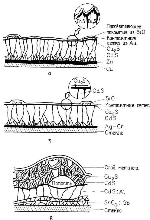
Рис. 4.4. Схематическое изображение микроstructures тонкопленочных солнечных элементов на основе \text{Cu}_2\text{S} — \text{CdS} , создаваемых методами испарения в сочетании с мокрым процессом (а), испарения в сочетании с сухим процессом (б) и пульверизации в сочетании с мокрым процессом (в).
