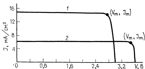
Рис. 8.11. Расчетные вольт-амперные характеристики сбалансированного (1) и несбалансированного (2) интегральных каскадных преобразователей, состоящих из трех элементов [30]. 1 — E_{g1}=1,10 эВ, E_{g2}=1,46 эВ, E_{g3}=1,97 эВ; 2 — E_{g1}=1,10 эВ, E_{g2}=1,55 эВ, E_{g3}=2,40 эВ; V_m и J_m — напряжение и плотность тока, соответствующие максимальной мощности.
