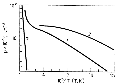
Рис. 3.6. Температурные зависимости концентрации p носителей в эпитаксиальном слое Si (1), осажденном методом ионного распыления [22], и в массивном образце Si (2). Кривая 3 соответствует собственной концентрации носителей.
