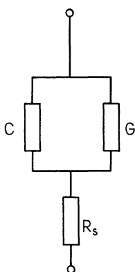
Рис. 1.5. Эквивалентная схема импеданса солнечного элемента.
