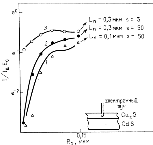
Рис. 1.14. Зависимости нормированного тока, наведенного электронным лучом, от средней глубины генерации носителей в слое \text{Cu}_x\text{S} солнечных элементов на основе \text{Cu}_x\text{S} — \text{CdS} , подвергнутых обработке в различных условиях [74]. Сплошные линии — теоретические зависимости при различных значениях диффузионной длины электронов L_n и нормированной скорости поверхностной рекомбинации s после получения пленки \text{Cu}_2\text{S} химическим методом (1), после термообработки на воздухе (2) и обработки в тлеющем разряде в атмосфере водорода с последующим старением (3).
