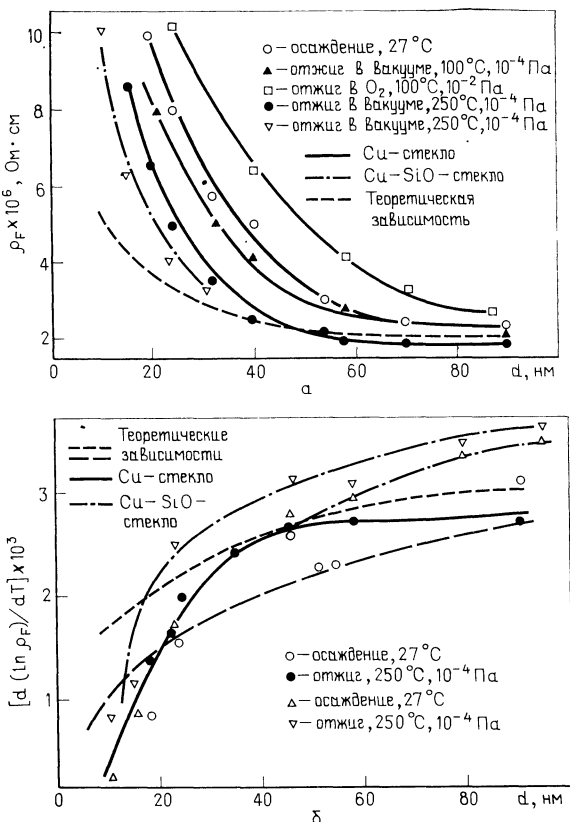
Рис. 3.35. а) Зависимости удельного сопротивления пленок меди (нанесенных на чистую поверхность стекла и на стеклянную подложку, покрытую слоем SiO) от их толщины d при различных параметрах процессов осаждения и отжига [259]; б) зависимости температурного коэффициента удельного сопротивления d(\ln \rho_F)/dT ( T , К) пленок меди (нанесенных на чистую поверхность стекла и на стеклянную подложку, покрытую слоем SiO) от их толщины непосредственно после осаждения и после отжига в вакууме [259].
