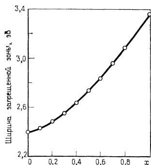
Рис. 3.20. г. Зависимость оптической ширины запрещенной зоны пленок \text{Zn}_x\text{Cd}_{1-x}\text{S} от параметра x [116].
