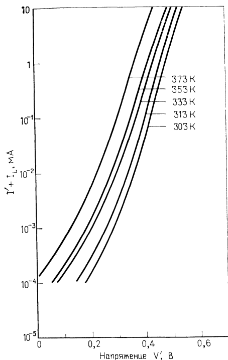
Рис. 1.1. Зависимости I' + I_L от V' для солнечных элементов на основе \text{Cu}_2\text{S} — \text{CdS} при различной температуре.
