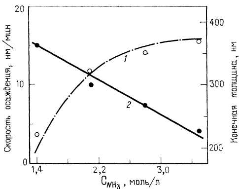
Рис. 2.13. Кривые зависимостей конечной толщины (1) и скорости осаждения из раствора (2) пленок CdSe от концентрации комплексобразующего агента [95].
