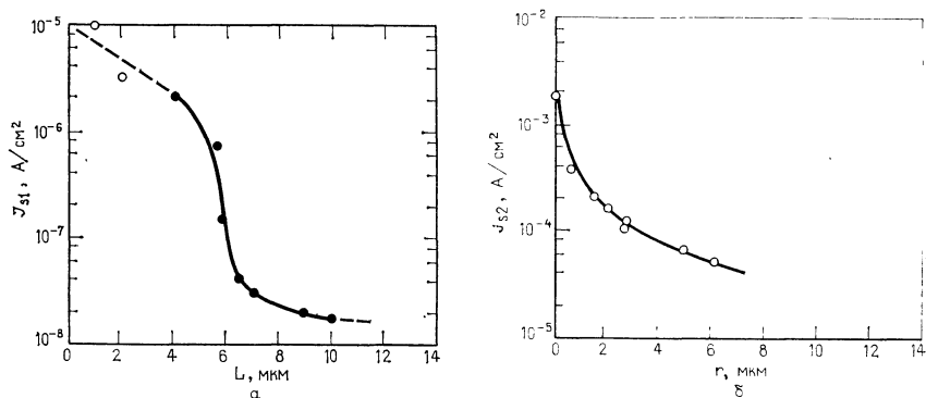
Рис. 5.1. Влияние диффузионной длины носителей заряда и размера зерен в пленке кремния на диффузионную J_{s1} и рекомбинационно-генерационную J_{s2} составляющие плотности обратного тока насыщения в солнечных элементах, изготовленных методом вакуумного испарения [23]. а) зависимость J_{s1} от диффузионной длины L носителей; б) зависимость J_{s2} от размера зерен r (предел разрешения метода поверхностной фото-э. д. с. — 4 \mu\text{м} ).
