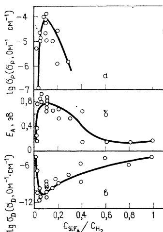
Рис. 6.5. Зависимости удельной фотопроводимости \sigma_p в условиях АМ1 (а), энергии активации E_A (б) и темновой удельной проводимости \sigma_D (в) пленок а-Si : F : H, осаждаемых в тлеющем разряде, от отношения концентраций \text{SiF}_4 и \text{H}_2 [6].
