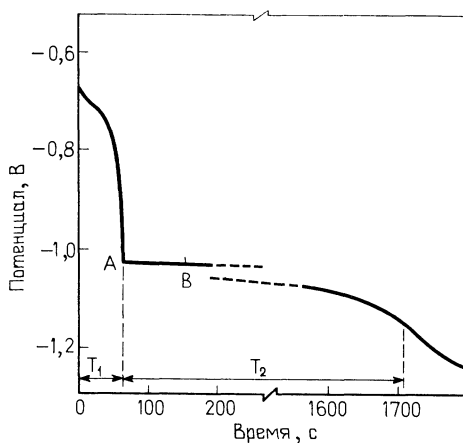
Рис. 1.11. Зависимости потенциала от времени, измеряемые при электрохимическом анализе \text{Cu}_x\text{S} [57].
