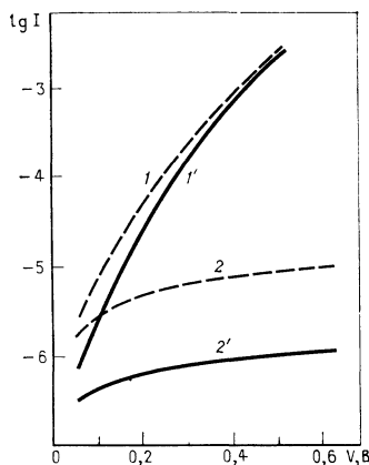
Рис. 5.3. Темновые вольт-амперные характеристики поликристаллических кремниевых солнечных элементов с n-p -переходом непосредственно после изготовления (1, 2) и после обработки в водородной плазме (1', 2') в течение 16 ч при температуре 350 °С и давлении \sim 270 Па [30]. Ток I измеряется в А, напряжение V — в В.
