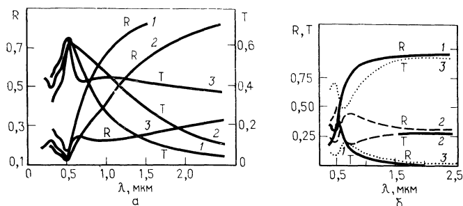
Рис. 3.38. Спектральные зависимости коэффициентов отражения R и пропускания T пленок золота [262]; а) пленки толщиной 12 нм имеют разную кристаллическую структуру (1, 2, 3); б) толщина пленок: 1 — 27,5 нм, 2 — 15,0 нм, 3 — 5,6 нм.
