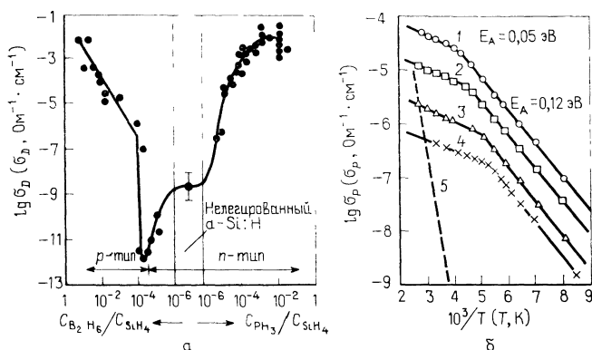
Рис. 6.4. а) Зависимость темновой удельной проводимости \sigma_D (при комнатной температуре) легированных пленок a-Si:H, осаждаемых в тлеющем разряде, от отношения концентраций газов \text{B}_2\text{H}_6 и \text{SiH}_4 , а также \text{PH}_3 и \text{SiH}_4 [43]; в нелегированном a-Si:H проводимость зависит от параметров энергетических уровней в запрещенной зоне, связанных с дефектами структуры; б) Температурные зависимости удельной фотопроводимости \sigma_p нелегированных пленок a-Si:H при различных плотностях потока фотонов: 1 — 2 \cdot 10^{15} \text{ см}^{-2} \cdot \text{с}^{-1} ; 2 — 2 \cdot 10^{14} \text{ см}^{-2} \cdot \text{с}^{-1} ; 3 — 2 \cdot 10^{13} \text{ см}^{-2} \cdot \text{с}^{-1} ; 4 — 2 \cdot 10^{12} \text{ см}^{-2} \cdot \text{с}^{-1} [37]; длина волны света — 0,61 мкм; около кривых указаны значения энергии активации E_A , соответствующие различным механизмам рекомбинации; кривая 5 — температурная зависимость темновой удельной проводимости эталонных образцов.
