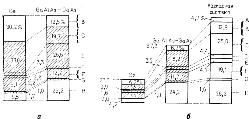
Рис. 8.9. Распределение потерь энергии в единичных солнечных элементах на основе Ge и GaAlAs—GaAs (а) и в двухэлементном каскадном преобразователе, состоящем из элементов на основе Ge и GaAlAs—GaAs (б), при 125-кратной интенсивности излучения в условиях AM2 [24]. А — потери в фильтре, В — отражение излучения и затенение поверхности, С — избыточная энергия фотонов, D — энергия нефотоактивных фотонов, Е — потери при собирании носителей заряда, F — потери в области перехода, G — омические потери ( IR^2 ), H — выходная мощность; заштрихованные области соответствуют потерям энергии, вызывающим нагрев элементов.
