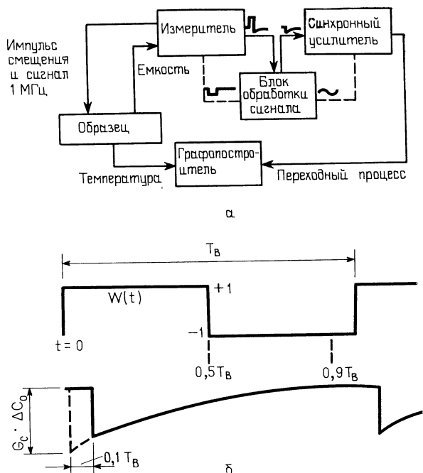
Рис. 1.7. Блок-схема установки для измерений по методу емкостной спектроскопии глубоких уровней (а) и схематическое изображение весовой функции и сигнала на входе синхронного усилителя (б) [26].
