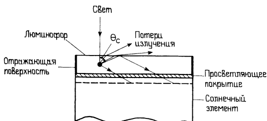
Рис. 8.4. Схематическое изображение структуры люминофор — солнечный элемент.
