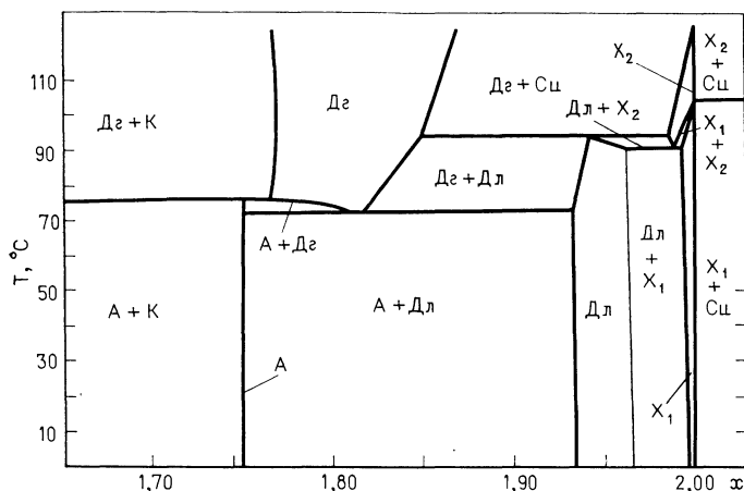
Рис. 3.21. Фазовая диаграмма системы \text{Cu-S} в области составов \text{Cu}_x\text{S} , при емлемых для создания солнечных элементов со структурой \text{Cu}_x\text{S-CdS} Дг — дигенит, К — ковеллит, Дл — дюрлит, X_1 — низкотемпературный халькоцит, X_2 — высокотемпературный халькоцит, А — анилит.
