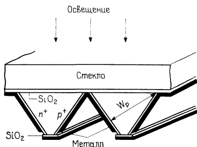
Рис. 8.2. Схема конструкции многопереходного солнечного элемента с V-образными канавками [16].
