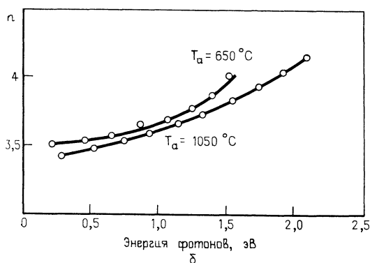
Рис. 3.7. Зависимости оптического коэффициента поглощения (а) и показателя преломления n (б) аморфных и поликристаллических пленок Si, полученных химическим осаждением из паровой фазы, от энергии фотонов [6]. 1 — аморфный Si, температура отжига T_a = 650^\circ\text{C} ; 2 — поликристаллический Si, T_a = 1050^\circ\text{C} ; 3 — монокристаллический Si.
