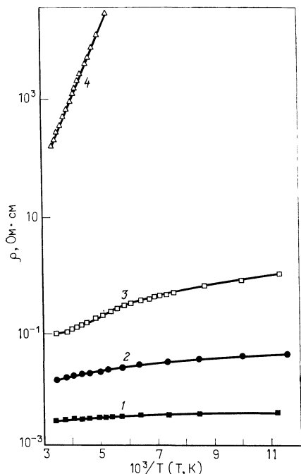
Рис. 3.26. Температурные зависимости удельного сопротивления \rho пленок \text{Cu}_x\text{S} различной толщины, полученных методом вакуумного испарения [185]. 1 — 0,17 мкм, 2 — 0,25 мкм, 3 — 0,36 мкм, 4 — 0,45 мкм.
