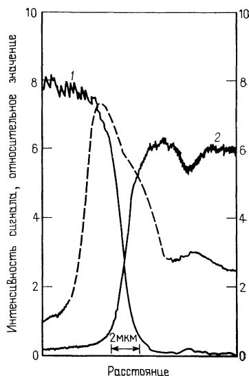
Рис. 7.2. Профили распределения концентрации теллура (1) и серы (2) в тонкопленочном солнечном элементе на основе \text{Cu}_x\text{Te} - \text{CdTe} - \text{CdS} после термообработки в оптимальном режиме, определенные методом рентгеновского микроанализа (масштаб кривой 2 по оси ординат уменьшен в 3 раза); штриховая линия — кривая распределения тока, наведенного электронным лучом, по толщине элемента [26].
