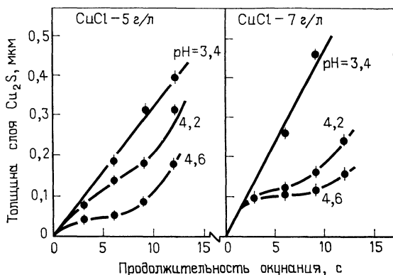
Рис. 2.20. Влияние различных параметров на процесс осаждения пленок \text{Cu}_2\text{S} , получаемых посредством окунания [137].
