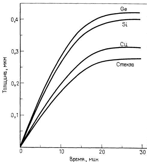
Рис. 2.15. Влияние материала подложки на процесс осаждения из раствора пленок PbSe [43] при температуре ванны 28 °C и pH = 10,4 .
