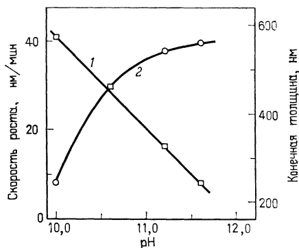
Рис. 2.14. Влияние pH на скорость роста (кривая 1) и конечную толщину (кривая 2) пленок PbSe, осаждаемых из раствора [43] при температуре ванны 60 °С.
