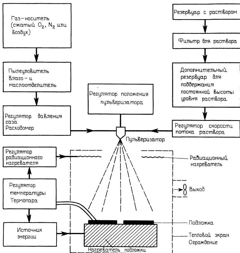
Рис. 2.3. Блок-схема установки, применяемой в лаборатории авторов для осаждения тонких пленок CdS методом пульверизации с последующим пиролизом.
