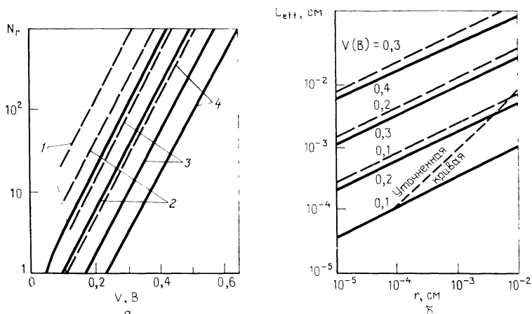
Рис. 5.5. Теоретические зависимости относительного количества N_r границ зерен, содержащих активные рекомбинационные центры, от напряжения смещения V , приложенного к элементу с барьером Шоттки, при различных размерах зерен: 10^{-5} см (1), 10^{-4} см (2), 10^{-3} см (3) и 10^{-2} см (4) (а); зависимости эффективной диффузионной длины L_{\text{eff}} неосновных носителей заряда от размера зерен r при различных напряжениях смещения V (б) [37]; сплошные линии соответствуют высоте потенциального барьера на границах зерен \Phi_g = 0,5 В, штриховые линии — \Phi_g = 0,6 В.
