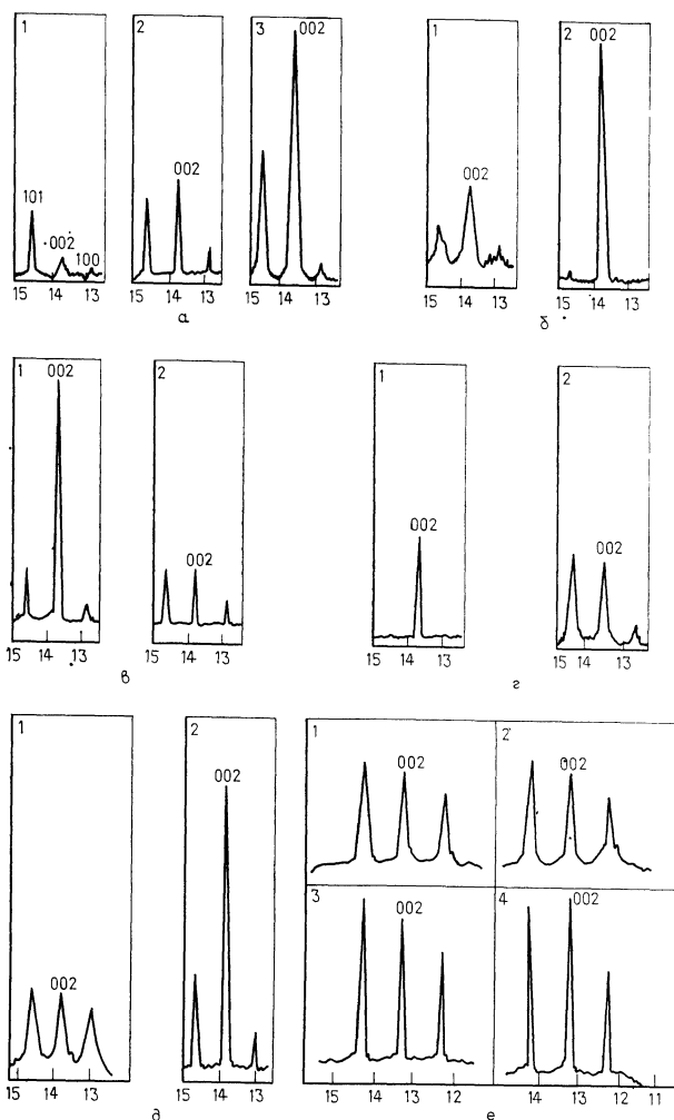
Рис. 3.14. Влияние отношения концентраций атомов Cd и S (а), температуры подложки (б), толщины пленки (в), легирующей примеси (г), наличия на подложке других слоев (д) и отжига, проводимого после осаждения (е) на степень ориентации пленки.
