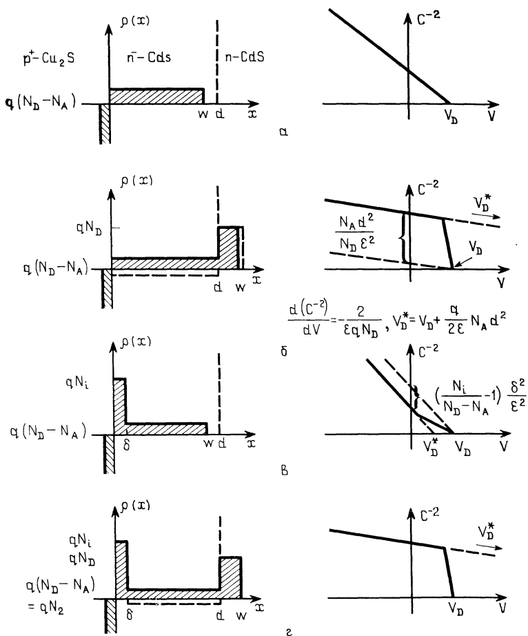
Рис. 1.6. Возможные профили распределения пространственного заряда и соответствующие зависимости C^{-2} от V .
