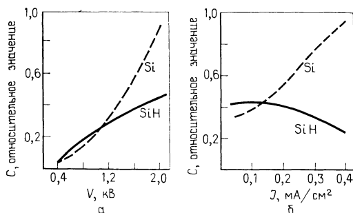
Рис. 6.2. Зависимости концентрации C кремния Si и моногидрида кремния SiH от напряжения V на электродах в системе для высокочастотного ионного распыления (а) и от плотности тока J тлеющего разряда в системе для плазменного осаждения (б) [23]. а) состав газа — \text{Ar} + \text{H}_2 (10 %), давление — 1 Па; б) состав газа — \text{Ar} + \text{SiH}_4 (1 %), давление — 3,6 Па.
