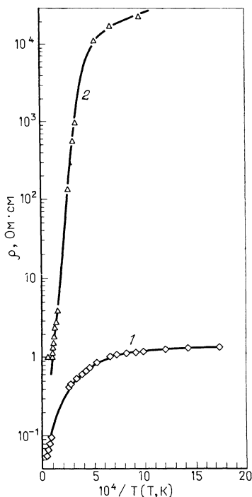
Рис. 3.23. Температурные зависимости удельного сопротивления \rho массивных образцов \text{Cu}_2\text{S} [180]. 1 — нелегированный \text{Cu}_2\text{S} , 2 — \text{Cu}_2\text{S} , легированный кадмием.
