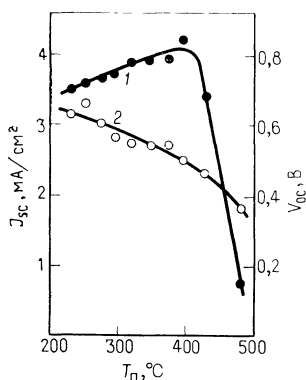
Рис. 6.11. Зависимости плотности тока короткого замыкания J_{sc} (1) и напряжения холостого хода V_{oc} (2) солнечного элемента с барьером Шоттки на основе а-Si:H и Pt от температуры подложки T_n при осаждении пленки а-Si:H [37].
