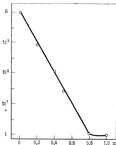
Рис. 3.20 б. Зависимость отношения G фотопроводимости к темновой проводимости от параметра x пленок \text{Zn}_x\text{Cd}_{1-x}\text{S} , получаемых методом пульверизации с последующим пиролизом [139].
