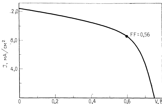
Рис. 6.10. Вольт-амперная характеристика солнечного элемента на основе а-Si : F : H со структурой металл — диэлектрик — полупроводник [14]; площадь элемента — 4,2 мм²; интенсивность излучения — 83 мВт/см².
