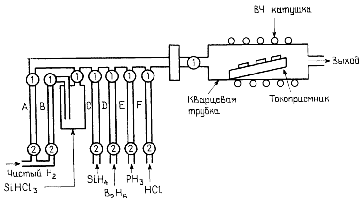
Рис. 2.18. Блок-схема системы для химического осаждения из паровой фазы, применяемая для изготовления тонкопленочных кремниевых солнечных элементов [115].
