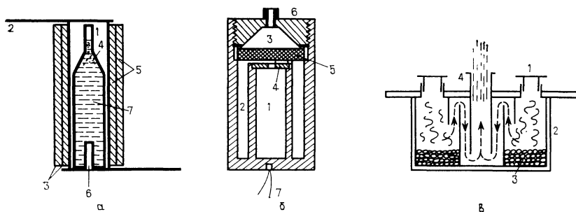
Рис. 2.1. Схемы устройства различных испарителей;
