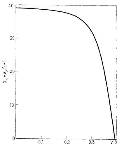
Рис. 7.5. Вольт-амперная характеристика тонкопленочного солнечного элемента на основе p\text{-CuInSe}_2 — n\text{-CdS} с переменным уровнем легирования, измеренная в условиях AM1 при интенсивности излучения 101,5 \text{ мВт/см}^2 [54].
