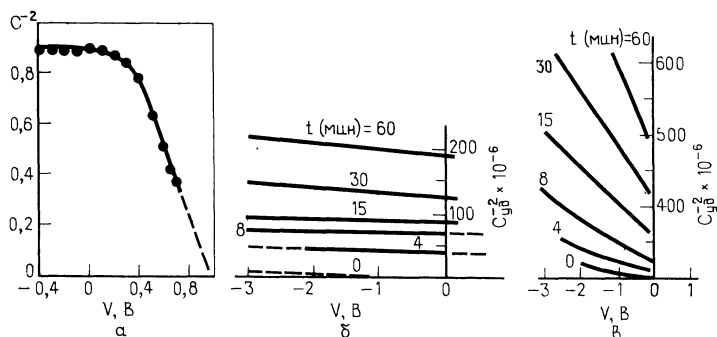
Рис. 4.9. Зависимость C^{-2} солнечного элемента на основе \text{Cu}_2\text{S} — \text{CdS} , изготовленного методом пульверизации, от напряжения смещения V (емкость C измерена в нФ) (а) [74]; кривые зависимости C_{\text{уд}}^{-2} солнечных элементов со структурой \text{Cu}_2\text{S} — \text{CdS} , полученных методом вакуумного испарения, с не травленным (б) и травленным (в) слоями \text{CdS} , от напряжения смещения V при различной продолжительности t термообработки (удельная емкость C_{\text{уд}} измерена в \text{Ф/м}^2 ) [76].
