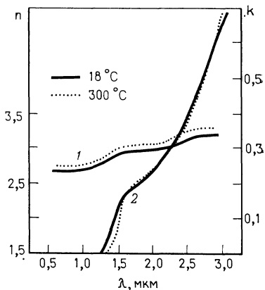
Рис. 3.11. Спектральные зависимости показателей преломления n (1) и поглощения k (2) пленок CdTe, полученных методом вакуумного испарения при двух различных температурах подложки [64].
