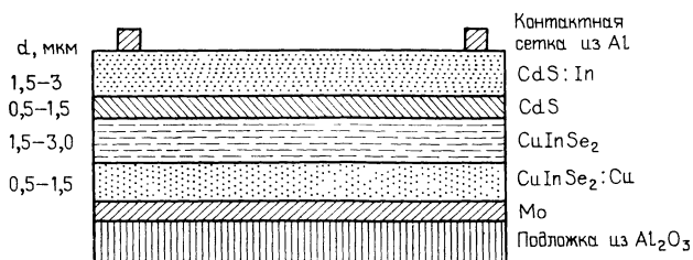
Рис. 7.4. Схема конструкции высокоэффективного тонкопленочного солнечного элемента на основе p\text{-CuInSe}_2 — n\text{-CdS} с переменным уровнем легирования [54].
