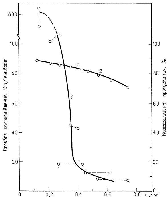
Рис. 3.32. Зависимости слоевого сопротивления (1) и коэффициента пропускания (2) легированных фтором пленок \text{SnO}_x , полученных методом пульверизации с последующим пиролизом, от их толщины d .
