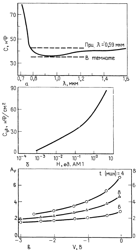
Рис. 4.10. Спектральная зависимость емкости C тонкопленочного солнечного элемента на основе \text{Cu}_2\text{S}-\text{CdS} (а), зависимость его удельной емкости C_{уд} от интенсивности излучения H (б) [65, 79] и кривые зависимости коэффициента увеличения A_F площади перехода от обратного напряжения смещения V при различной продолжительности термообработки ( t ) [76].
