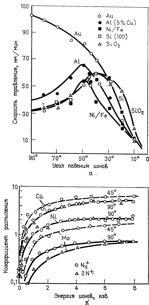
Рис. 2.2. Зависимости скорости ионного травления различных материалов от угла падения ионов (а) и зависимости коэффициента распыления материалов от энергии ионов двух видов, имеющих разный угол падения (б).
