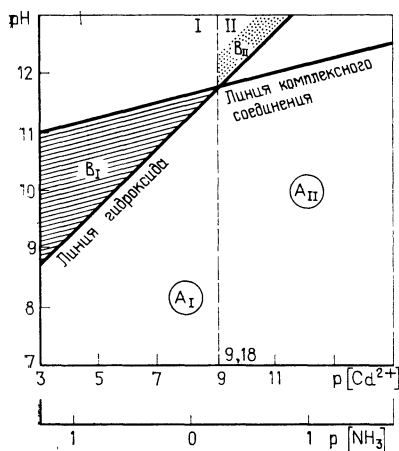
Рис. 2.9. Графики зависимости pH от p[\text{Cd}^{2+}] и p[\text{NH}_3] [91].
