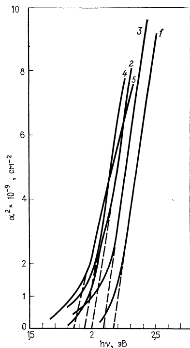
Рис. 3.27. Зависимости квадрата коэффициента поглощения \alpha пленок \text{Cu}_x\text{S} , полученных методом вакуумного испарения, от энергии фотонов h\nu [185] для пленок различной толщины (обозначения кривых см. в подписи рис. 3.25).
