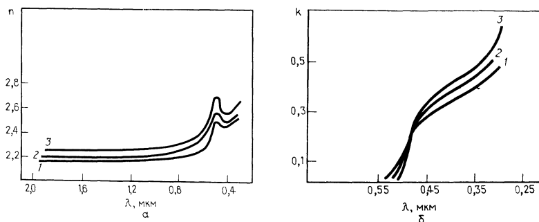
Рис. 3.18. Спектральные зависимости показателей преломления n (а) и поглощения k (б) пленок CdS, полученных вакуумным испарением при трех различных температурах подложки [124]. 1 — комнатная температура; 2 — 140 °C; 3 — 180 °C.
