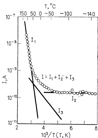
Рис. 3.40. Температурная зависимость тока, проходящего через диод со структурой \text{Au}-\text{Si}_3\text{N}_4-\text{Si} при напряженности электрического поля 5,3 \cdot 10^6 В/см [261]. I_1 — ток, обусловленный эмиссией Пула—Френкеля, I_2 — туннельный ток, I_3 — омический ток.
