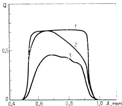
Рис. 7.3. Кривые зависимостей коэффициента сбора Q носителей заряда в тонкопленочных солнечных элементах на основе InP — CdS от длины волны света \lambda .
