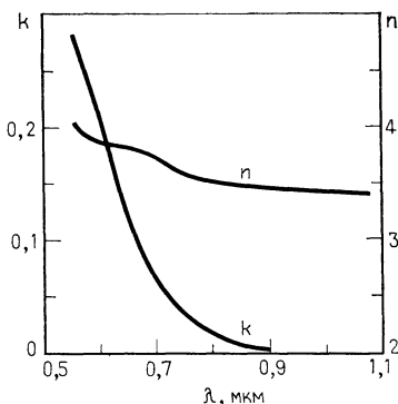
Рис. 3.13. Спектральные зависимости оптических постоянных n и k пленок \text{Zn}_3\text{P}_2 [83].
