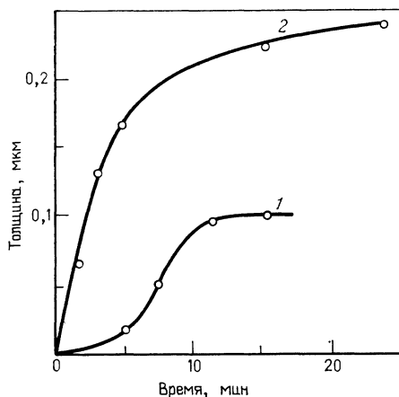
Рис. 2.10. Типичный характер роста пленок, осаждаемых из раствора [43]. 1 — неактивированная подложка, 2 — активированная подложка.
