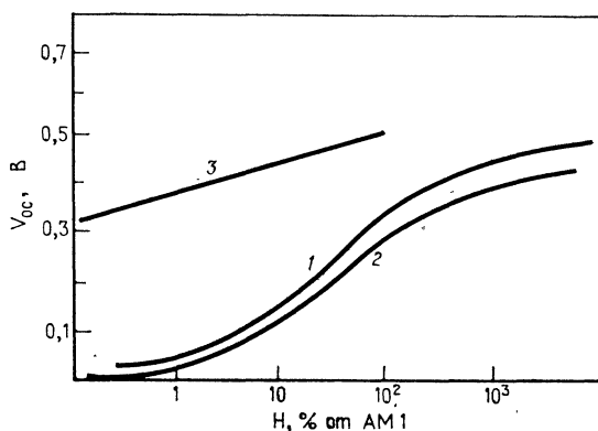
Рис. 4.7. Кривые зависимостей напряжения холостого хода V_{oc} от интенсивности излучения H для солнечных элементов на основе \text{Cu}_2\text{S} — \text{Zn}_{0.1}\text{Cd}_{0.9}\text{S} (1) и \text{Cu}_2\text{S} — \text{CdS} (2), получаемых методом пульверизации, и типичных элементов со структурой \text{Cu}_2\text{S} — \text{CdS} , создаваемых с помощью вакуумного испарения (3) [28].
