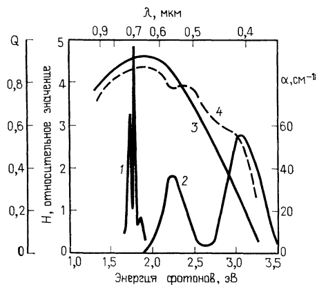
Рис. 8.5. Спектральные зависимости интенсивности люминесценции H (1) и коэффициента поглощения \alpha (2) рубина (массовое содержание Сг 0,7 %), а также коэффициента сбора носителей Q в кремниевом солнечном элементе с n — p -структурой при отсутствии (3) и наличии (4) покрытия из рубина [17].
