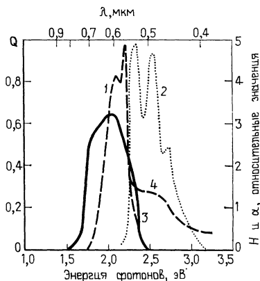
Рис. 8.6. Спектральные зависимости интенсивности люминесценции H (1) и коэффициента поглощения \alpha (2) рубена, а также коэффициента сбора носителей Q в тыльно-барьерном солнечном элементе на основе \text{Cu}_2\text{S} - \text{CdS} при отсутствии (3) и наличии (4) люминесцентного покрытия, активированного рубеном [17].
