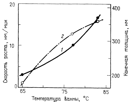
Рис. 2.16. Влияние температуры ванны на скорость роста (кривая 1) и конечную толщину (кривая 2) пленок CdSe, осаждаемых из раствора [49].
