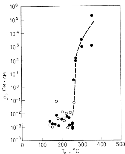
Рис. 3.29. Зависимость удельного сопротивления \rho пленок \text{CuInSe}_2 , получаемых методом вакуумного испарения, от температуры подложки T_n при избыточной концентрации Se в испаряемом веществе, равной 20 % [193].
