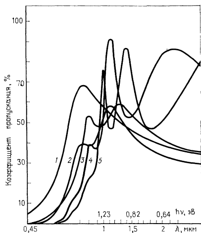
Рис. 3.25. Спектральные зависимости коэффициента пропускания пленок \text{Cu}_x\text{S} различной толщины, полученных методом вакуумного испарения [185]. 1 — 0,13 мкм, 2 — 0,25 мкм, 3 — 0,33 мкм, 4 — 0,45 мкм, 5 — 0,6 мкм.
