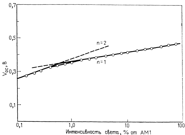
Рис. 1.3. Зависимость V_{oc} солнечного элемента на основе Cu_2S — CdS от интенсивности излучения.
