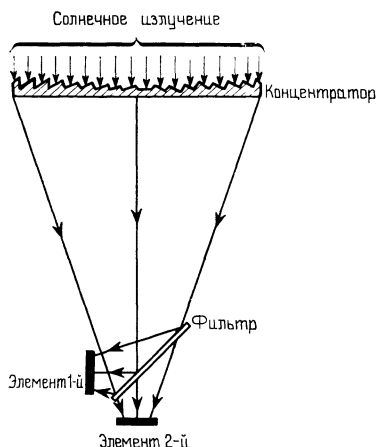
Рис. 8.7. Схема каскадного солнечного элемента на основе оптического фильтра, концентратора излучения и двух элементов.
