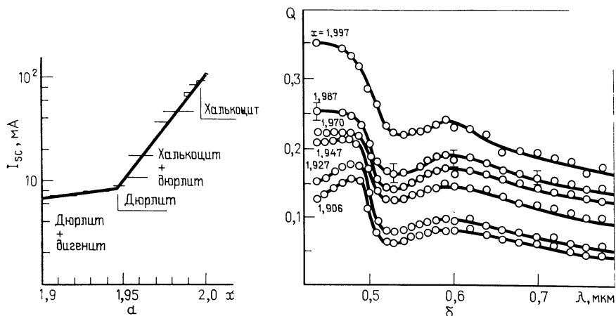
Рис. 4.12. Влияние состава слоя \text{Cu}_x\text{S} на ток короткого замыкания I_{sc} (а) [89] и коэффициент собирания Q носителей (б) [92] в солнечных элементах со структурой \text{Cu}_x\text{S} — \text{CdS} .
