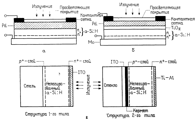
Рис. 6.8. Схемы конструкций солнечных элементов на основе а-Si:H. а — структура с барьером Шоттки; б — структура металл — диэлектрик — полупроводник; в — p-i-n-структура.
