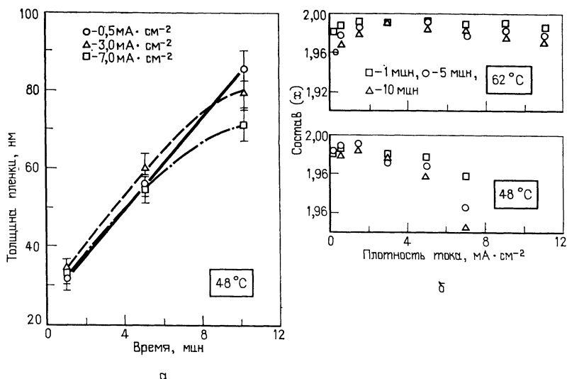
Рис. 2.21. Особенности процесса роста (а) и зависимость состава пленок \text{Cu}_2\text{S} , получаемых методом электроосаждения, от температуры и плотности тока при различной продолжительности процесса (б) [151].
