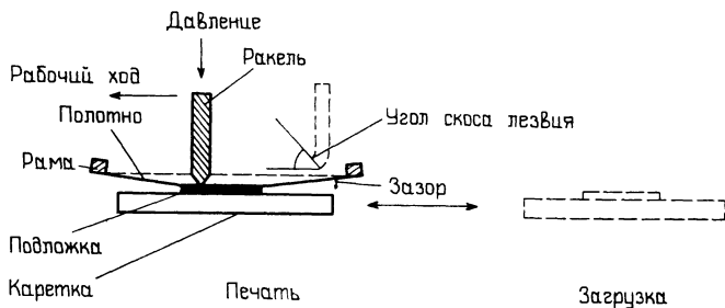
Рис. 2.17. Схема устройства для трафаретной печати.
