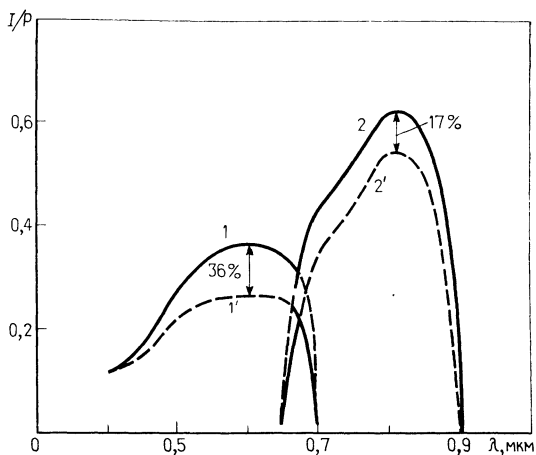
Рис. 8.13. Спектральные зависимости чувствительности — отношения генерируемого тока I (А) к мощности падающего излучения P (Вт) — интегрального каскадного солнечного элемента со структурой GaAlAs—GaAs [34]. Кривые 1 и 2 характеризуют чувствительность единичных элементов, изготовленных соответственно из GaAlAs и GaAs при наличии просветляющего покрытия, состоящего из пленок \text{Ta}_2\text{O}_5 толщиной 56 нм и \text{SiO}_2 толщиной 120 нм; кривые 1' и 2' — аналогичные зависимости до нанесения просветляющего покрытия.
