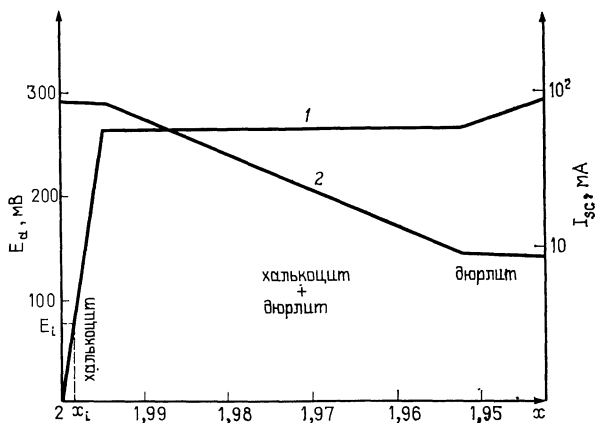
Рис. 3.22. Зависимость потенциала E_d разложения \text{Cu}_x\text{S} (1) и тока короткого замыкания I_{sc} (2) солнечных элементов со структурой \text{Cu}_x\text{S—CdS} от параметра x [179].
