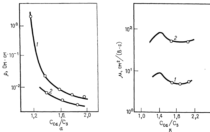
Рис. 3.15. Зависимости удельного сопротивления \rho (а) и подвижности \mu (б) носителей в пленках CdS, полученных вакуумным испарением и легированных индием, от отношения концентраций атомов Cd и S в потоке пара [107]—1 — концентрация In — 1 %; 2 — концентрация In — 1,5 %.
