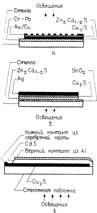
Рис. 4.1. Схемы конструкций тонкопленочных солнечных элементов на основе \text{Cu}_2\text{S} - \text{CdS} : а — фронтально-барьерная, б — тыльно-барьерная, в — с обратным расположением слоев.
