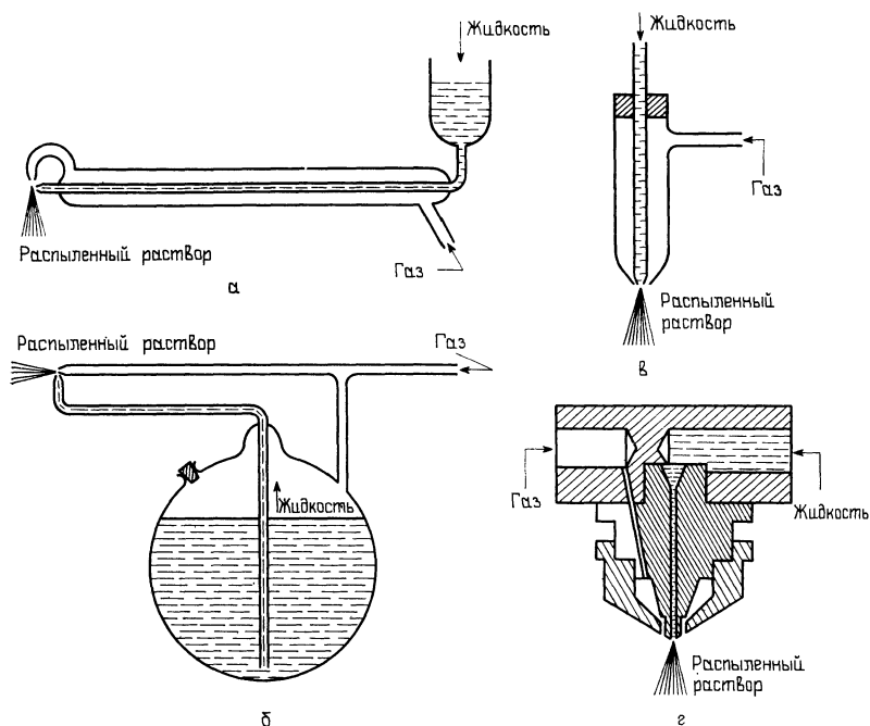
Рис. 2.4. Схемы обычно применяемых пульверизаторов (а, б, в) и поперечное сечение пульверизатора, выпускаемого Spraying System Co., США (г).
