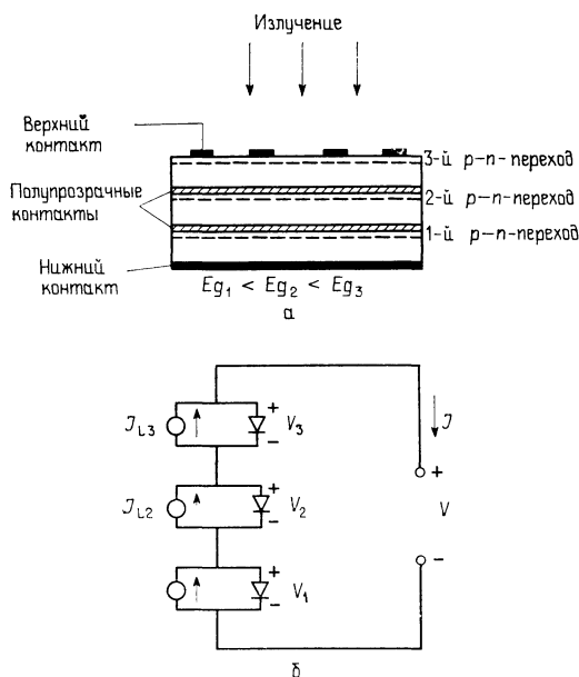
Рис. 8.10. Поперечное сечение интегрального каскадного солнечного элемента, содержащего три гомогенных перехода (а), и его эквивалентная схема (б).
