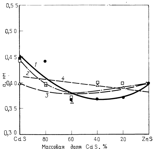
Рис. 3.20 а. Зависимость параметра a гексагональной кристаллической решетки пленок \text{Zn}_x\text{Cd}_{1-x}\text{S} от их состава при температуре осаждения 200 °C (1), 170 °C (2) и 90 °C (3) [111]; аналогичная зависимость для массивного образца, рассчитанная с помощью закона Вигарда (4).
