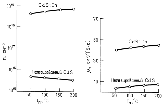
Рис. 3.16. Зависимости концентрации n и подвижности \mu носителей от температуры подложки T_p для нелегированных и легированных индием пленок CdS, полученных дискретным испарением [110].
