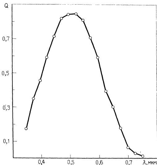
Рис. 6.9. Спектральная зависимость коэффициента сбора Q носителей заряда в солнечном элементе на основе a\text{-Si:H} с p-i-n -структурой 1-го типа [39].
