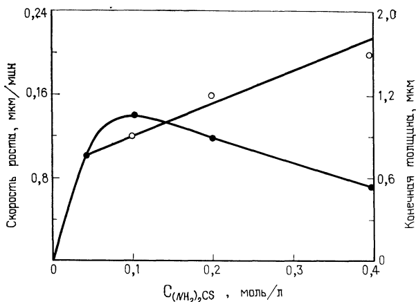
Рис. 2.12. Кривые зависимостей скорости роста (1) и конечной толщины (2) пленок CdS, осаждаемых из раствора, от концентрации ионов серы в исходном соединении [91].
