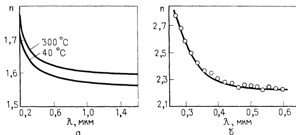
Рис. 3.39. Спектральные зависимости показателей преломления пленок \text{Al}_2\text{O}_3 , осажденных методом вакуумного испарения на подложки с температурой 40 и 300 °C (а), и анодной пленки \text{Ta}_2\text{O}_5 (б) [254].
