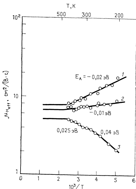
Рис. 3.5. Температурные зависимости эффективной холловской подвижности носителей \mu_{H,eff} в пленках Si, осажденных методом вакуумного испарения, при различных концентрациях легирующей примеси [17]: 1 — 1,1 \cdot 10^{19} \text{ см}^{-3} ; 2 — 1,8 \cdot 10^{19} \text{ см}^{-3} ; 3 — 3,6 \cdot 10^{19} \text{ см}^{-3} ; около кривых указаны значения энергии активации E_A .
