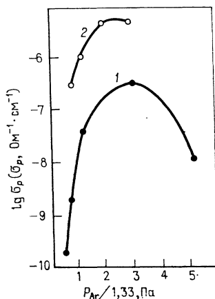
Рис. 6.6. Зависимости удельной фотопроводимости \sigma_p (при комнатной температуре) пленок а-Si : H, получаемых методом ионного распыления, от парциального давления аргона p_{\text{Ar}} при парциальном давлении водорода, равном 0,03 Па (1) и 0,08 Па (2) [22]; энергия фотонов—1,96 эВ; плотность потока фотонов— 10^{15} \text{ см}^{-2} \cdot \text{с}^{-1} .
