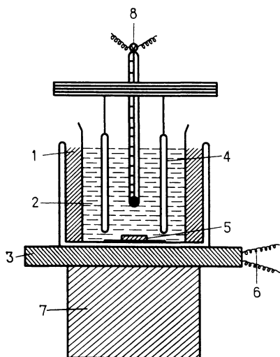
Рис. 2.8. Экспериментальная установка, применяемая в лаборатории авторов для выращивания полупроводниковых пленок из раствора.
