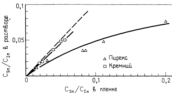
Рис. 2.7. Зависимости отношения концентраций атомов олова и индия C_{Sn}/C_{In} в пленках ИТО от состава распыляемого раствора при использовании различных подложек [47].
