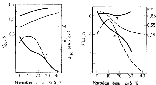
Рис. 4.14. Зависимости напряжения холостого хода V_{oc} (1), плотности тока короткого замыкания J_{sc} (2), коэффициента заполнения вольт-амперной характеристики FF (3) и КПД (4) от содержания сульфида цинка ZnS в слое Zn_xCd_{1-x}S тонкопленочных солнечных элементов на основе Cu_2S-Zn_xCd_{1-x}S , изготовленных методами вакуумного испарения (сплошные линии) и пульверизации с последующим пиролизом (штриховые линии) [19].
