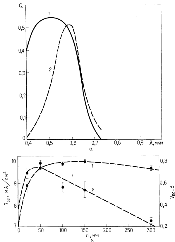
Рис. 6.12. а) Спектральные зависимости коэффициента собирания Q носителей заряда в солнечных элементах на основе a-Si : H с p-i-n -структурой при толщине верхнего легированного слоя p -типа, равной 10 нм (1) и 36 нм (2) [122]; б) Зависимости плотности тока короткого замыкания J_{sc} (2) и напряжения холостого хода V_{oc} (1) солнечного элемента на основе a-Si : H с p-i-n -структурой от толщины d n -слоя [39]; элемент освещен со стороны n -слоя.
