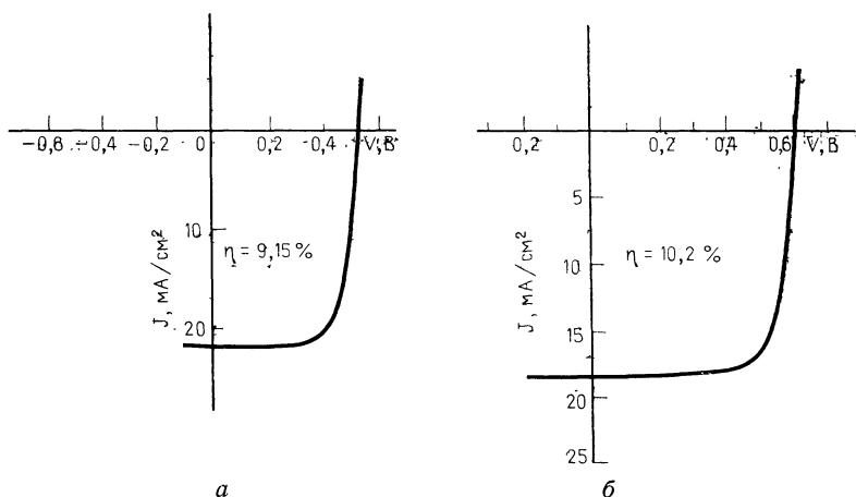
Рис. 4.5. Вольт-амперные характеристики высокоэффективных тонкопленочных солнечных элементов на основе \text{Cu}_2\text{S}-\text{CdS} (а) и \text{Cu}_2\text{S}-\text{Zn}_{0,16}\text{Cd}_{0,84}\text{S} (б), изготовленных методом испарения в сочетании с мокрым химическим процессом [6, 7]; а — площадь элемента A = 0,84 \text{ cm}^2 , интенсивность излучения H = 87,9 \text{ мВт/см}^2 ; б — A = 0,98 \text{ cm}^2 , H = 81,2 \text{ мВт/см}^2 .
