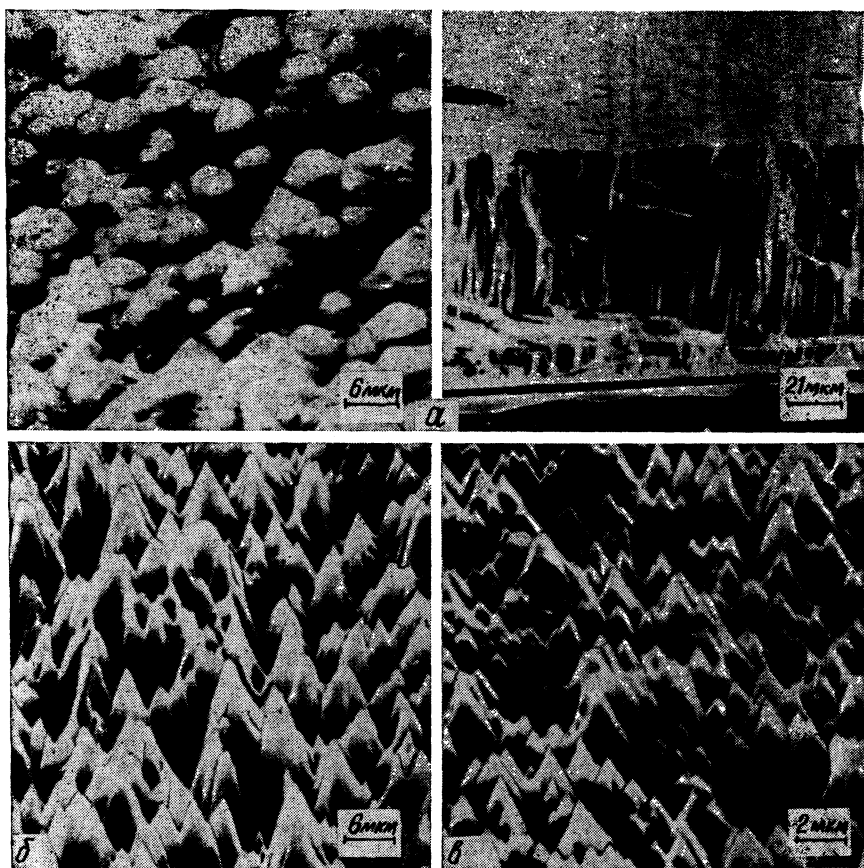
Рис. 4.2. Микроснимки, полученные с помощью растрового электронного микроскопа: а — поверхностный рельеф и структура поперечного сечения пленки CdS, нанесенной методом вакуумного испарения, непосредственно после ее осаждения; б — поверхность CdS после травления; в — поверхностный рельеф пленки \text{Cu}_2\text{S} , выращенной на травленной поверхности CdS.
