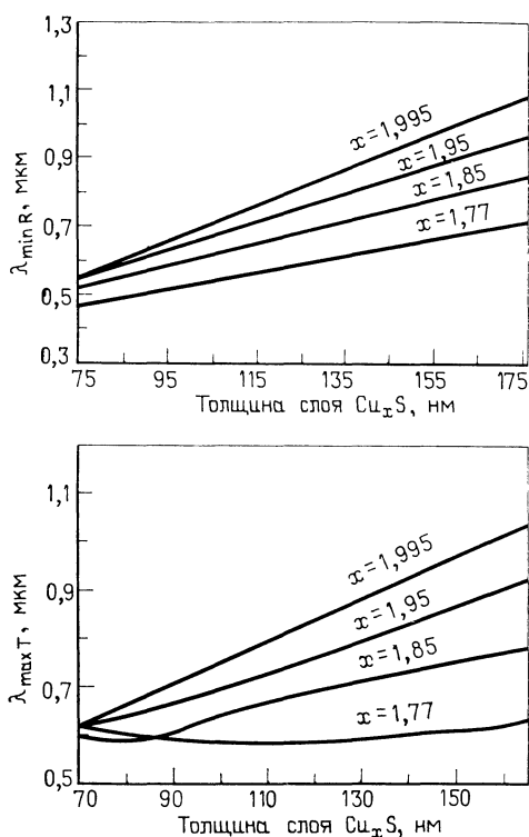
Рис. 1.12. Положение главных минимумов коэффициента отражения ( \lambda_{\min R} ) и максимумов коэффициента пропускания ( \lambda_{\max T} ) в зависимости от толщины пленок \text{Cu}_x\text{S} при различных значениях x [61].
