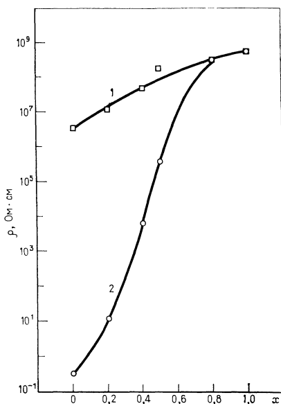
Рис. 3.20. в. Зависимость удельного сопротивления \rho пленок \text{Zn}_x\text{Cd}_{1-x}\text{S} , получаемых методом пульверизации с последующим пиролизом, от параметра x [139]. 1 — непосредственно после осаждения, 2 — после отжига.
