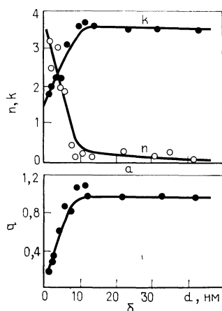
Рис. 3.37. Зависимости оптических постоянных n и k при длине волны 0,59 мкм (а) и коэффициента заполнения q (б) пленок серебра от их толщины d [254].
