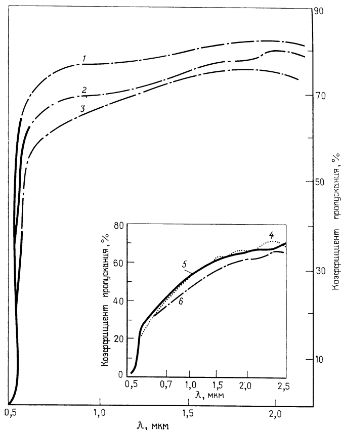
Рис. 3.19. Спектральные зависимости коэффициента пропускания пленок CdS, осажденных методом пульверизации с последующим пиролизом при различных условиях [134, 141]. 1 — T_p = 365^\circ\text{C} , d = 3,5 мкм; 2 — T_p = 380^\circ\text{C} , d = 5,7 мкм; 3 — T_p = 260^\circ\text{C} , d = 3,3 мкм; 4 — Cd : S = 1 : 1,4, T_p = 317^\circ\text{C} ; 5 — Cd : S = 1 : 1,2, T_p = 317^\circ\text{C} ; 6 — Cd : S = 1 : 1, T_p = 317^\circ\text{C} .
