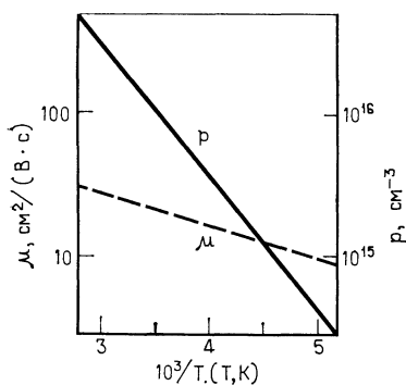
Рис. 3.12. Температурные зависимости подвижности \mu и концентрации p носителей в пленках InP, осажденных методом вакуумного испарения [80].
