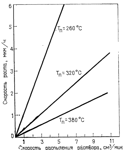
Рис. 2.5. Зависимости скорости роста пленки CdS, осаждаемой методом пульверизации с последующим пиролизом, от скорости распыления раствора и температуры подложки ( T_p ) [39].
