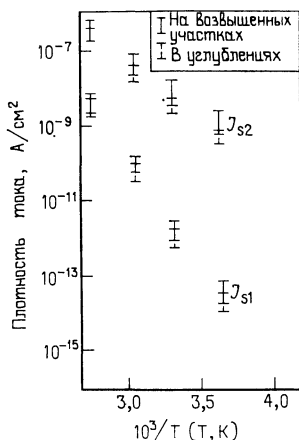
Рис. 5.4. Температурные зависимости диффузионной J_{s1} и рекомбинационно-генерационной J_{s2} составляющих плотности обратного тока насыщения диодов, изготовленных на возвышенных участках пленки кремния и в углублениях поверхности [16].
