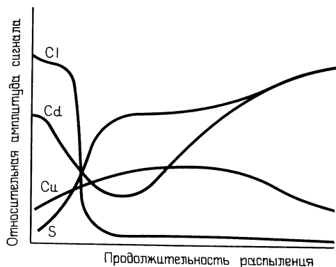
Рис. 1.10. Полученные методом оже-спектроскопии профили распределения химических элементов в тонкопленочных солнечных элементах на основе \text{Cu}_2\text{S} - \text{CdS} непосредственно после реакции в твердой фазе.
