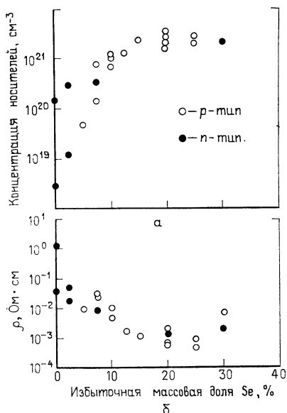
Рис. 3.28. Зависимости концентрации носителей (а) и удельного сопротивления \rho (б) пленок \text{CuInSe}_2 , полученных вакуумным испарением при температуре подложки 250^\circ\text{C} , от избыточного содержания селена в испаряемом веществе [193] для пленок n - и p -типов.
