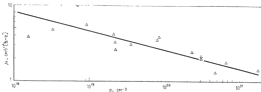
Рис. 3.24. Зависимость подвижности дырок \mu от их концентрации p в массивных образцах \text{Cu}_x\text{S} [180].
