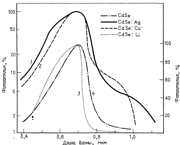
Рис. 3.9. Спектральные зависимости фоточувствительности нелегированных и легированных пленок CdSe, осажденных из раствора [46]. Кривые 1, 2 — левая шкала, кривые 3, 4 — правая шкала.
