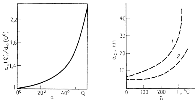
Рис. 3.36. а) Зависимость нормированной критической толщины пленок Ag, осаждаемых методом вакуумного испарения на стеклянные подложки при температуре 25^\circ\text{C} со скоростью \sim 0,1 нм/с, от угла падения Q на подложку пучка пара [254]; б) зависимости критической толщины пленок от температуры подложки при отсутствии электрического поля (1) и при наличии поля напряженностью 100 В/см (2).
