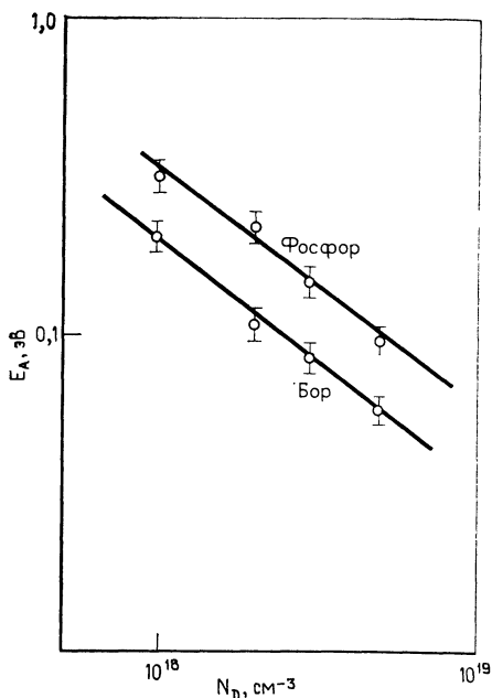
Рис. 3.3. Зависимости энергии активации E_A от концентрации N_D легирующей примеси в поликристаллических пленках Si, полученных химическим осаждением из паровой фазы [8].
