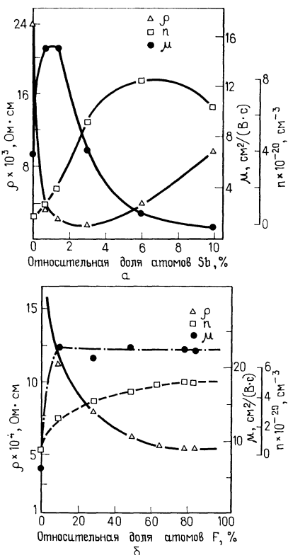
Рис. 3.30. Зависимости удельного сопротивления \rho , подвижности \mu и концентрации n носителей от содержания примеси в пленках \text{SnO}_x , легированных Sb (a) и F (б) [219, 220].
