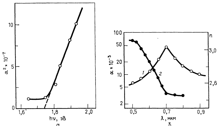
Рис. 3.10. Зависимость квадрата коэффициента поглощения \alpha^2 от энергии фотонов h\nu (а) и зависимости показателя преломления n (1) и \alpha (2) от длины волны света \lambda (б) для пленок CdSe, осажденных из раствора [46]. Величина \alpha измеряется в \text{см}^{-1} .
