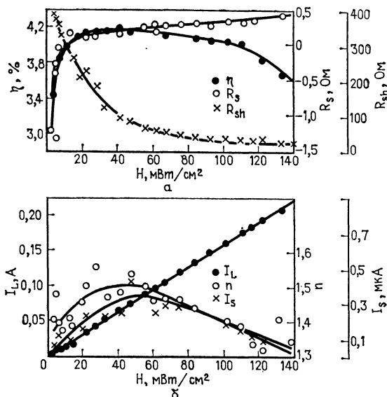
Рис. 4.6. Зависимости КПД, последовательного R_s и шунтирующего R_{sh} сопротивлений (а), а также фототока I_L , диодного коэффициента n и обратного тока насыщения I_s (б) солнечного элемента на основе \text{Cu}_2\text{S} — \text{CdS} от интенсивности излучения H [61].
