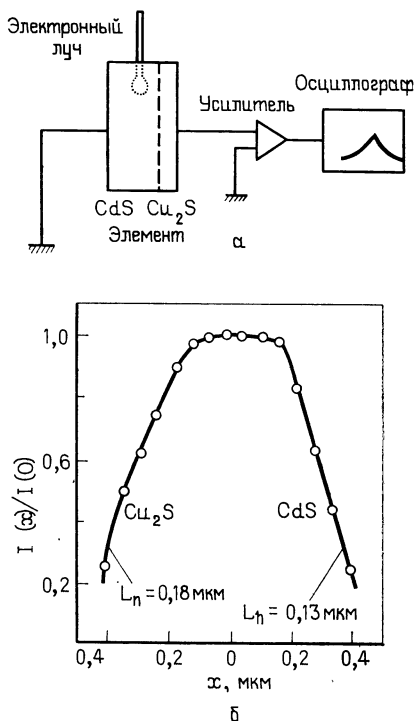
Рис. 1.13. Схема экспериментальной установки для измерения диффузионной длины неосновных носителей заряда по методу наведения тока электронным лучом (а) и зависимость I(x)/I(0) от расстояния до перехода в тонкопленочном солнечном элементе на основе \text{Cu}_2\text{S} — \text{CdS} (б).
