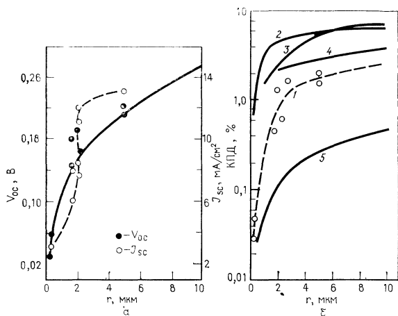
Рис. 5.2. а) Зависимости напряжения холостого хода V_{oc} и плотности тока короткого замыкания J_{sc} солнечных элементов, изготовленных методом вакуумного испарения, от размера зерен r в пленке кремния; сплошная линия — теоретическая зависимость V_{oc} от r ; б) Зависимости КПД солнечных элементов от размера зерен r в пленке кремния; 1 — экспериментальные данные [23], 2—5 — результаты расчета различных авторов: 2 — [32], 3 — [34], 4 — [31], 5 — [33].
