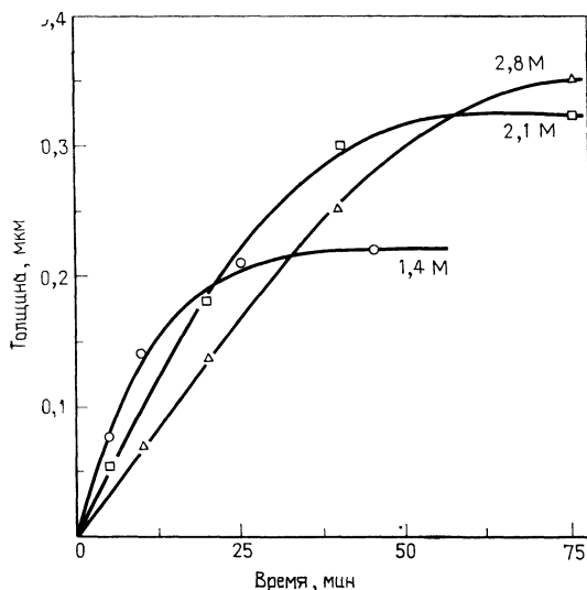
Рис. 2.11. Зависимости толщины пленки CdSe, осаждаемой на активированную подложку, от продолжительности процесса осаждения при различных концентрациях \text{NH}_3 [95].
