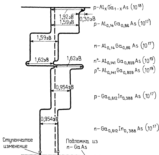
Рис. 8.12. Энергетическая зонная диаграмма идеализированного двухпереходного интегрального каскадного солнечного элемента на основе \text{AlGaAs} — \text{GaInAs} , оптимизированного для работы в условиях АМ0 [32]; около химических формул в скобках указаны значения концентрации носителей заряда ( \text{см}^{-3} ).
