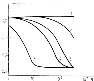
Рис. 8.1. Расчетные зависимости коэффициента заполнения FF вольт-амперной характеристики кремниевых элементов от коэффициента концентрации K солнечного излучения при различных значениях последовательного сопротивления [4]. 1 — 0 Ом, 2 — 0,01 Ом, 3 — 0,05 Ом, 4 — 0,1 Ом, 5 — 1,0 Ом; диодный коэффициент n=1,5 , плотность темнового тока насыщения J_s = 3,3 \times 10^{-12} А/см 2 , T = 300 К, площадь элемента — 1 см 2 ; фототок пропорционален коэффициенту концентрации излучения.
