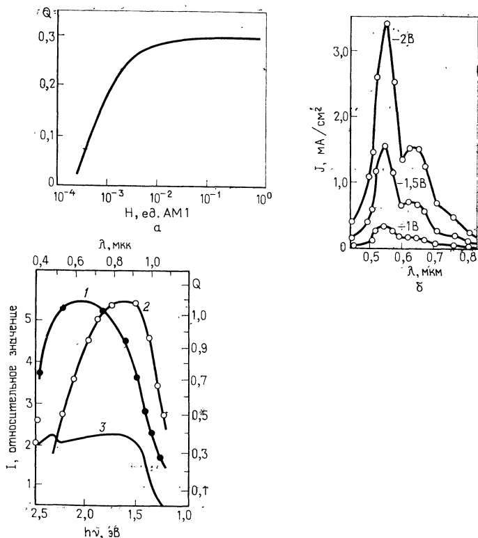
Рис. 4.8. Зависимость коэффициента собирания Q носителей при \lambda = 0,9 \text{ мкм} в тонкопленочных солнечных элементах на основе \text{Cu}_2\text{S}-\text{CdS} от интенсивности H белого света, используемого в качестве подсветки (а) [65]; спектральные зависимости плотности тока J солнечных элементов со структурой \text{Cu}_2\text{S}-\text{CdS} , получаемых методом пульверизации, при различных напряжениях смещения (б) [56]; зависимости тока I тыльно-барьерных солнечных элементов на основе \text{Cu}_2\text{S}-\text{CdS} от энергии фотонов h\nu при толщине слоя \text{CdS} 0,4 (1) и 13 \text{ мкм} (2), а также зависимости коэффициента собирания Q носителей во фронтально-барьерном элементе со структурой \text{Cu}_2\text{S}-\text{CdS} (3) от длины волны света \lambda (б). [65]
