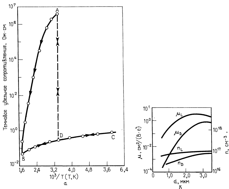
Рис. 3.17. Температурные зависимости темнового удельного сопротивления пленок CdS, осажденных методом пульверизации с последующим пиролизом, при отжиге в вакууме и в атмосфере различных газов [136] (а). Точка А определяет удельное сопротивление пленок непосредственно после осаждения, кривая АВ — изменение удельного сопротивления пленок в процессе отжига в вакууме, кривая ВС — удельное сопротивление пленок, отожженных в вакууме или атмосфере инертных газов, измеренное при различных температурах, точка D — измеренное при комнатной температуре удельное сопротивление пленок, отожженных в вакууме.
