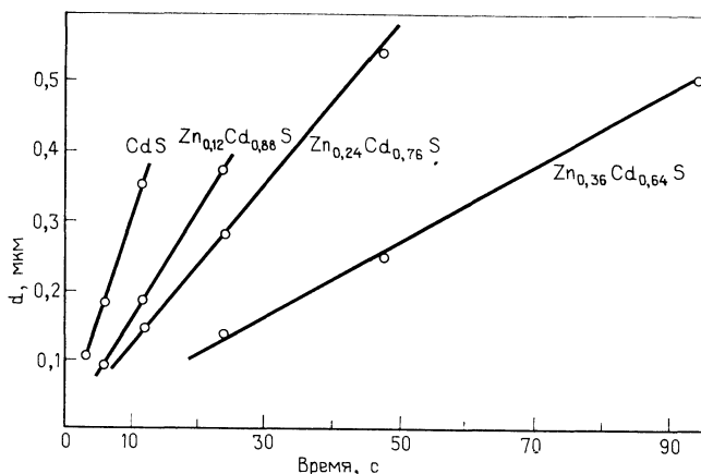
Рис. 4.13. Графики зависимости толщины слоя сульфида меди d от продолжительности окунания при различных составах пленок Zn_xCd_{1-x}S [79].
