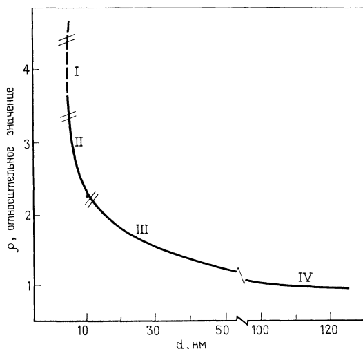
Рис. 3.33. Типичная зависимость удельного сопротивления \rho при 300 К пленки Au, нанесенной на стеклянную подложку, от ее толщины d . Области I—IV характеризуются различными механизмами проводимости.
