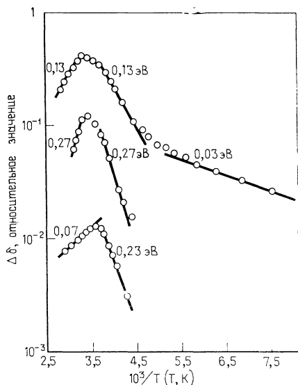
Рис. 3.2. Температурные зависимости фотопроводимости \Delta\delta (измеренные при энергии фотонов h\nu = 2,14 \text{ эВ} ) отожженных поликристаллических пленок Si, полученных химическим осаждением из паровой фазы при различных температурах подложки [6]: 1—680 °C; 2—600 °C; 3—700 °C; температура отжига 1050 °C; около кривых указаны значения энергии активации E_A .
