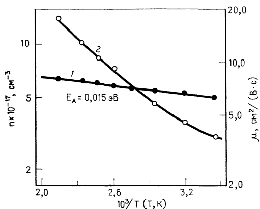
Рис. 3.8. Температурные зависимости концентрации n (1) и подвижности \mu (носителя \gamma в отожженных пленках CdSe, осажденных из раствора [46]).
