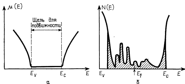
Рис. 6.1. Зависимости подвижности \mu(E) носителей заряда (а) и плотности состояний N(E) (б) от энергии E в аморфных полупроводниках. E_f — уровень Ферми, E_c и E_v — пороги подвижности, соответствующие дну зоны проводимости и вершине валентной зоны в кристаллических полупроводниках
