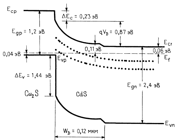
Рис. 4.15. Энергетическая зонная диаграмма солнечного элемента с гетеро-переходом \text{Cu}_2\text{S} — \text{CdS} ; E_{cp} , E_{gp} и E_{vp} — соответственно дно зоны проводимости, ширина запрещенной зоны и вершина валентной зоны в \text{Cu}_2\text{S} ; E_{cn} , E_{gn} и E_{vn} — аналогичные параметры \text{CdS} ; E_f — уровень Ферми, V_D — диффузионный потенциал, W_D — ширина обедненного слоя, \Delta E_c = E_{cp} - E_{cn} , \Delta E_v = E_{vp} - E_{vn} .
