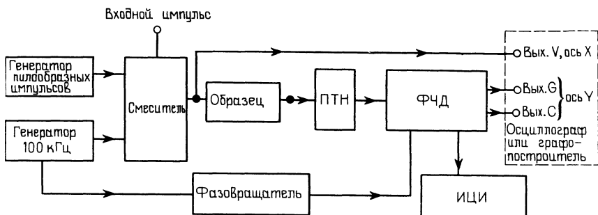
Рис. 1.4. Блок-схема автоматического измерителя вольт-фарадных характеристик.
