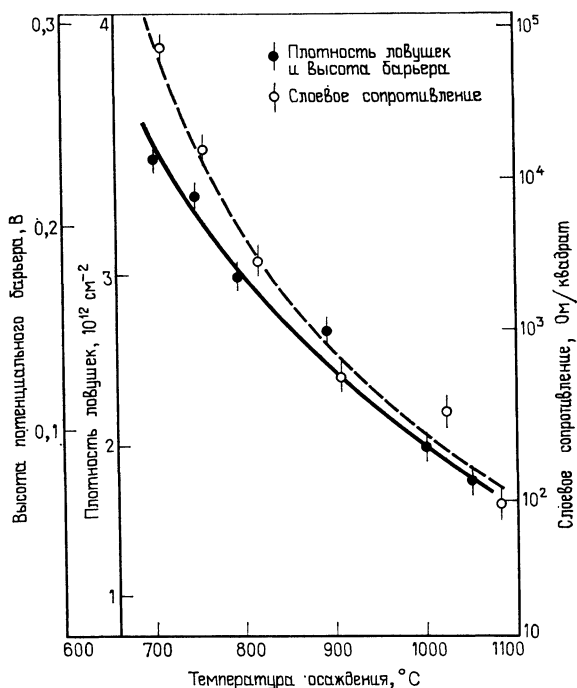
Рис. 3.4. Зависимости высоты потенциального барьера, плотности ловушек и слоевого сопротивления от температуры осаждения имплантированных бором поликристаллических пленок Si, полученных химическим методом из паровой фазы [8].
