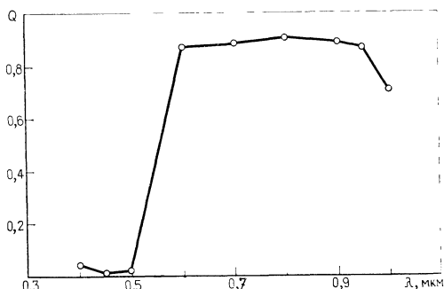
Рис. 7.6. Кривая спектральной зависимости коэффициента собирания Q носителей заряда в тонкопленочном солнечном элементе на основе \text{CuInSe}_2\text{—CdS} [54].
