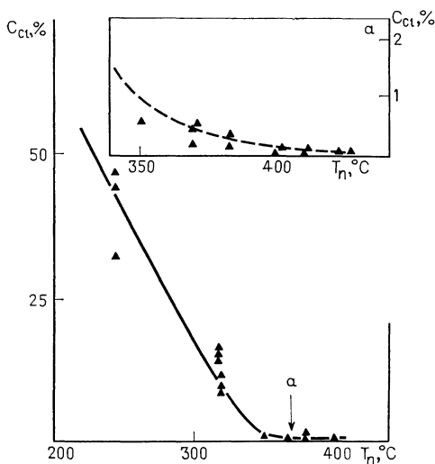
Рис. 2.6. Зависимость концентрации хлора C_{Cl} в пленках CdS, осаждаемых методом пульверизации с последующим пиролизом, от температуры подложки T_n [34].
