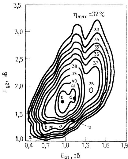
Рис. 8.8. Уровни равных значений предельного КПД ( \eta_{\max} ) каскадных систем на основе двух элементов, оптического фильтра и концентратора при 100-кратной интенсивности излучения в условиях АМ2 [24]. В системах используются солнечные элементы на основе следующих полупроводниковых материалов: а) Si и Ge ( \eta_{\max} = 34\% ); б) GaAs и Ge ( \eta_{\max} = 37\% ); в) GaAs и Si ( \eta_{\max} = 35\% ); д) Материал с E_{g2} = 1,75 эВ и Si ( \eta_{\max} = 41\% ); е) Материалы с оптимальными значениями ширины запрещенной зоны ( \eta_{\max} = 42\% ).
