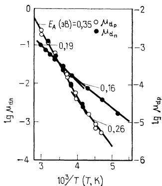
Рис. 6.7. Температурные зависимости дрейфовой подвижности основных носителей заряда — электронов ( \mu_{dn} ) и дырок ( \mu_{dp} ) — в пленках \text{a-Si:H} [34]. Подвижность измеряется в \text{см}^2/(\text{В} \cdot \text{с}) .
