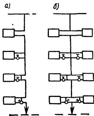
Рис. IV.25. Схемы вертикальных однетрубных стояков при верхней разводке подающей магистрали с односторонним а и двухсторонним б присоединением отопительных приборов
