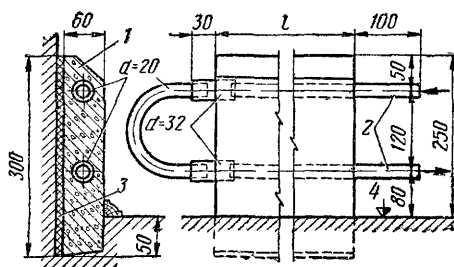
Рис. VIII.6. Плитусная приставная бетонная отопительная панель
