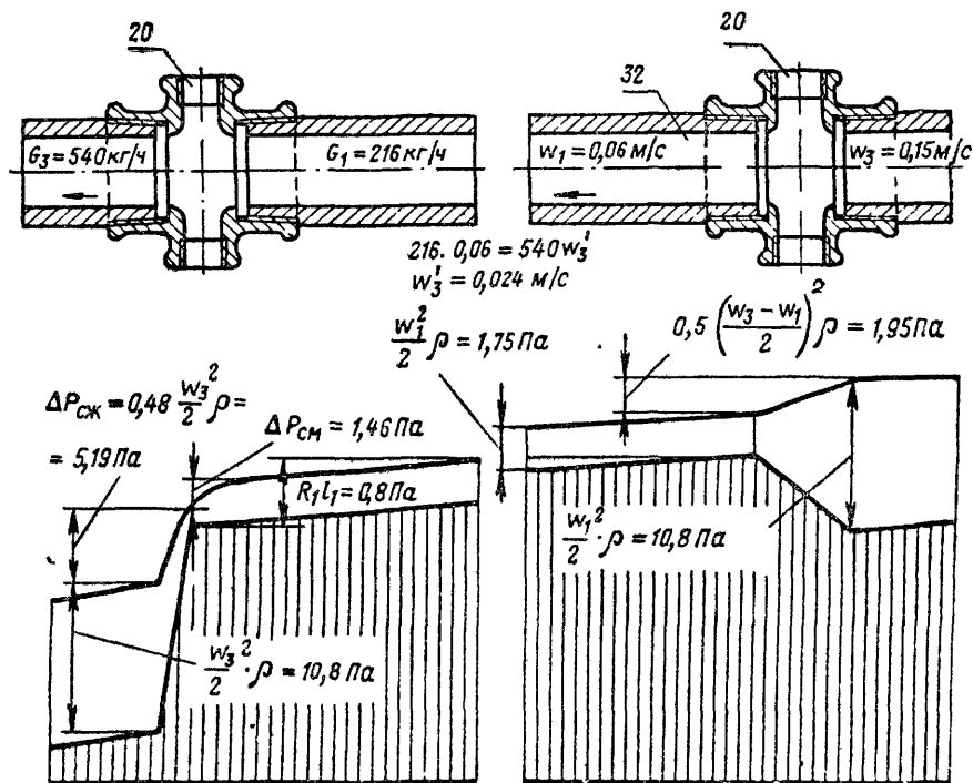
Рис. V.3. Схема распределения давления в замыкающем участке однетрубной системы отопления (без учета геометрической высоты между крестовинами; стояк условно расположен горизонтально)
