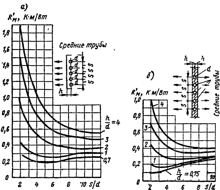
Рис III.6 Графики для определения сопротивления теплопроводности массив бетона, отнесенного к 1 м средних труб отопительной панели, при теплопроводности \lambda_M = 1 \text{ Вт/(м} \cdot \text{К)}
