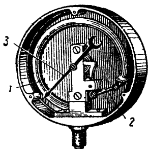
Рис. VI.18. Манометр
