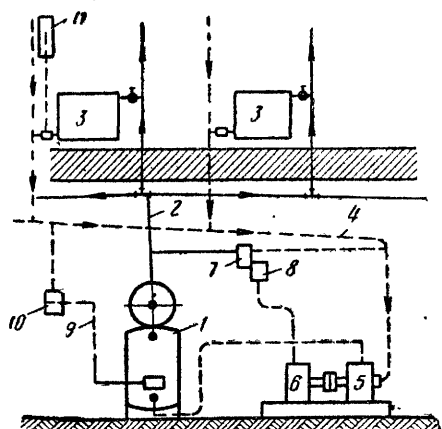
Рис. VI.11. Вакуум-паровая система
