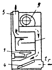
Рис. VII.4. Напольный газозадушный отопительный агрегат
