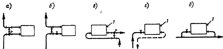
Рис. III.17. Присоединение труб к отопительному прибору
