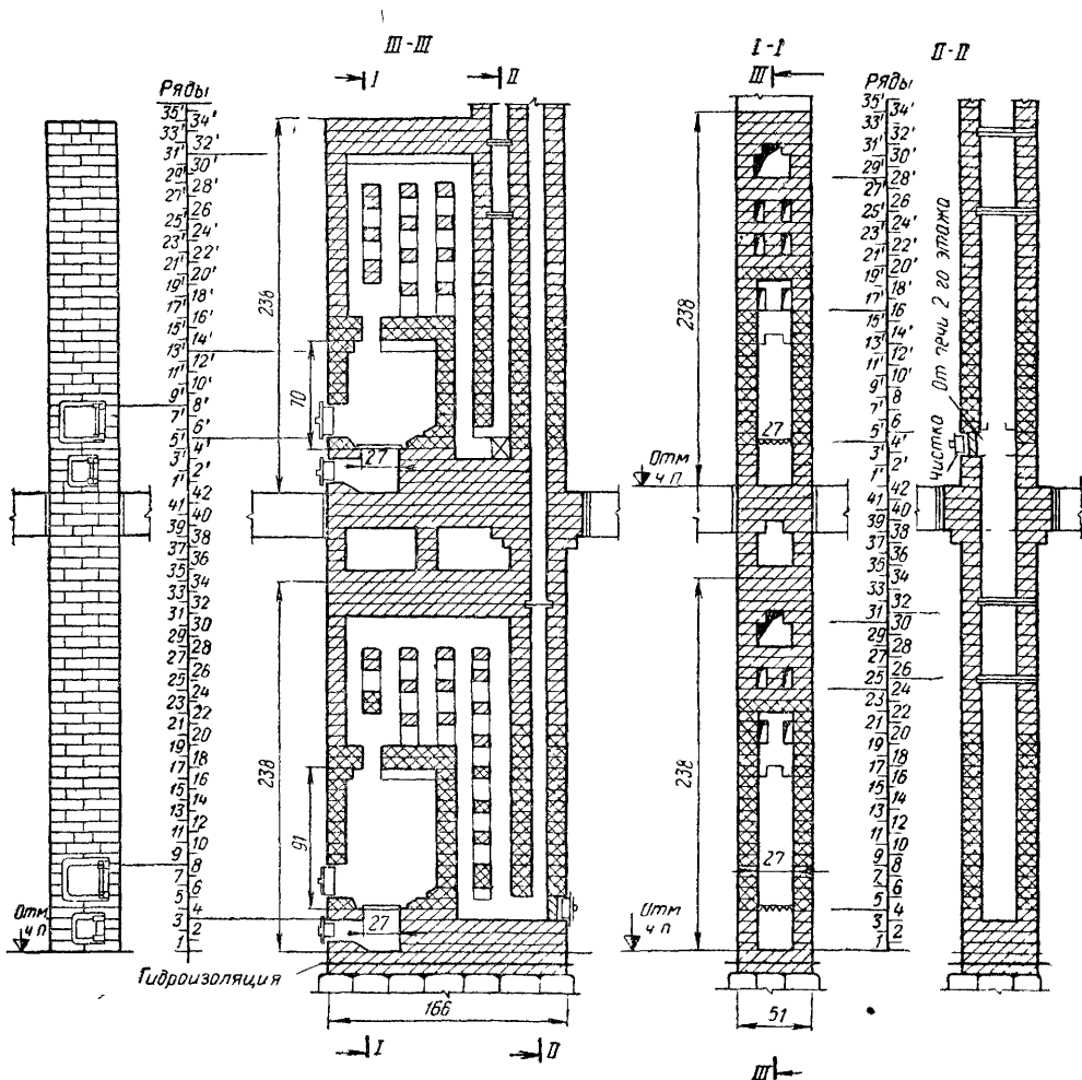
Рис. X.6. Двухъярусная печь
