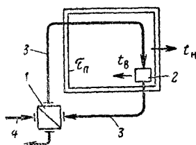
Рис. I.4 Принципиальная схема системы отопления
