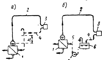
Рис. 1.9. Принципиальные схемы систем парового отопления
