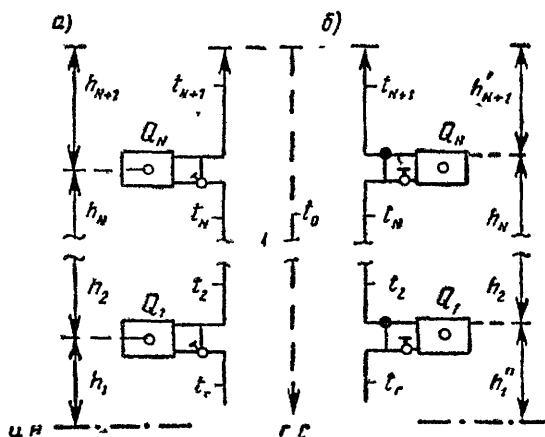
Рис. IV.34 Расчетные схемы вертикальных однетрубных стояков при нижней разводке подающей магистрали и верхней прокладке обратной
