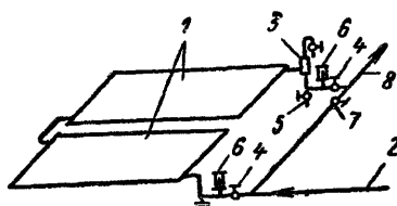
Рис. VIII.12. Схема присоединения напольных панелей к водной системе отопления
