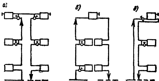
Рис. IV.26. Схемы вертикальных однетрубных стояков при нижней прокладке обеих магистралей
