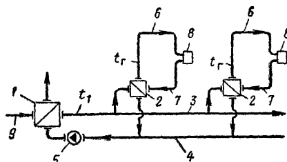
Рис. I.6 Принципиальная схема системы теплоснабжения и отопления 1 и 2 — центральный и местный теплообменники, 3 и 4 — подающий и обратный теплопроводы системы теплоснабжения, 5 — циркуляционный насос, 6 и 7 — подающий и обратный теплопроводы системы отопления, 8 — отопительный прибор, 9 — подвод топлива (тепла)
