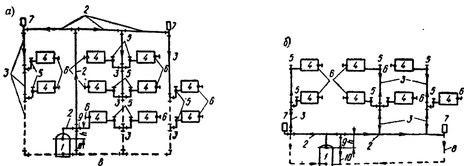
Рис. VI.7. Однотрубная паровая система отопления
