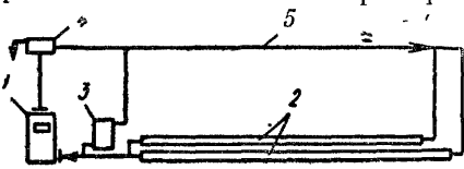
Рис. IV.48. Схема ветви гравитационной системы водяного отопления железнодорожного пассажирского вагона
