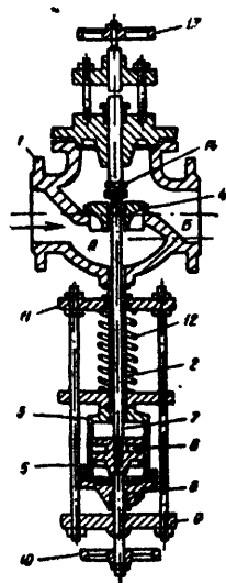
Рис. VI.23. Редукционный клапан
