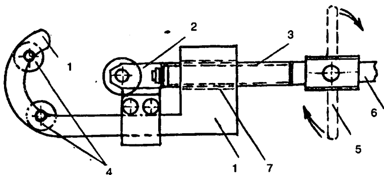
Рис. 68. Трехроликовый трубсрез:
