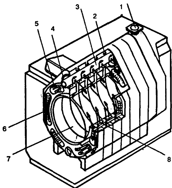
Рис .23. Газовый котел Logano GE- 515: 1 - подающая линия котла; 2 - отверстия выхода воды; 3 - обратная линия котла; 4 - верхняя обечайка; 5 - второй ход продуктов сгорания; 6 - третий ход продуктов сгорания; 7 - топка (первый ход продуктов сгорания)
