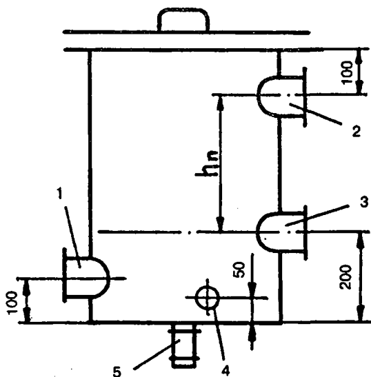
Рис. 53. Открытый демпфер:
