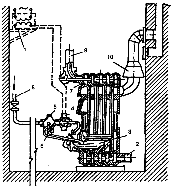
Рис. 14. Секционный водогрейный котел КЧМ-2:
