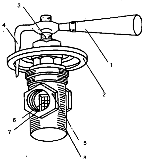
Рис. 46. Кран двойной регулировки: 1 - рукоятка; 2 - розетка; 3 - шпindelь; 4 - упорный палец; 5 - проход корпуса; 6 - боковое окошко; 7 - полный бронзовый стакан; 8 - корпус
