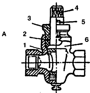
Рис. 50. Проходной кран (А) и кран с дросселирующим устройством (Б):
