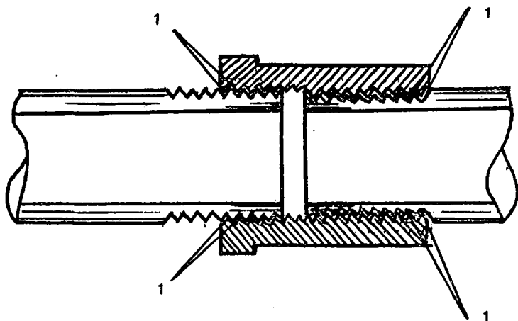
Рис. 64. Сгон: 1 - две нитки сбёга
