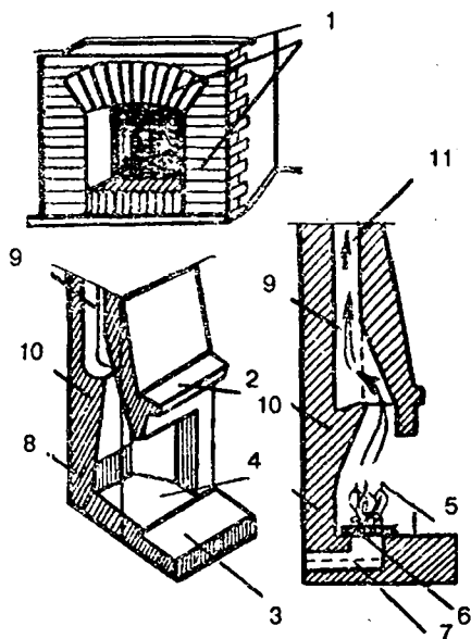
Рис. 107. Элементы конструкции камина:
