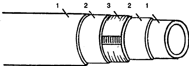
Рис. 44. Металлополимерная труба:
