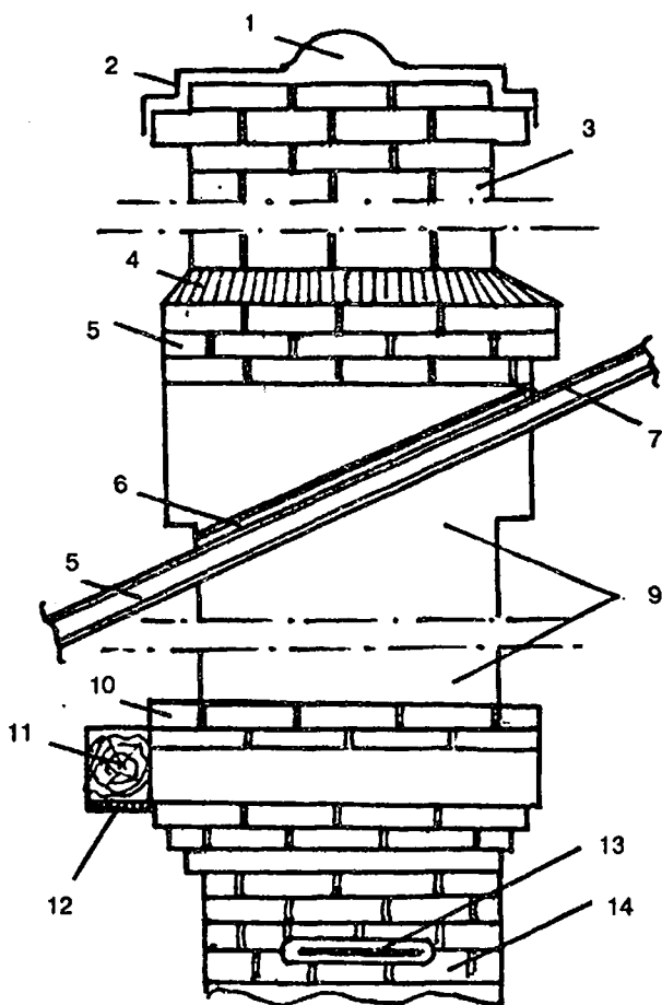
Рис. 94. Насадная дымовая труба:
