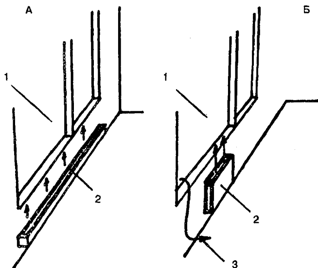
Рис. 32. Воздушные потоки при установке под окном отопительных приборов различных типов:
