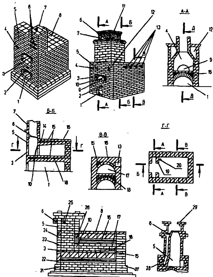
Рис. 103. Традиционная русская печь и щиток:
