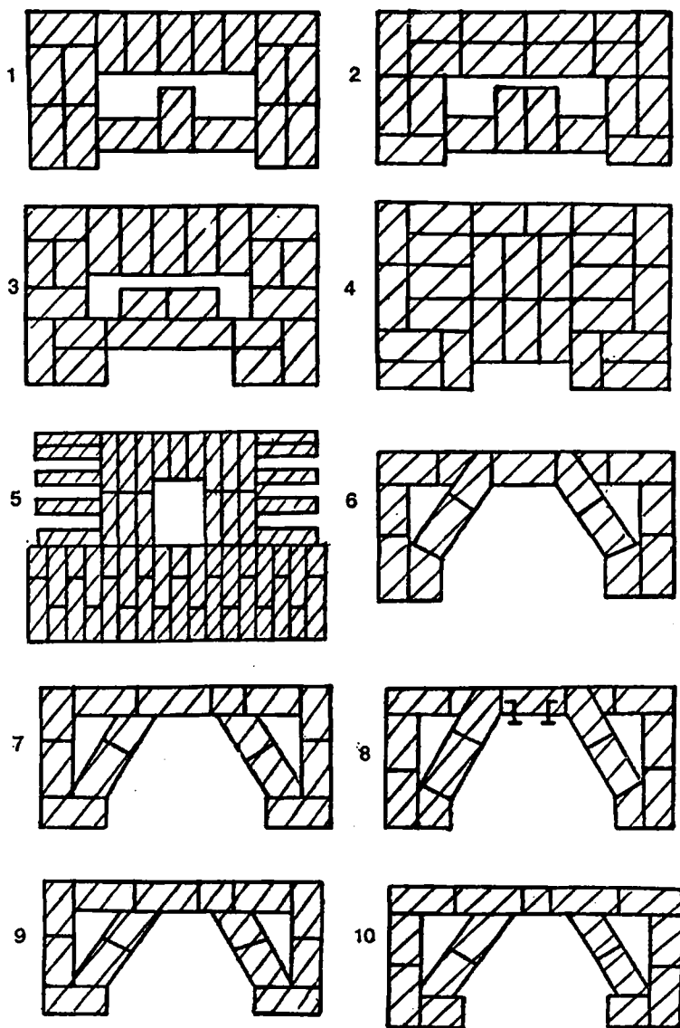
Рис. 109 А. Порядовка камина с арочной перемычкой (1-10 ряды)
