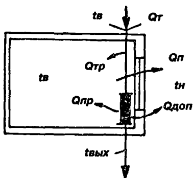
Рис. 29. Потоки теплопередачи от прибора, расположенного у внешнего ограждения дома:
