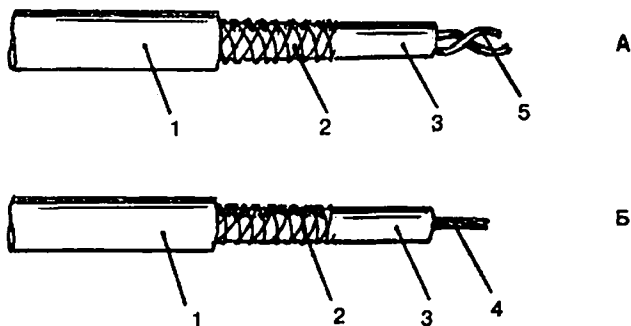
Рис. 77. Двухпроводниковый (А) и однопроводниковый (Б) бронированные кабели:
