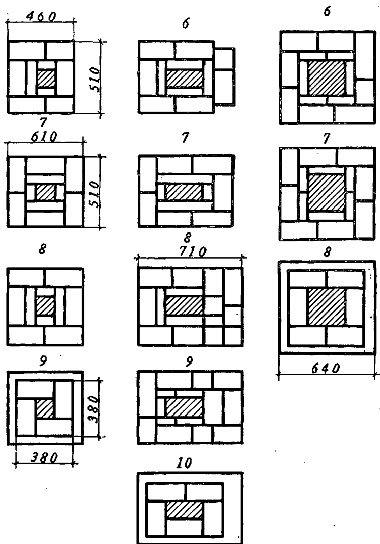
Рис. 96 А. Кладка выдры: А - кладка 6-9 рядов дымового канала сечением 130х130 мм; Б - 6-10 ряды дымового канала сечением 130х250 мм; В - 6-8 ряды дымового канала сечением 250х250 мм
