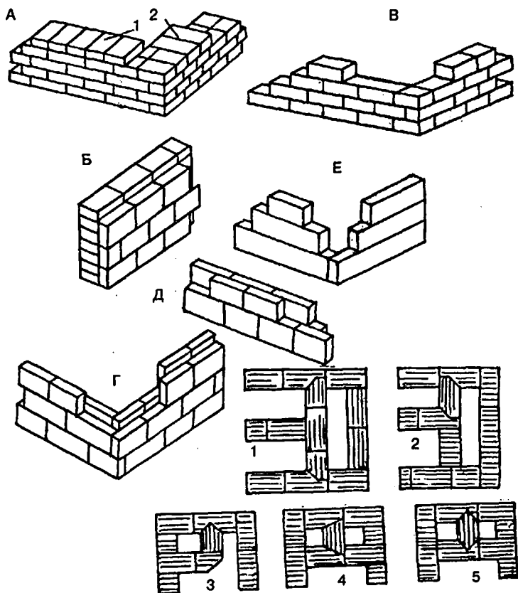
Рис. 90. Варианты печной кладки и кладки замков: А - кладка в один кирпич; 1 - тычки; 2 - ложки; Б - кладка в 3/4 кирпича; В - кладка в 1/2 кирпича; Г - кладка в 1/4 кирпича; Д - кладка в 1/2 кирпича (две четвертки на ребро); Е - 1/2 кирпича с полным перекрытием швов; 1 - 5 - варианты замков
