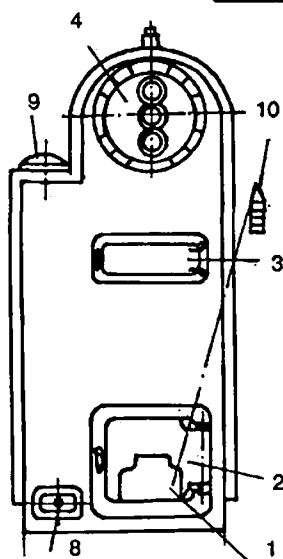
Рис. 17. Котел с дровяной топкой из листовой стали:
