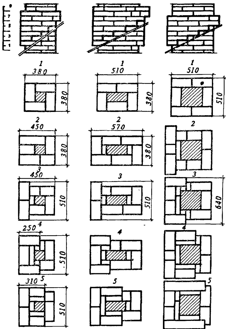
Рис. 96. Кладка выдры:
