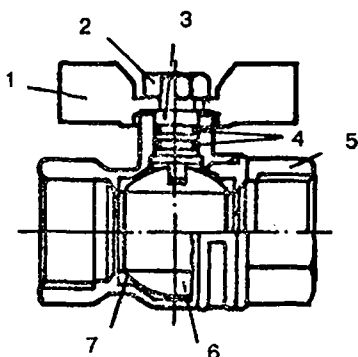
Рис. 52. Шаровой кран:
