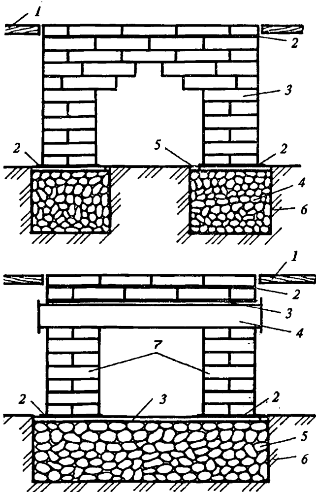
Рис. 84 А. Столбчатый фундамент для печей: А - первый вариант: 1 - пол; 2 - выравнивающий слой; 3 - кладка; 4 - кирпичный щебень и гравий; 5 - гидроизоляция; 6 - грунт; Б - второй вариант: 1 - пол; 2 - гидроизоляция; 3 - выравнивающий слой; 4 - железобетонные перемычки или плита; 5 - фундамент в грунте из бутового камня и щебня; 6 - грунт; 7 - столбики из кир- пичной кладки
