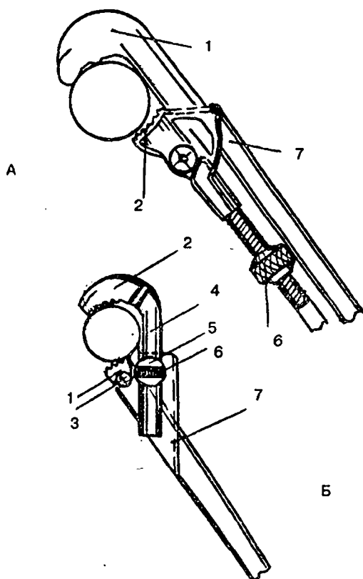
Рис. 65. Трубные ключи:
