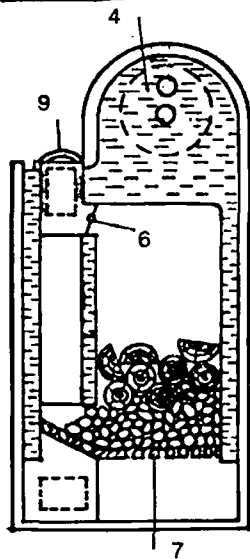
Рис. 17. Котел с дровяной топкой из листовой стали:
