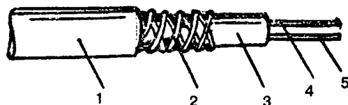
Рис. 80. Нагревательный кабель марки ЕСО: 1 - оболочка из ПВХ-пластика; 2 - оплетка из медной проволоки; 3 - теплоустойчивый ПВХ-пластик; 4 - вспомогательная жила из отожженной меди; 5 - нагревательная жила
