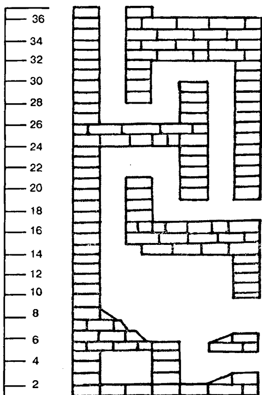
Рис. 102. Отопительная печь с толстыми стенками
