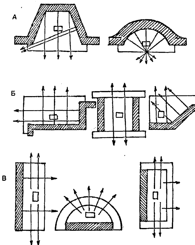
Рис. 106. Разновидности каминов по виду излучения тепла: А - односторонняя поверхность излучения; Б - двухсторонняя поверхность излучения; В - трехсторонняя поверхность излучения
