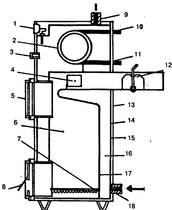
Рис. 21. Котел "Пламя":
