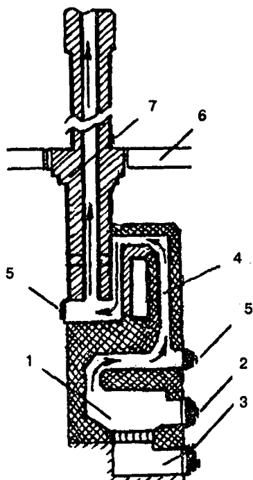
Рис. 87. Дымоход печи:
