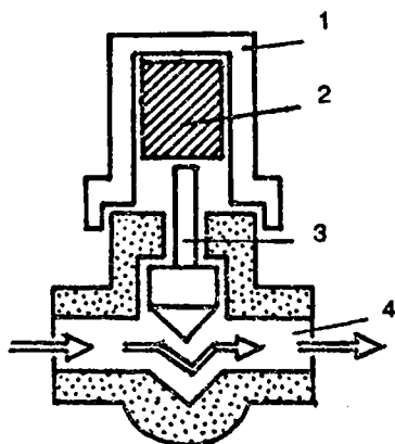
Рис. 48. Термостат: 1 - термоголовка; 2 - рабочее вещество; 3 - клапан; 4 - вода
