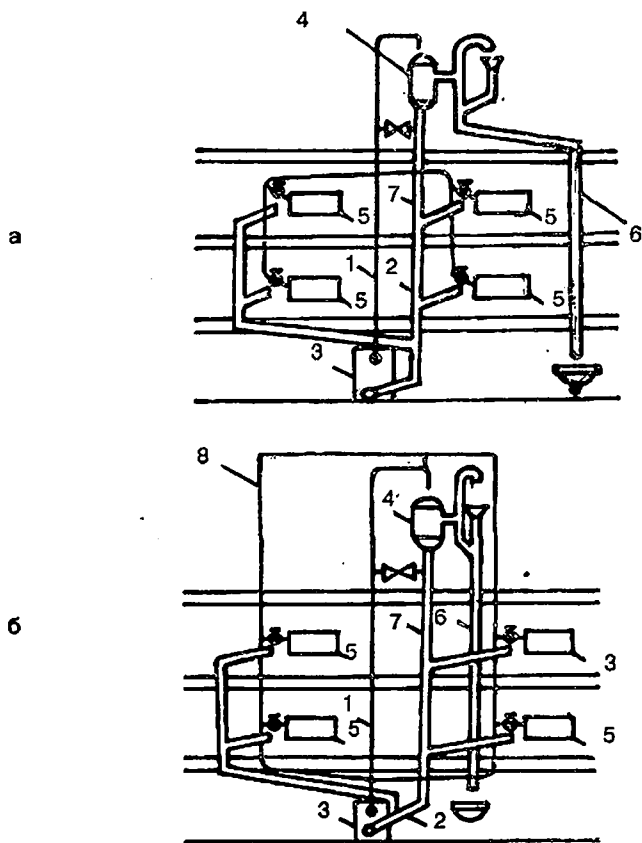
Рис. 6. Двухтрубная схема водяного отопления: а - с верхней разводкой; б - с нижней разводкой; 1 - главный стояк; 2 - трубопровод обратной воды; 3 - котел; 4 - расширительный бачок; 5 - нагревательные приборы; 6 - перелив; 7 - предохранительный трубопровод; 8 - воздушная труба
