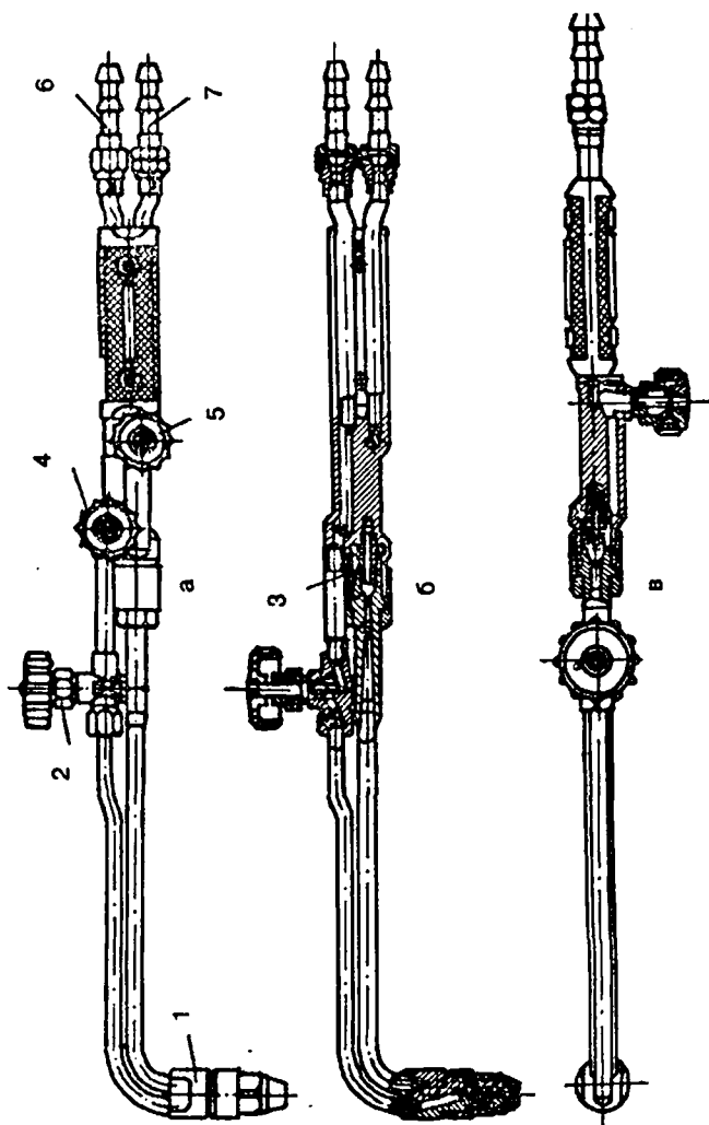
Рис. 67. Резак газовый:
