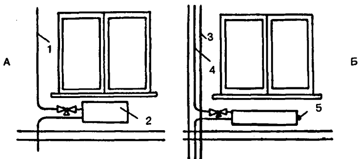
Рис. 61. Монтаж стояков:
