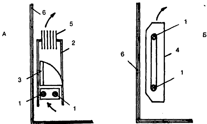
Рис. 34. Конвекторы:
