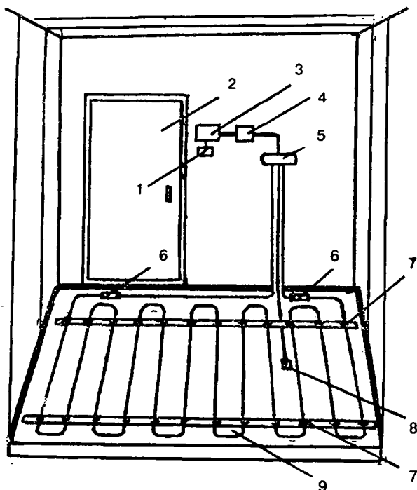
Рис. 73. Схема монтажа напольного кабельного обогрева: 1 - выключатель; 2 - дверь; 3 - регулятор; 5 - распаечная коробка; 6 - соединительные муфты; 7 - монтажная лента; 8 - датчик; 9 - нагревательная секция
