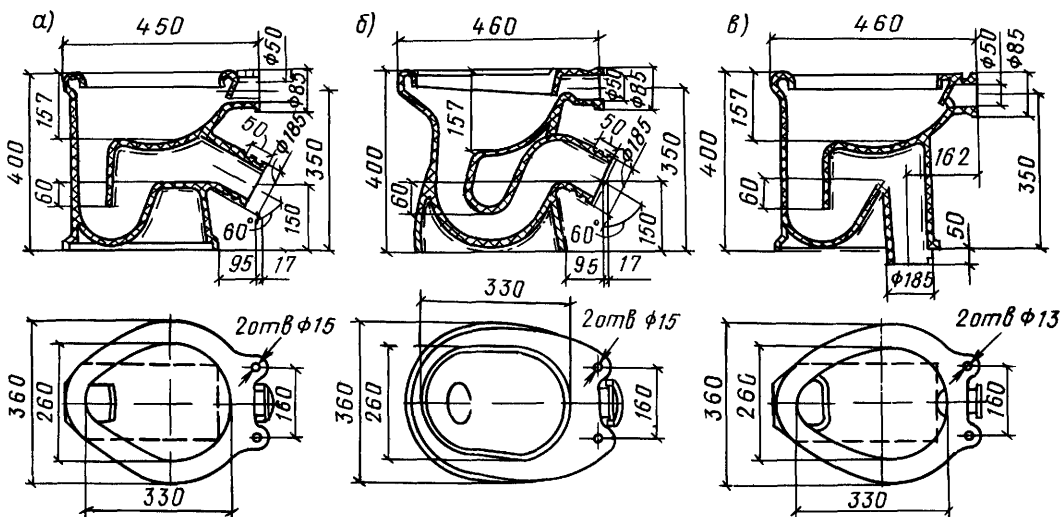
Рис. XI.1. Унитаз тарельчатый
