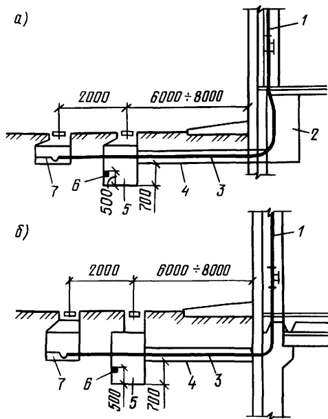
Рис. 15.2. Схема устройства выпуска водостока или канализации а в бесподвальном здании, б-при наличии подвала, 1 стояк, 2 приемок размером 1 \times 1 м, 3-выпуск, 4-непроходной железобетонный канал, 5 контрольный колодец, 6 сигнализатор аварийного уровня, 7 колодец на сети
