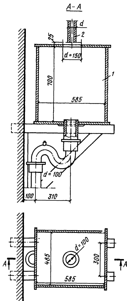
Рис. 8.3. Установка бачка для разрыва струи 1 — бакоч для разрыва струи; 2 — переливная труба
