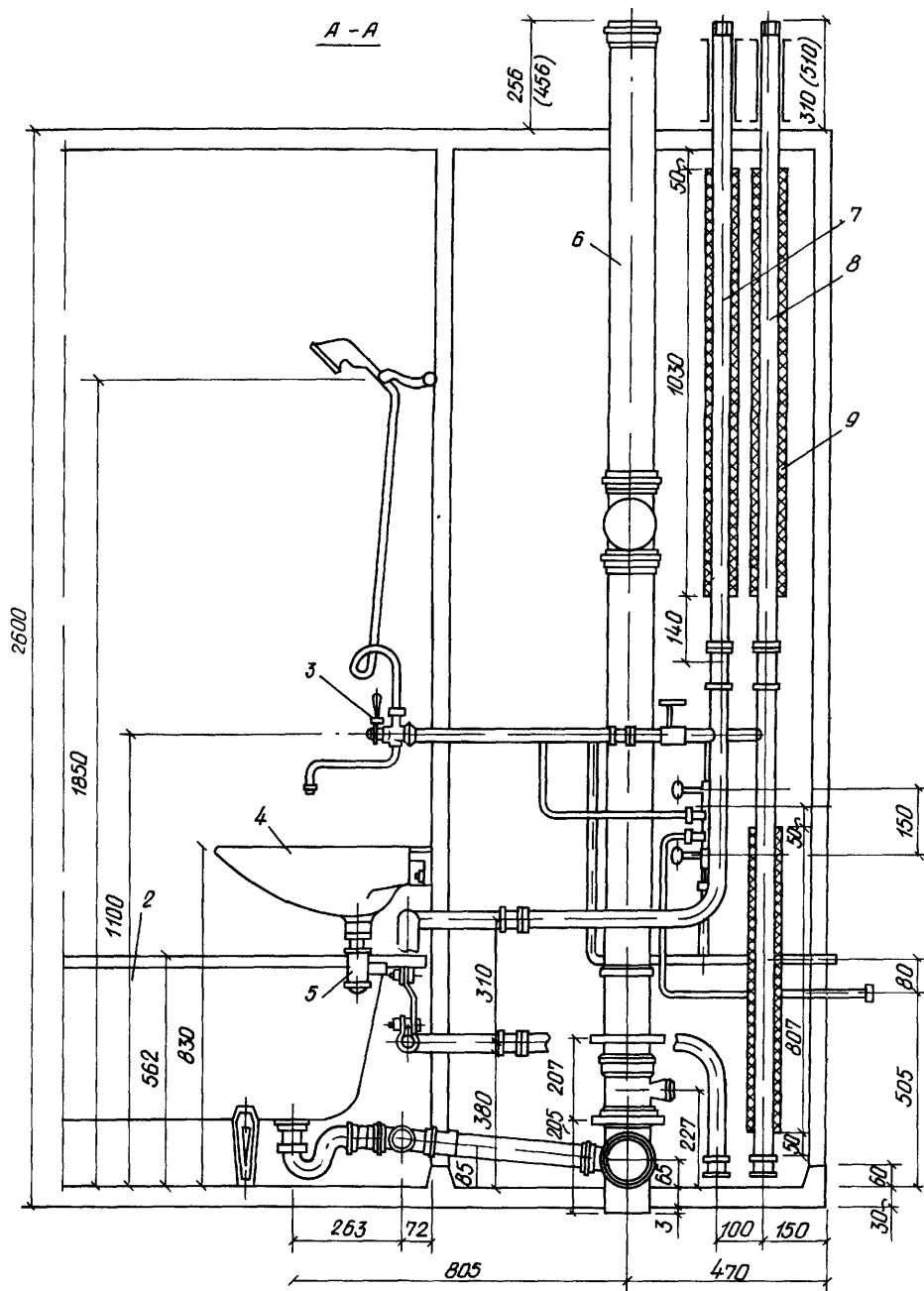
Рис. 11.1. Унифицированная санитарно-техническая кабинка раздельного типа
