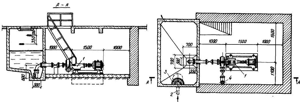
Рис. 12.5. Размещение канализационных насосов в здании 1 — насос, 2 — проточная труба, 3 — решетка, 4 — напорный трубопровод
