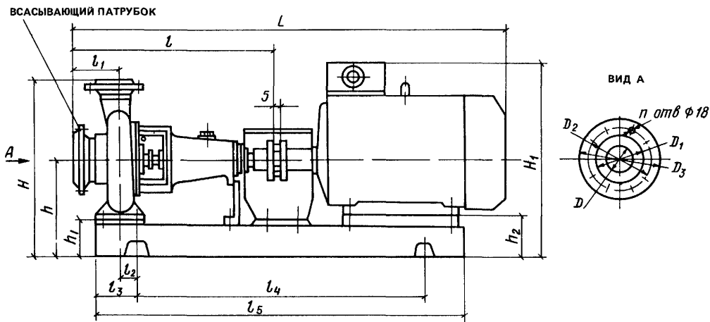
РАЗМЕРЫ, мм, ЦЕНТРОБЕЖНЫХ КОНСОЛЬНЫХ НАСОСОВ ТИПА К
