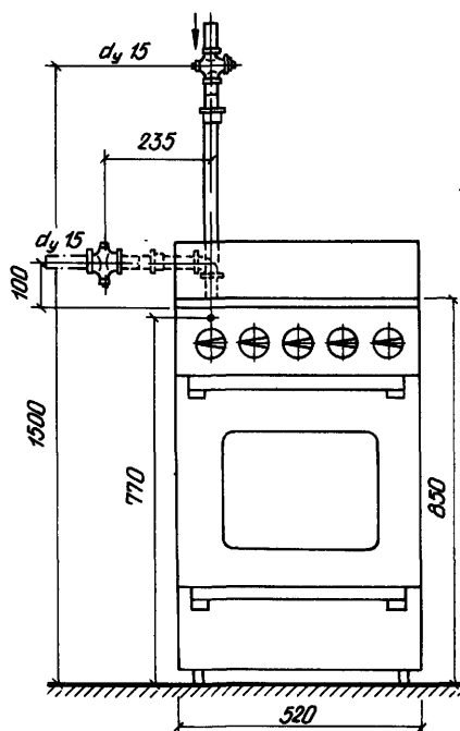
Рис. 17.1. Установка четырехгорелочной бытовой газовой плиты
