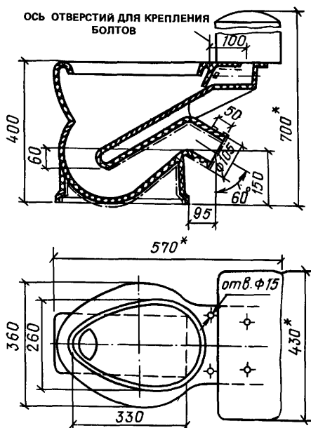
Рис. XI.4. Унитаз козырьковый с цельноотлитой полочкой с косым выпуском типа КПИ-КВ
