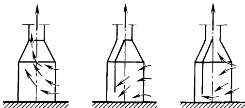
Рис. 8.17. Укрытия шкафного типа
