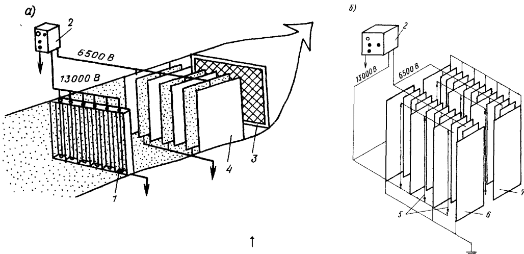
Рис. 4.6. Принципиальная схема двухзонного электрического фильтра
