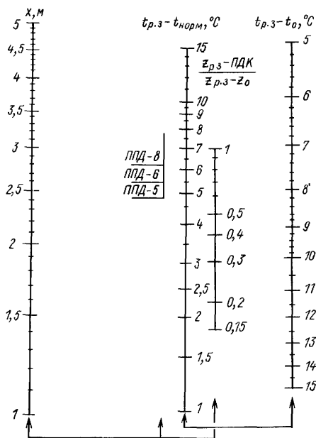
Рис. 6.11. Номограмма для определения типоразмера ППД
