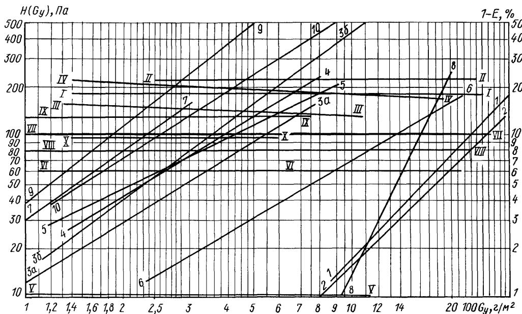
Рис. 4.4. Пылевая характеристика фильтра и фильтрующих материалов
