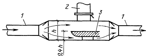
Рис 9 2 Приемная коробка
