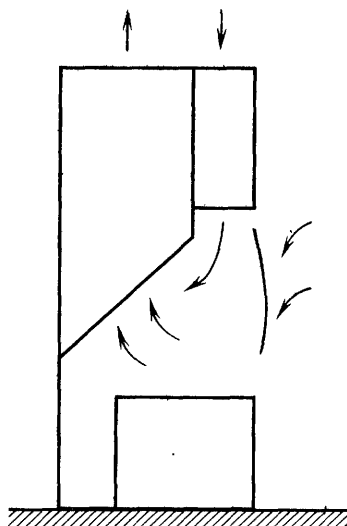
Рис. 8.14. Компенсационное воздушно-струйное укрытие
