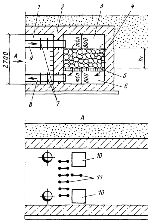
Рис. 14.5. Гравийный охладитель
