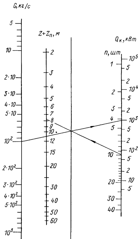
Рис. 5.3. Номограмма для определения высоты расположения температурного перекрытия Z (при c_p = 1 кДж/(кг·°C); T_{р.з} = 298 К; \rho_{р.з} = 1,18 кг/м³). Ключ: G = 100 кг/с; Q_k = 1000 кВт; n = 10 ; Z + Z_n = 7,6 м
