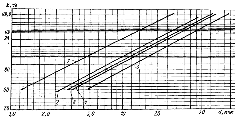
Рис 4.10 Фракционная эффективность циклонов ВНИИОГАЗа
