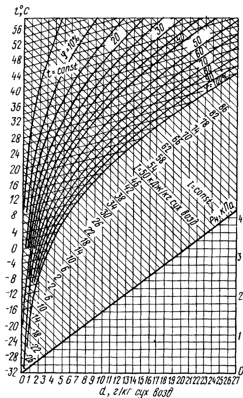
Рис. 1.1. I - d -диаграмма влажного воздуха
