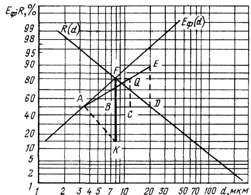
Рис. 4.12. К примеру расчета циклона ЦН-15 графоаналитическим методом
