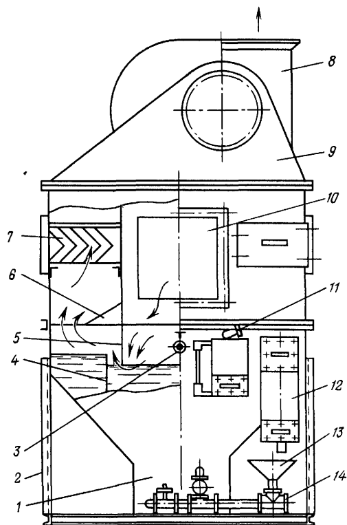
Рис. 4.13. Устройство пылеуловителя ПВМ
