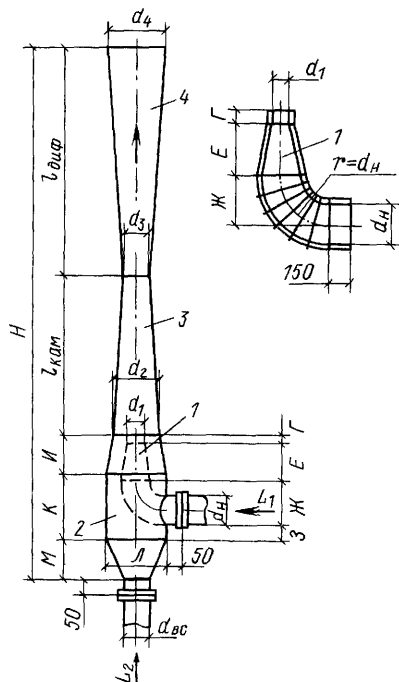
Рис. 10.2. Эжектор низкого давления
