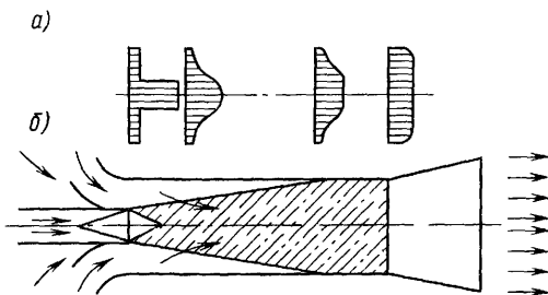
Рис. 10.1 Схема распределения скоростей воздуха по длине камеры смешения эжектора
