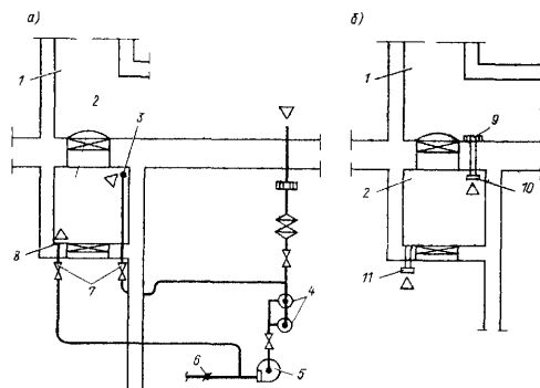
Рис. 14.6. Продувка тамбура входа
