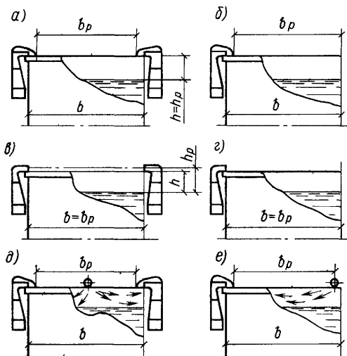
Рис. 8.8 Бортовые отсосы от ванн
