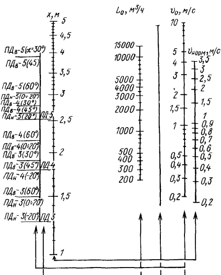
Рис. 6.14. Номограмма для определения расхода воздуха на ПД
