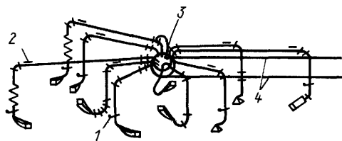
Рис 9 3 Кустовая система с малогабаритным коллектором
