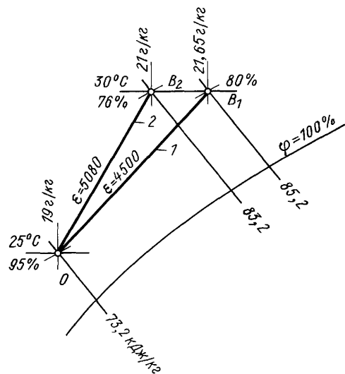
Рис 14.8 I-d -диаграмма
