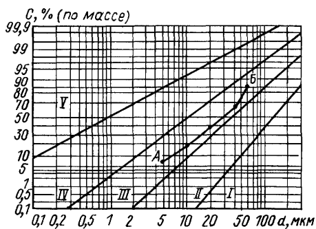
Рис. 4.2. Классификационная номограмма пылей
