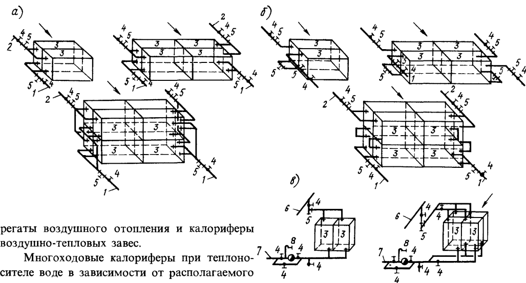
Рис 11.5 Схемы подводов теплоносителя к калориферам
