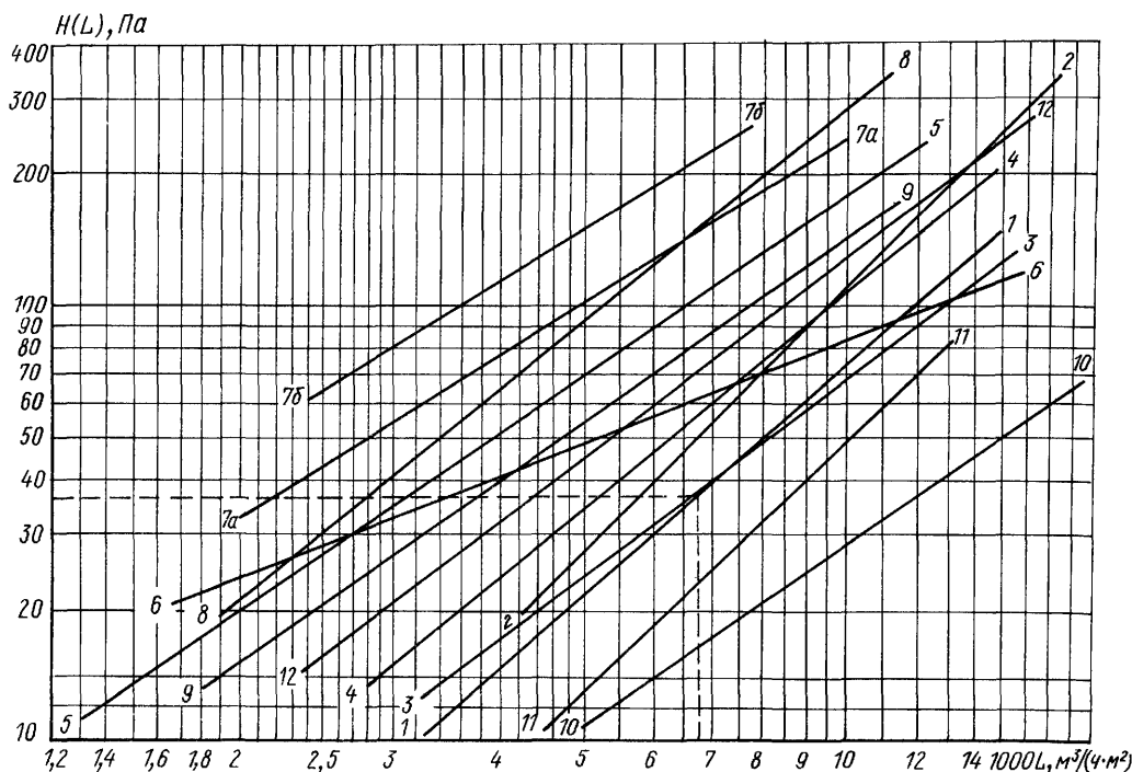
Рис 4.3 Аэродинамические характеристики фильтров и фильтрующих материалов
