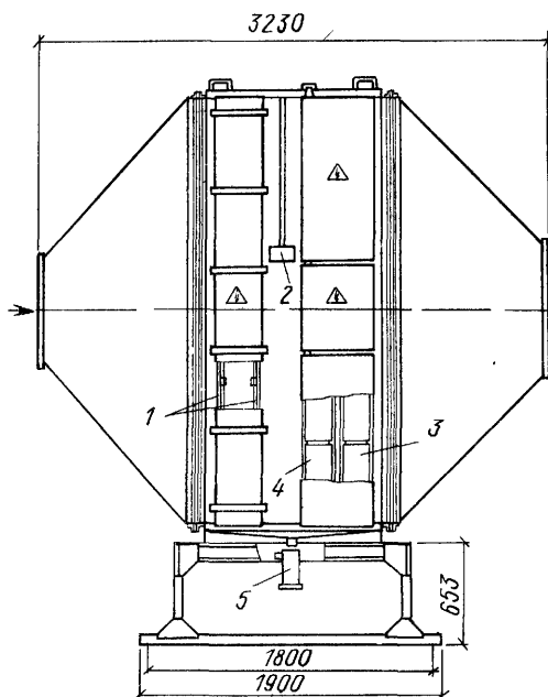
Рис 4.16. Двухкаскадный электрический уловитель масляных аэрозолей ЭФУ202
