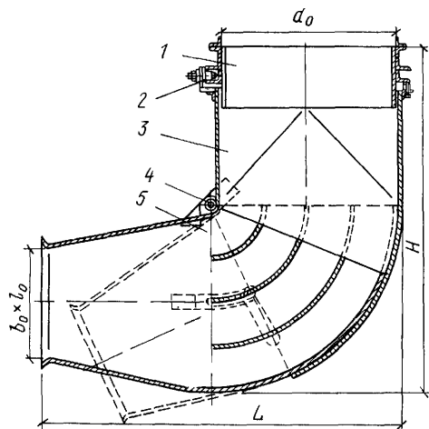
Рис. 6.3. Поворотный душирующий патрубок типа ВПД
