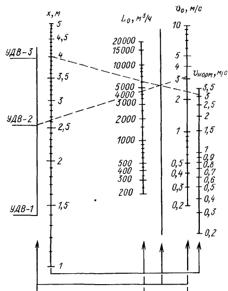
Рис. 6.10. Номограмма для определения расхода воздуха на УДВ
