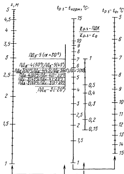
Рис. 6.13. Номограмма для определения типоразмера ПД
