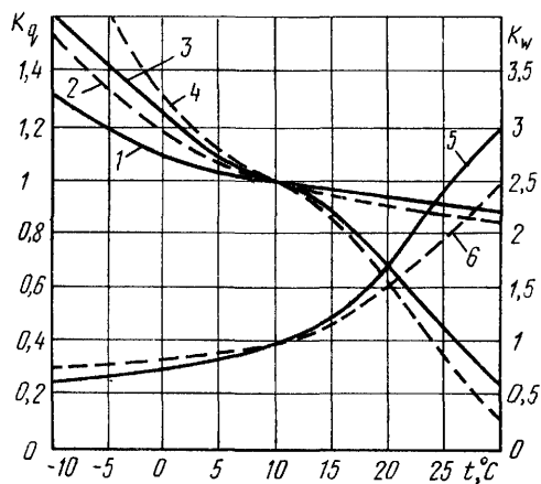
Рис. 3.1. Коэффициенты отклонения тепловыделений K_q и влаговывделений K_w животных в зависимости от температуры воздуха в помещениях
