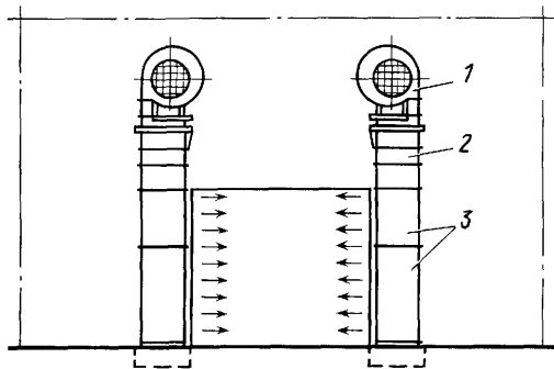
Рис 7.1 Двусторонняя воздушно-тепловая завеса шиберного типа
