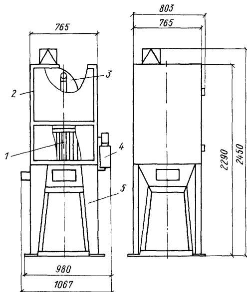
Рис. 4.17. Тканевый пылеуловитель АІ-БПШ
