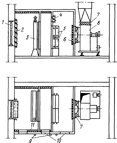
Рис. 11.3. Компоновка приточной камеры
