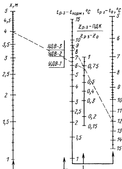
Рис. 6.9. Номограмма для определения типоразмера УДВ
