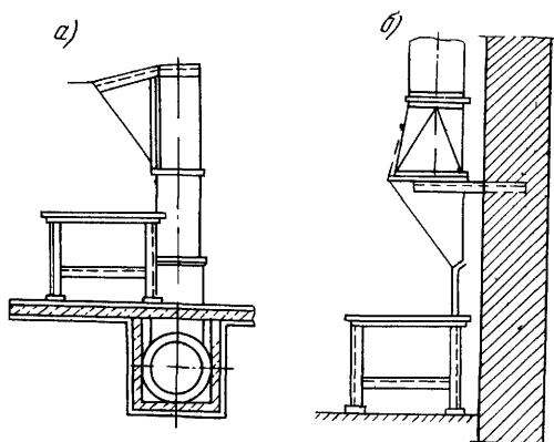
Рис. 8.7 Панели равномерного всасывания у стационарных постов сварки
