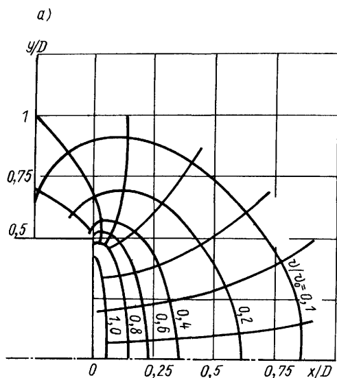
Рис 8.1 Распределение скоростей в зоне действия всасывающих отверстий
