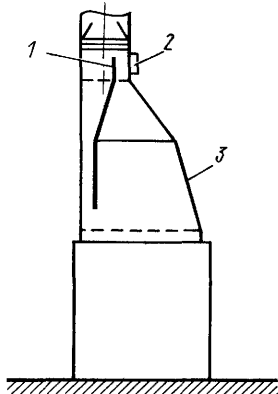
Рис. 8.18. Вытяжной шкаф с комбинированным отсосом
