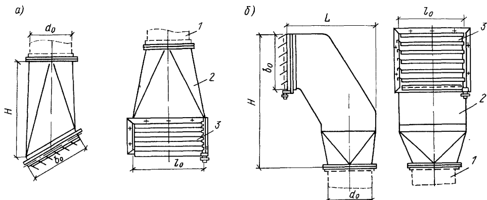
Рис. 6.4. Душирующие патрубки типа ПД
