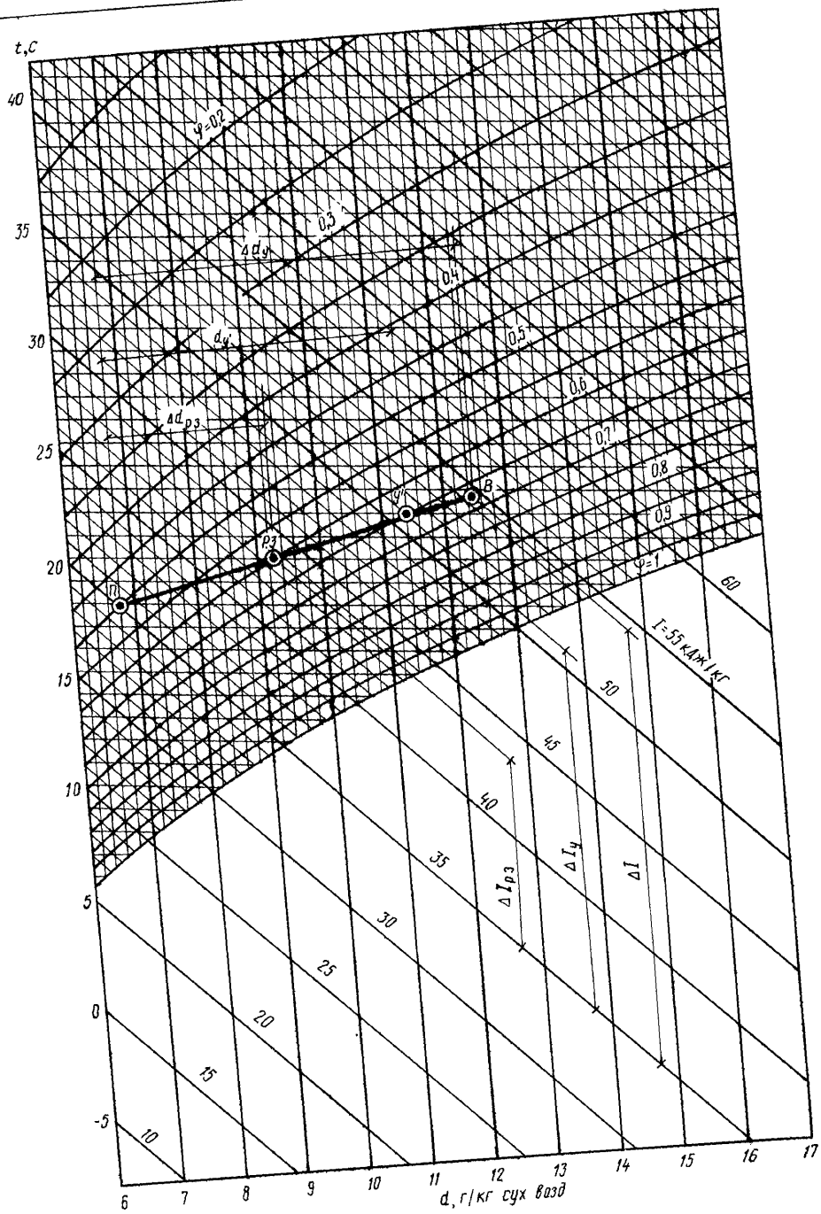
Рис. 2.11. Графический расчет вентиляции с использованием I-d -диаграммы
