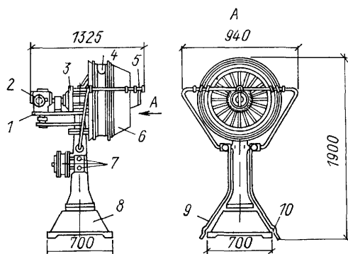
Рис. 6.7. Поворотный аэратор ПАМ-24
