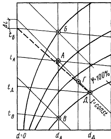
Рис. 1.2. Построение процесса на I - d -диаграмме для случая 1
