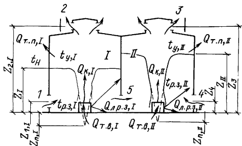
Рис. 5.4. Схема аэрации двухпролетного здания
