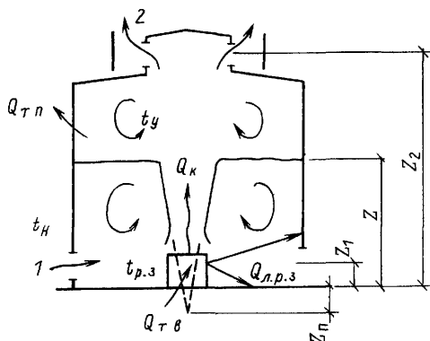
Рис. 5.1. Схема аэрации однопролетного здания 1 и 2 номера проемов
