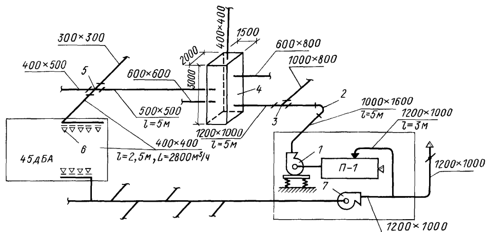
Рис. 12.6. Схема расчетной ветви воздуховодов
