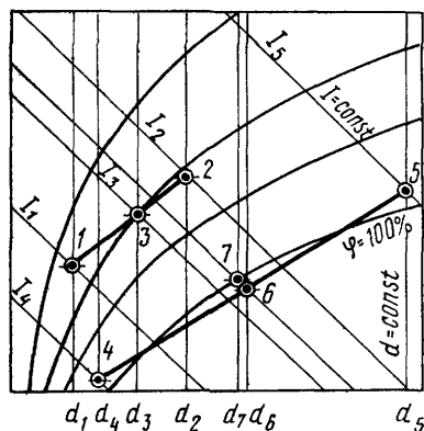
Рис. 1.3. Построение процесса на I - d -диаграмме для случая 2
