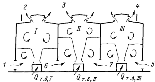
Рис. 5.6. Схема аэрации трехпролетного здания с тепловыделениями во всех пролетах
