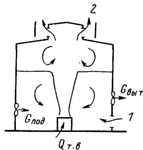
Рис. 5.8. Схема аэрации здания, оборудованного местной механической вентиляцией
