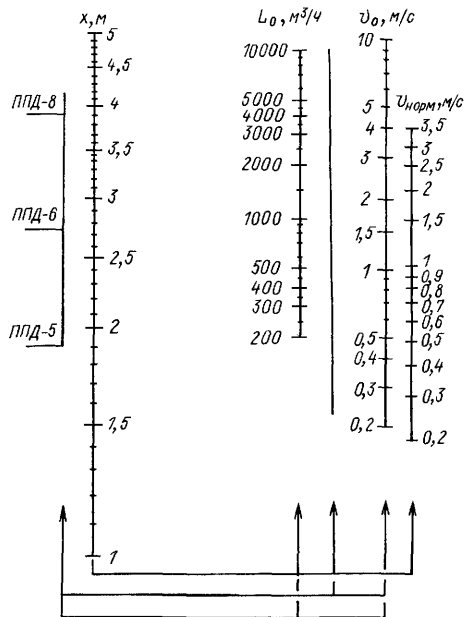
Рис. 6.12. Номограмма для определения расхода воздуха на ППД
