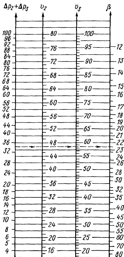
Рис. 10.4. Схема эжектора высокого давления
