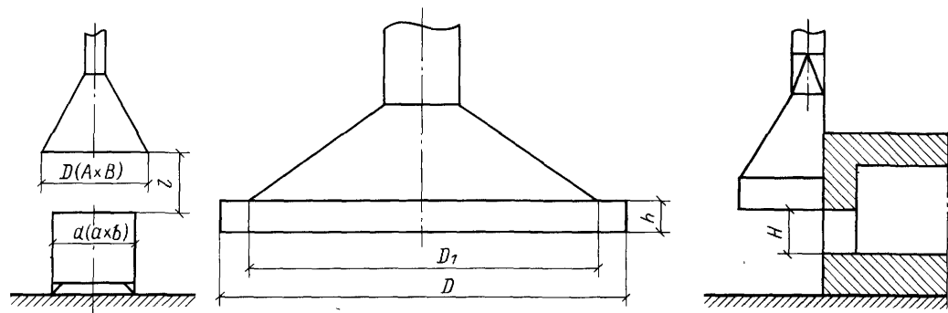
Рис. 8.3. Вытяжной зонт над теплоисточником
