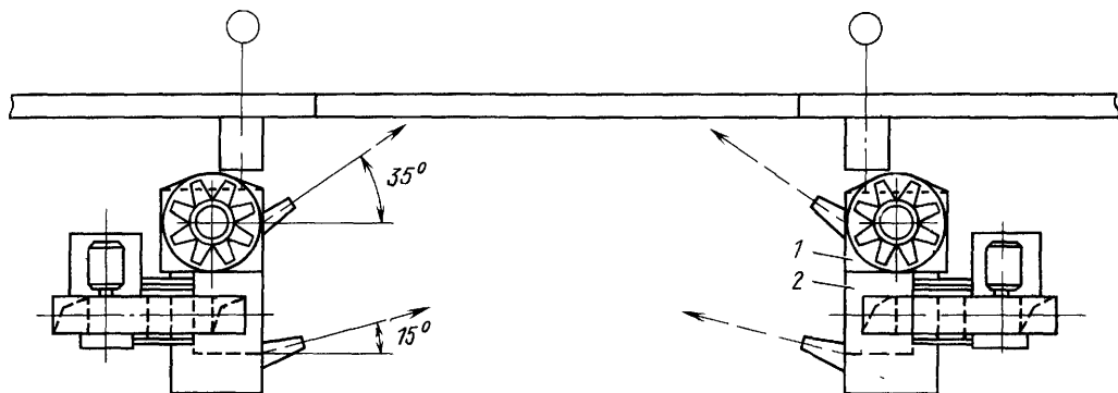
Рис 7.5. Комбинированная воздушно-тепловая завеса
