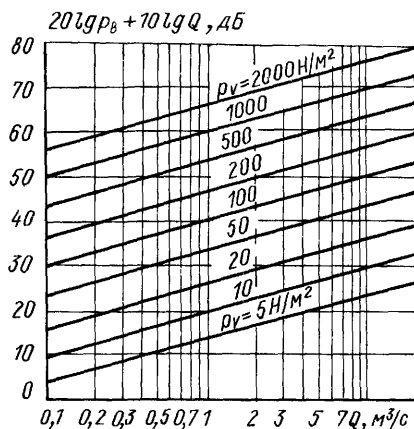
Рис. 12.2. К определению значений 20 \lg p_n + 10 \lg Q
