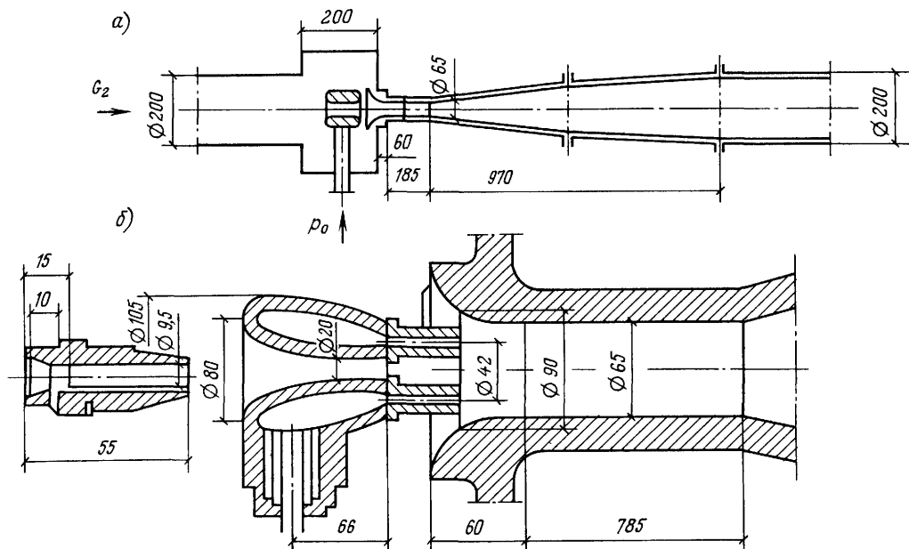
Рис 10.9. Многоструйный эжектор
