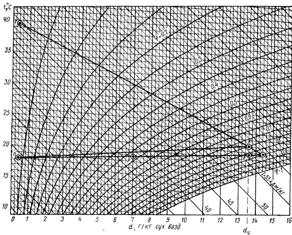
Рис. 2.13. Ход расчета продувки верхней зоны помещения на t-d -диаграмме
