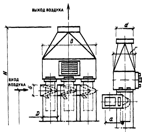
Рис IV.14. Группа из трех циклонов с ЦН-15 с выходом воздуха через колпак
