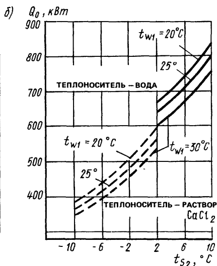
Рис. 16.2. Зависимости холодопроизводительности Q_0 от температуры хладонносителя t_{s2} и охлаждающей воды t_{w1} для хладоновой машины марки 21МКТ 280-2-1 (а) и 2МКТ 350-2-1 (б)
