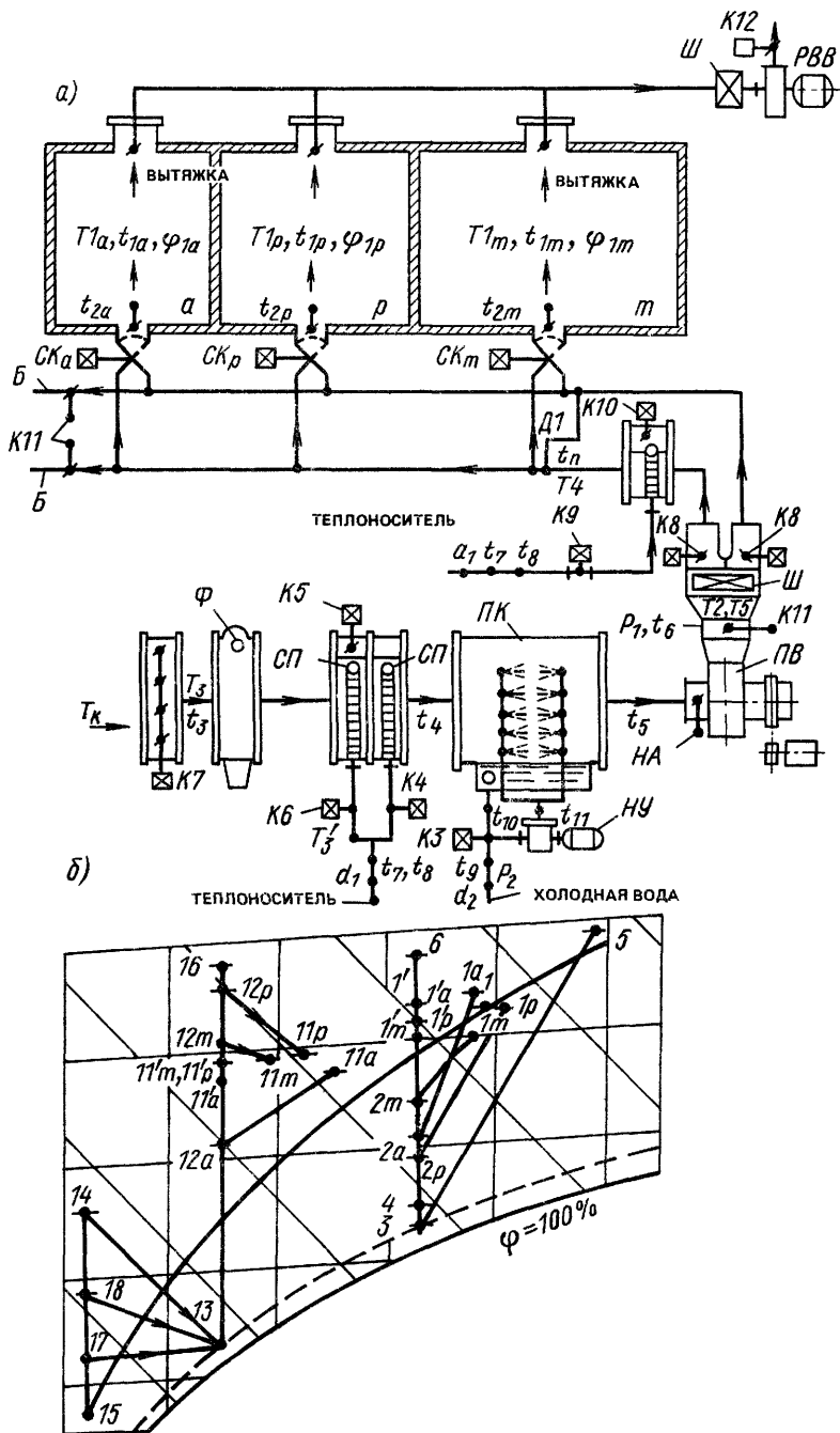
Рис 15.16. Центральная многозональная двухканальная система кондиционирования воздуха, работающая на наружном воздухе
