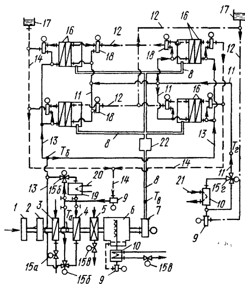
Рис. 15.20. Схема центральной одноканальной четырехтрубной эжекционной СКВ с вводом к ЭКД холодного первичного воздуха, горячей и холодной воды 1—приемный клапан; 2—фильтр; 3—воздухонагреватель; 4—охладитель воды для холодного периода года; 5—воздухоохладитель; 6—форсуночная камера орошения; 7—вентилятор; 8—воздуховод; 9—насос; 10—водоподогреватель; 11—трубопровод горячей воды; 12—трубопровод отработавшей горячей воды; 13 и 14—трубопроводы холодной и отработавшей холодной воды; 15—автоматические клапаны регуляторов температуры T_a , T_b , T_c ; 16—эжекционные кондиционеры-доводчики с воздухоохладителем и воздухонагревателем; 17—расширитель; 18—клапан регулятора РТК-5215 ИТС-15
