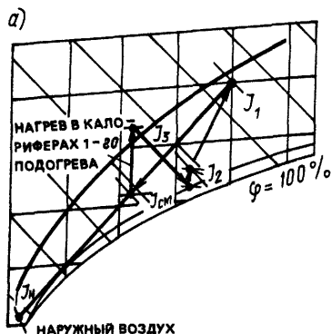
Рис. 15.6. Схемы обработки воздуха в системе, работающей с переменными расходами наружного и рециркуляционного воздуха (а и б) и с постоянными расходами (а и в), при условии, что расход наружного воздуха меньше вычисленного по формуле (15.16)
