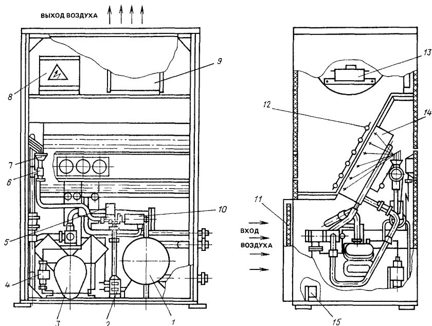
Рис. III.16. Кондиционер КПА1-3,5-04
