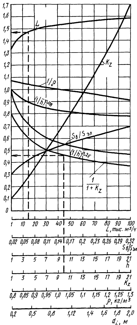
Рис. 22.2. Номограмма вспомогательных величин для определения v^{\text{эк}}
