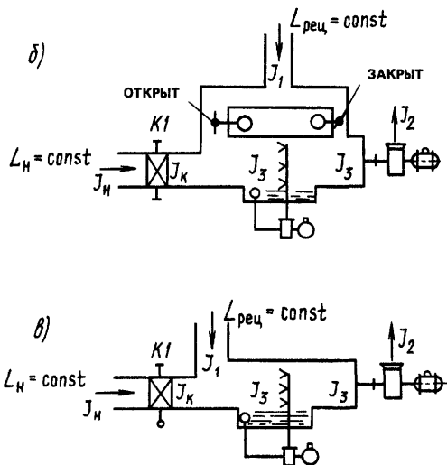
Рис. 15.7. Схемы обработки воздуха в системе, работающей с постоянным расходом наружного воздуха при применении первой и второй рециркуляции (а и б), и в системе, работающей без применения второй рециркуляции (а и в), при условии, что расход наружного воздуха больше или равен вычисленному по формуле (15.16)
