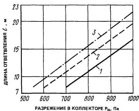
Рис. 22.7. График для приближенного определения разрежения в сборном магистральном коллекторе (1), вертикальном шаровом сборнике (2) и горизонтальном сборнике (3)
