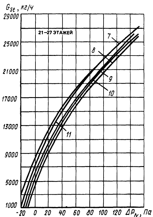
Рис 20.2. Номограммы для определения расхода наружного воздуха G_{st} , нагнетаемого в незадымляемую лестничную клетку 2-го типа в зависимости от разности давления между лестничной клеткой и лифтовой шахтой \Delta P_N на уровне верхнего этажа и от давления в лифтовой шахте на первом этаже p_i
