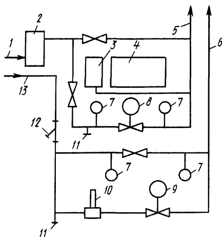
Рис 15.36. Узел управления доувлажнительной установки «Туман»
