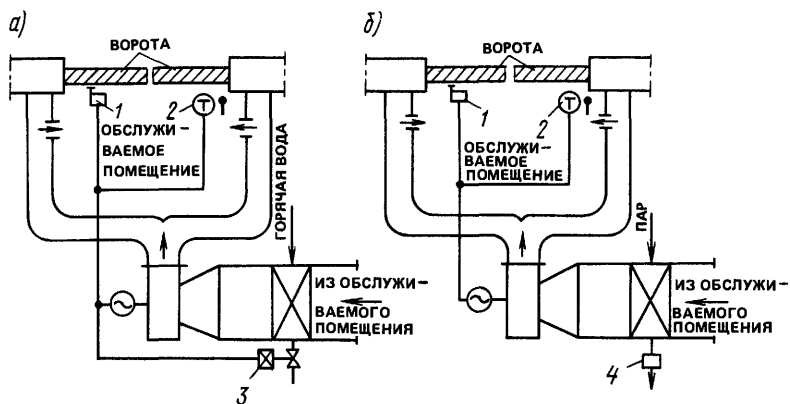
Рис. 19.5. Воздушно-тепловые завесы с теплоносителем водой (а) и теплоносителем паром (б)
