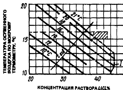
Рис. 15.53. Зависимость конечной температуры воздуха по мокрому термометру от концентрации водного раствора хлористого лития и температуры воды, охлаждающей раствор t_{\text{ок}} (по И. И. Чернобыльскому, О. А. Кремневу и А. С. Чавдарову)
