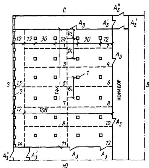
Рис. 20.1. План цеха к примеру расчета 20.1 (А – эвакуационные выходы из горящего помещения)
