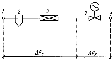
Рис. 18.2. Схема регулируемого участка 1 — прямая и обратная магистрали; 2 — фильтр; 3 — воздушонагреватель; 4 — регулирующий клапан
