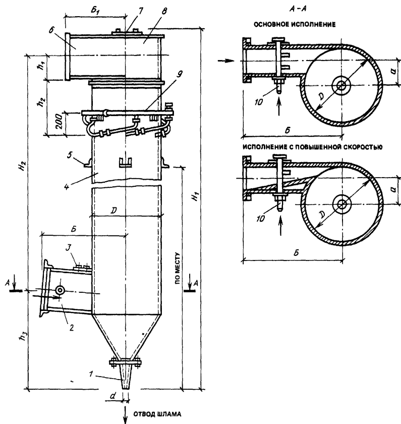
Рис. IV.28. Пылеуловители ЦВП
