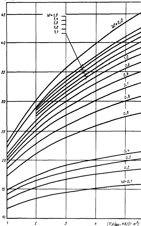
Рис. 21.6. Определение коэффициентов теплопередачи K воздухонагревателей КТЦ-3 двухрядных (раствор \text{CaCl}_2 ).
