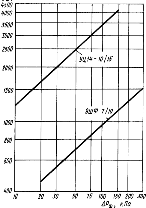
Рис. 15.26. Зависимости расхода воды q_\phi от давления воды перед форсунками \Delta p_\phi
