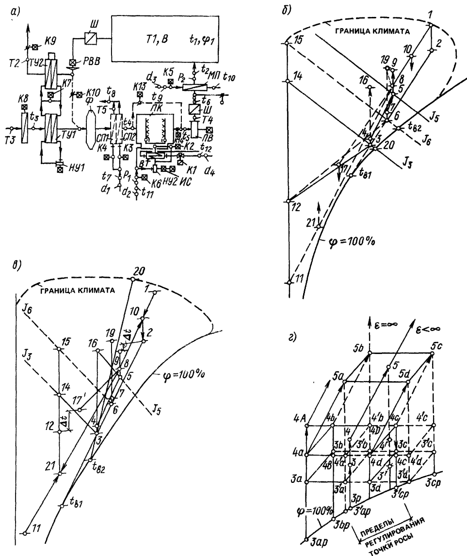
Рис. 15.8. Центральная прямоточная однозональная система кондиционирования воздуха, работающая полностью на наружном воздухе или с рециркуляцией (рециркуляционный воздуховод и клапан K10 показаны пунктиром)
