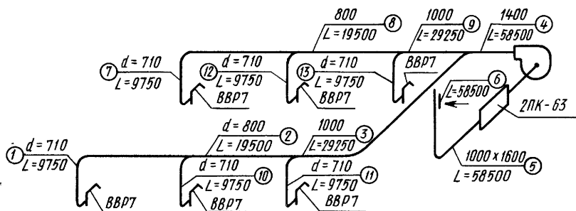
Рис. 22.6. Расчетная схема сети воздуховодов общего назначения
