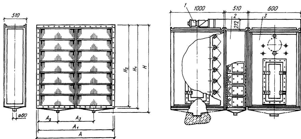
Рис. IV.5. Электрофильтр ФЭ
