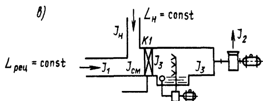
Рис. 15.6. Схемы обработки воздуха в системе, работающей с переменными расходами наружного и рециркуляционного воздуха (а и б) и с постоянными расходами (а и в), при условии, что расход наружного воздуха меньше вычисленного по формуле (15.16)
