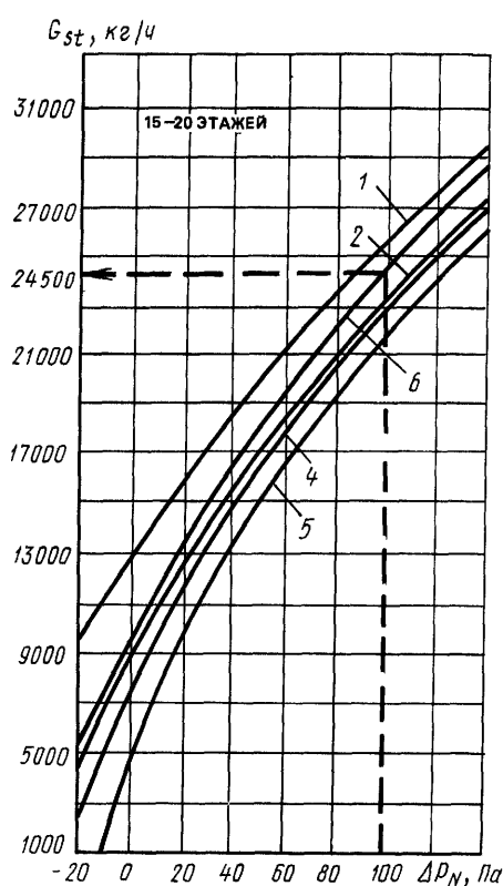
Рис 20.2. Номограммы для определения расхода наружного воздуха G_{st} , нагнетаемого в незадымляемую лестничную клетку 2-го типа в зависимости от разности давления между лестничной клеткой и лифтовой шахтой \Delta P_N на уровне верхнего этажа и от давления в лифтовой шахте на первом этаже p_i
