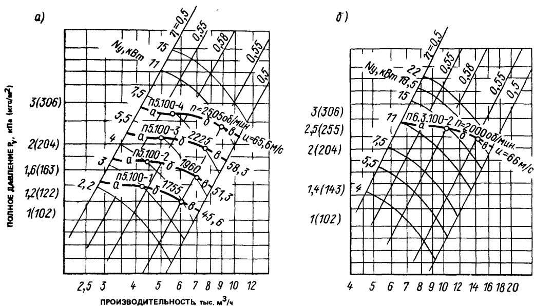
Рис. 1.23. Аэродинамические характеристики пылевых вентиляторов В.ЦПБ-45-5 (а) и В.ЦПБ-45-6,3 (б) (исполнение б)
