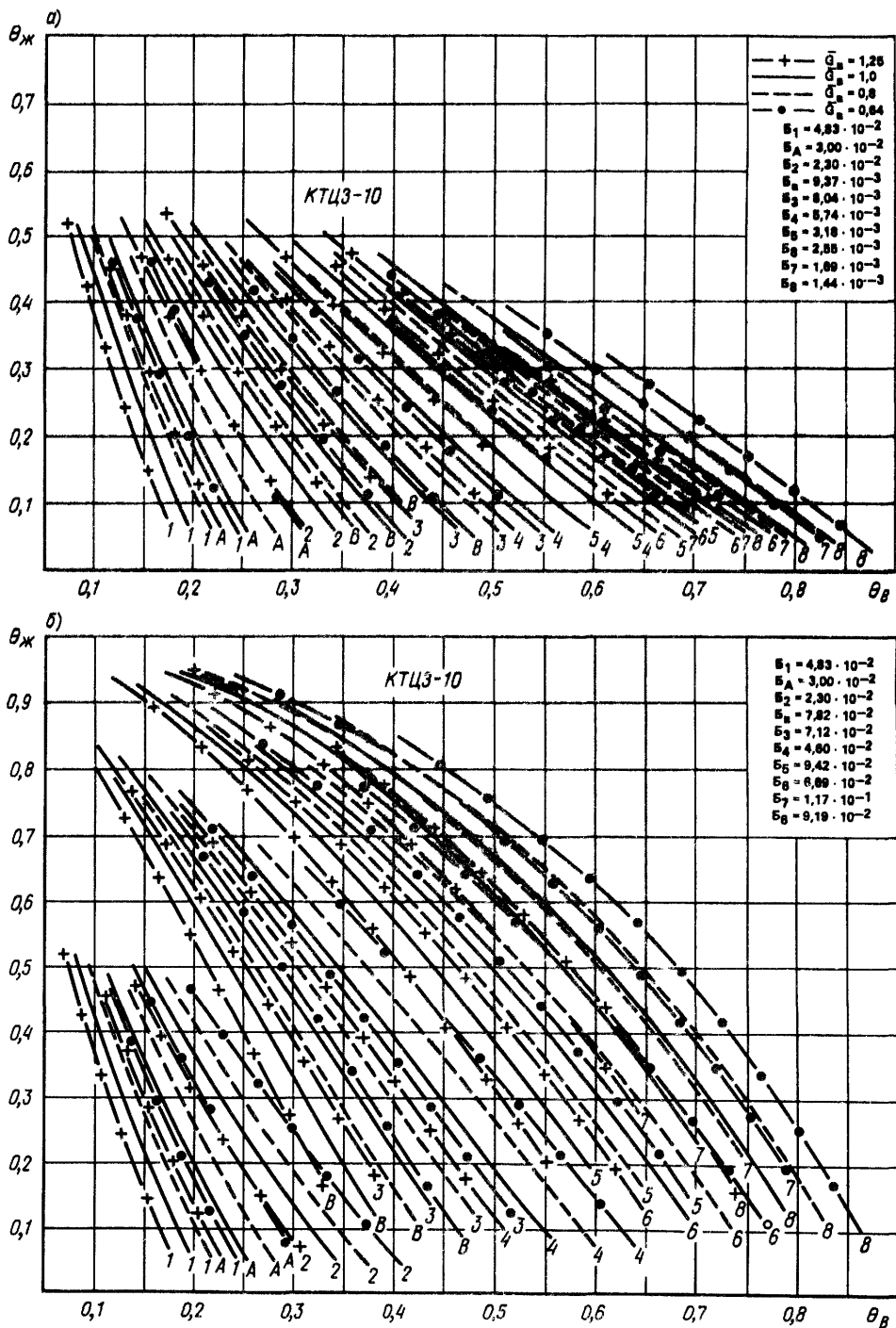
Рис. 15.40. Теплотехнические и гидравлические характеристики теплообменников кондиционеров КТЦ3-10 и КТЦ3-20 с параллельной схемой обвязки (а, б) и последовательно-противоточной (б, з)
