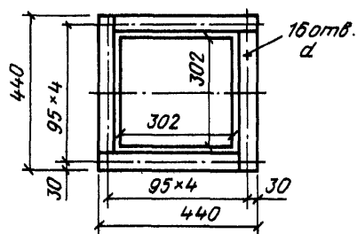
ФЛАНЕЦ БУНКЕРА D = 650-800 \text{ мм}
