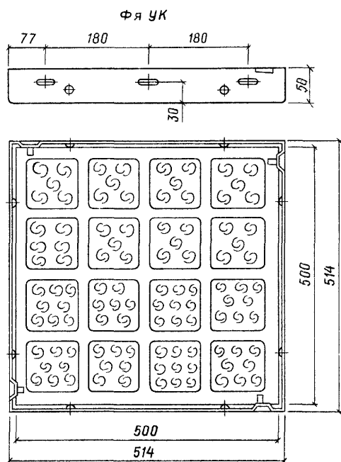
Рис. IV.1. Унифицированные ячейки фильтра Фя
