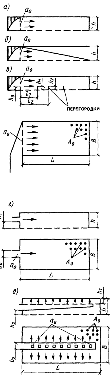
Рис. 17.8. Схемы подачи воздуха в подшивное пространство
