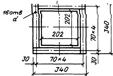
ФЛАНЕЦ БУНКЕРА D = 650-800 \text{ мм}
