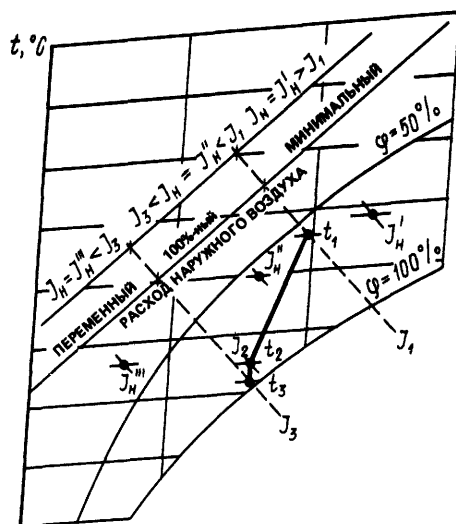
Рис. 15.4. Определение расхода наружного воздуха, необходимого для уменьшения интенсивности запахов, связанных с пребыванием в помещении людей 1 и 2 — ошутимый и умеренный запах; 3 и 4 — сильный и очень сильный запах
