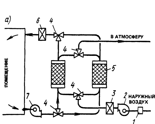
Рис. 15.57. Принципиальные схемы воздушосушителей с неподвижным слоем поглощающего материала и автоматическим переключением с режима адсорбции на режим реактивации
