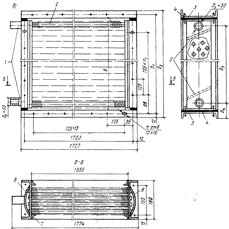
Рис. П.2. Калориферы КСК4-6-02ХЛЗА — КСК4-10-02ХЛЗА (а) и КСК4-11-02ХЛЗА и КСК4-12ХЛЗА (б)
