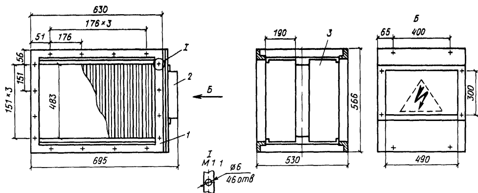
Рис. IV.6 Электрофильтр ЭФ-2М
