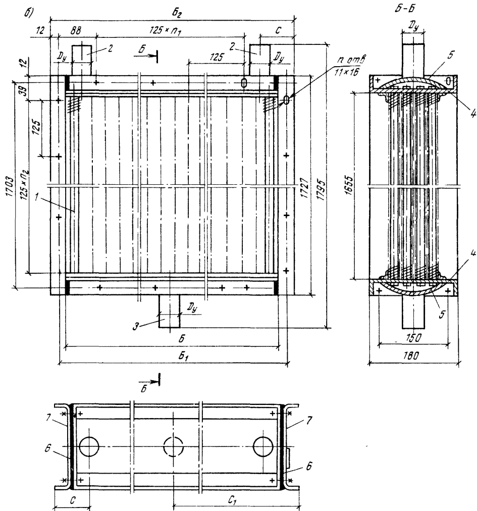
Рис. II.3. Воздуонагреватели (калориферы) КП36-СК-01УЗА – КП310-СК-01УЗА (а), КП311-СК-01УЗА и КП312-СК-01УЗА (б)
