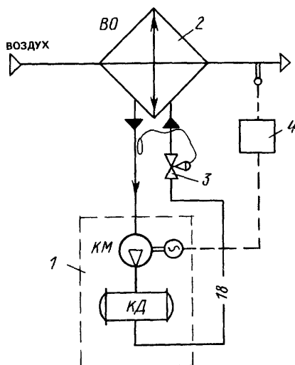
Рис 16.3. Схема непосредственного охлаждения воздуха с помощью хладонового воздухоохладителя
