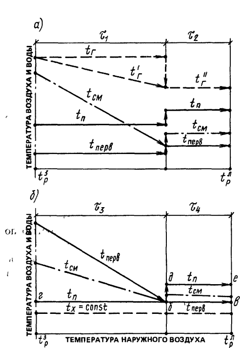
Рис 15.21 Графики изменения температуры первичного воздуха, холодной и горячей воды, поступающих к доводчикам одноканальных СКВ, поддерживающих в помещении температуру воздуха
