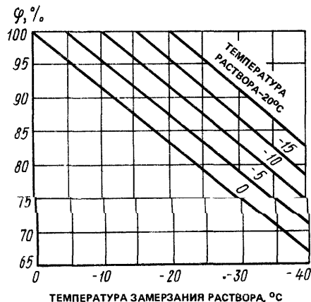
Рис. 15.45. Относительная влажность воздуха \varphi в пограничном слое над водными растворами солей
