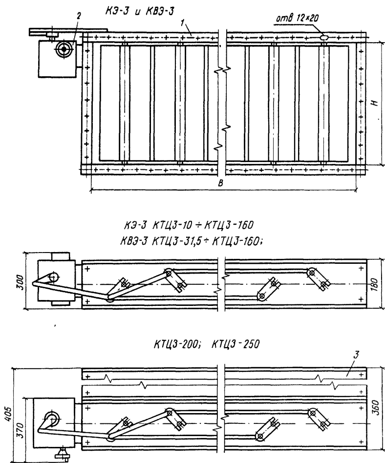
Рис. III.11. Клапаны воздушные КЭ-3 и КВЭ-3
