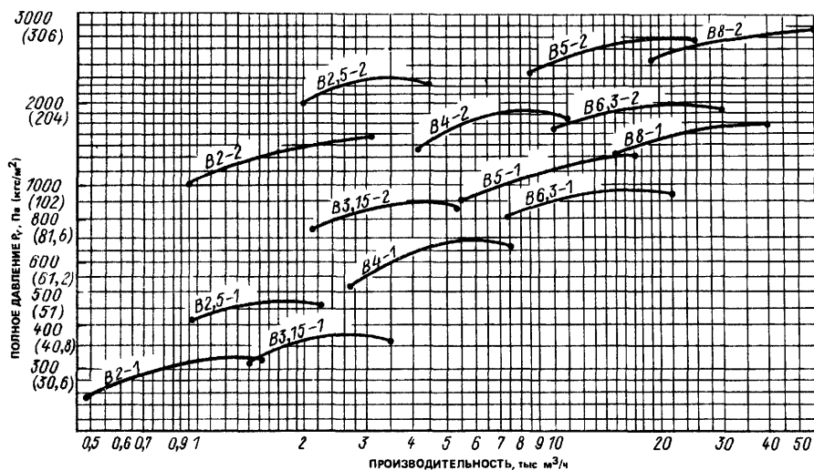
Рис. I.14. Сводный график характеристик вентиляторов В.Ц4-46 (исполнение 1)
