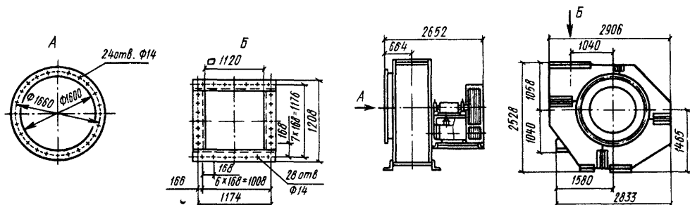
Рис. I.13. Вентилятор В.Ц4-75-16 (исполнение 6)
