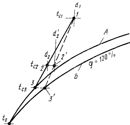
Рис 15.51 Схема процессов тепло- и влагообмена при орошении воздухоохладителя соляным раствором А и Б кривые насыщения соответственно над раствором и водой
