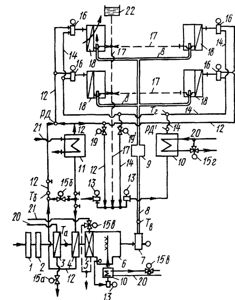
Рис. 15.19. Схема центральной одноканальной трехтрубной эжекционной СКВ с вводом к ЭКД холодного первичного воздуха, горячей и холодной воды.
