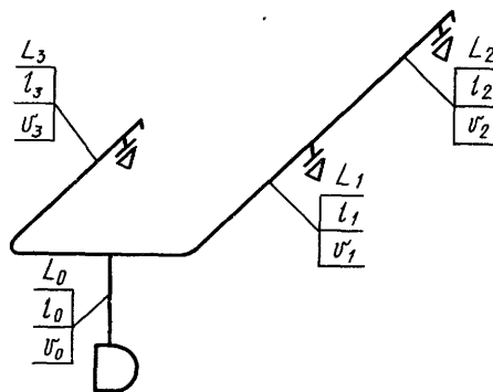
Рис. 22.3. Расчетная схема сети воздухопроводов для определения экономической целесообразной скорости воздуха
