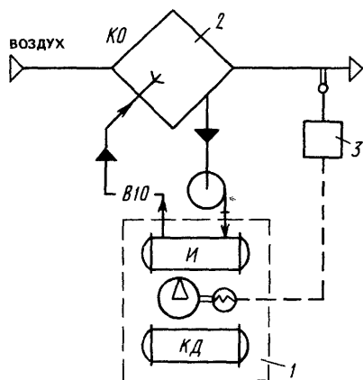
Рис 16.4. Одноконтурная схема присоединения воздухоохлаждающей машины к камере орошения
