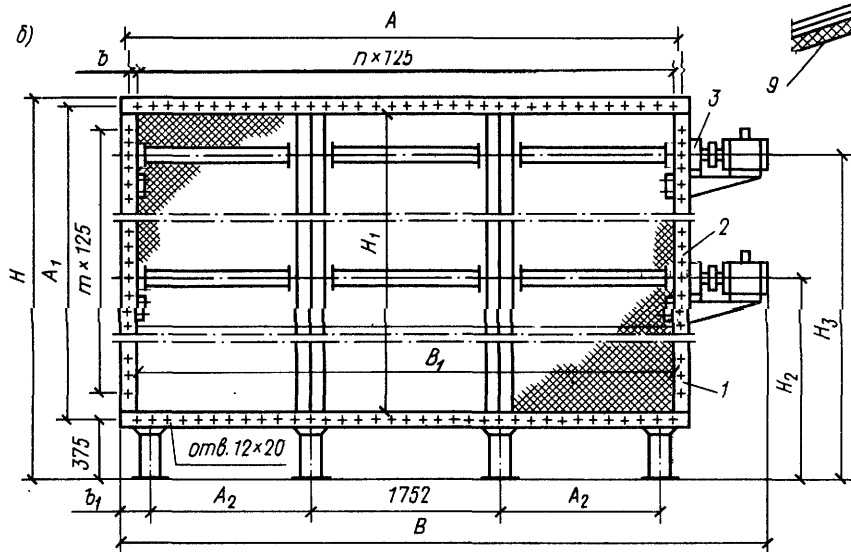
Рис. III.9. Фильтры воздушные ФР1-3
