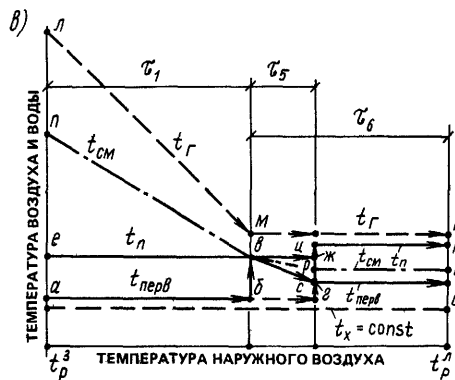
Рис 15.21 Графики изменения температуры первичного воздуха, холодной и горячей воды, поступающих к доводчикам одноканальных СКВ, поддерживающих в помещении температуру воздуха
