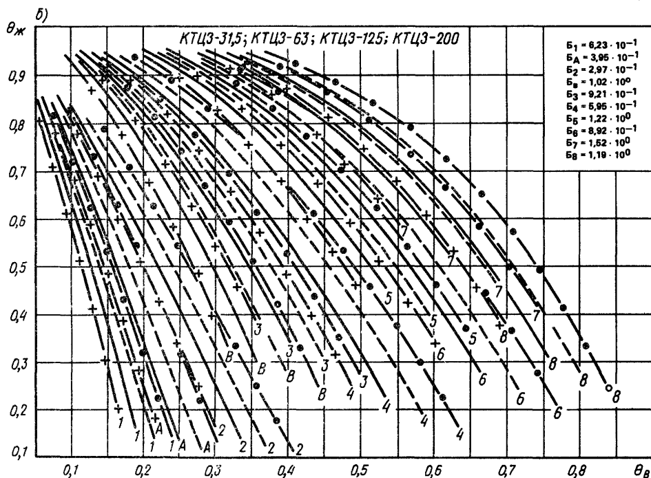
Рис. 15.41. Тепло технические и гидравлические характеристики теплообменников кондиционеров КТЦЗ-31,5; КТЦЗ-40; КТЦЗ-63; КТЦЗ-80; КТЦЗ-125; КТЦЗ-200 с параллельной схемой обвязки (а, в) и последовательно-противоточной (б, г)
