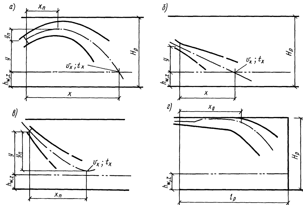
Рис. 17.3. Схемы подачи охлажденного воздуха вверх под углом к горизонтальной плоскости (а), нагретого воздуха вниз под углом к горизонтальной плоскости—ось струи пересекает РЗ (б) и ось струи выше РЗ (в), схема настилающей подачи охлажденного воздуха (г)
