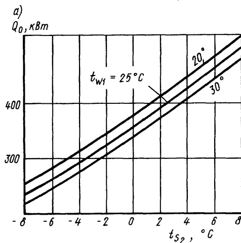
Рис. 16.2. Зависимости холодопроизводительности Q_0 от температуры хладонносителя t_{s2} и охлаждающей воды t_{w1} для хладоновой машины марки 21МКТ 280-2-1 (а) и 2МКТ 350-2-1 (б)
