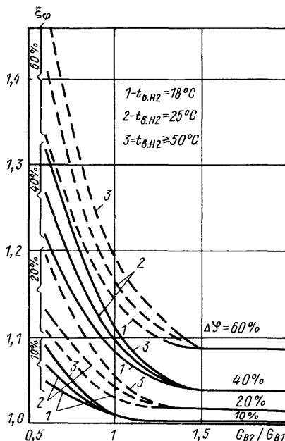
Рис. 21.10. Определение поправочного коэффициента \xi_\phi при \Delta\varphi = 10-60\%
