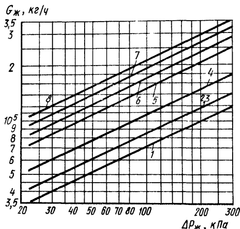
Рис. 15.35. Зависимость давления воды перед форсунками \Delta P_{\text{ж}} от расхода воды G_{\text{ж}} для камер орошения ОКС-3
