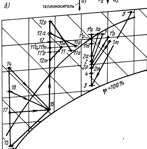
Рис. 15.10. Центральная прямооточная многозональная система кондиционирования воздуха, работающая полностью на наружном воздухе
