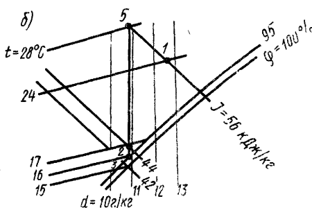
Рис. 17.9. Схемы процесса ассимиляции теплоты и влаги приточным воздухом для систем кондиционирования (а) и с увлажнением воздуха в помещении (б)
