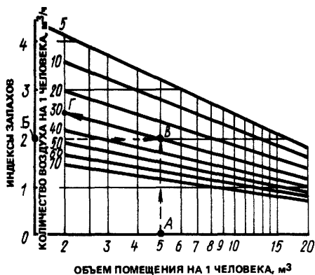
Рис. 15.4. Определение расхода наружного воздуха, необходимого для уменьшения интенсивности запахов, связанных с пребыванием в помещении людей 1 и 2 — ошутимый и умеренный запах; 3 и 4 — сильный и очень сильный запах
