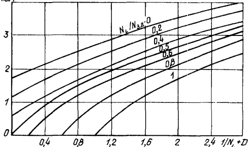
6.4. Зависимость B_{и.пом} от \left( \frac{1}{N_i} + D \right) и N_i / N_{зд}
