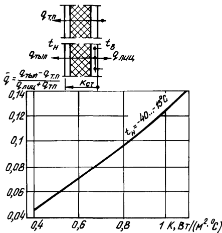
Рис. 13.13. Зависимость относительных дополнительных потерь тепла \bar{q} от коэффициента теплопередачи наружной стены K_{\text{ст}}
