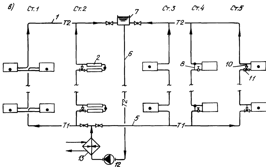
Рис. 10.7. Схемы вертикальных однотрубных систем насосного водяного отопления с верхней разводкой (а), с нижней разводкой (б) и с опрокинутой циркуляцией воды (в)
