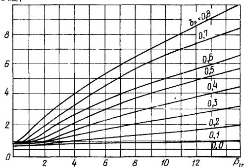
6.3. Зависимость B_{и.пом} от b_r и \bar{p}_в
