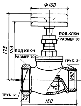
Вентиль запорный пожарный с муфтой и цапкой D_v = 50 мм латунный на p_v 0,6 МПа (6 кгс/см 2 ) 1Б 1р, применяемый на пожарных трубопроводах для воды с рабочей температурой до 50°С по ТУ 26-07-226-78
