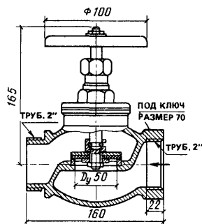
Вентиль запорный пожарный с муфтой и цапкой D_v = 50 мм латунный на p_v 0,6 МПа (6 кгс/см 2 ) 1Б 1р, применяемый на пожарных трубопроводах для воды с рабочей температурой до 50°С по ТУ 26-07-226-78
