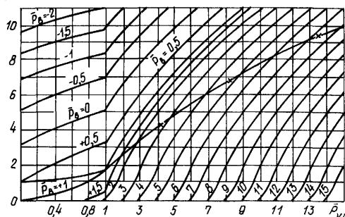
6.1. Зависимость B_{и.пом} от \bar{p}_{вн} и (\bar{p}_{вн}, \bar{p}_в)
