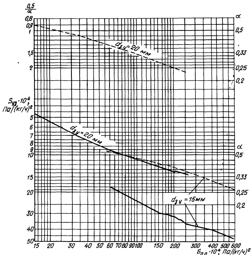
Рис. 10.25. Зависимость характеристики сопротивления S_{yz} \cdot 10^4 (сплошные линии) и коэффициента затекания \alpha (пунктирные линии) приборного узла со смещенным замыкающим участком в вертикальной однотрубной системе отопления от характеристик сопротивления подводки с прибором S_{yn} \cdot 10^4 ( d_{yz} - диаметр замыкающего участка)
