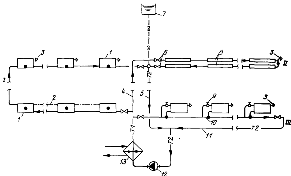
Рис. 10.8. Схема горизонтальной однотрубной системы насосного водяного отопления с ветвями
