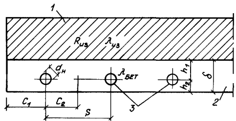
Рис. 13.14. Расчетная схема размещения нагревательных элементов в конструкции перекрытия (силовая плита)
