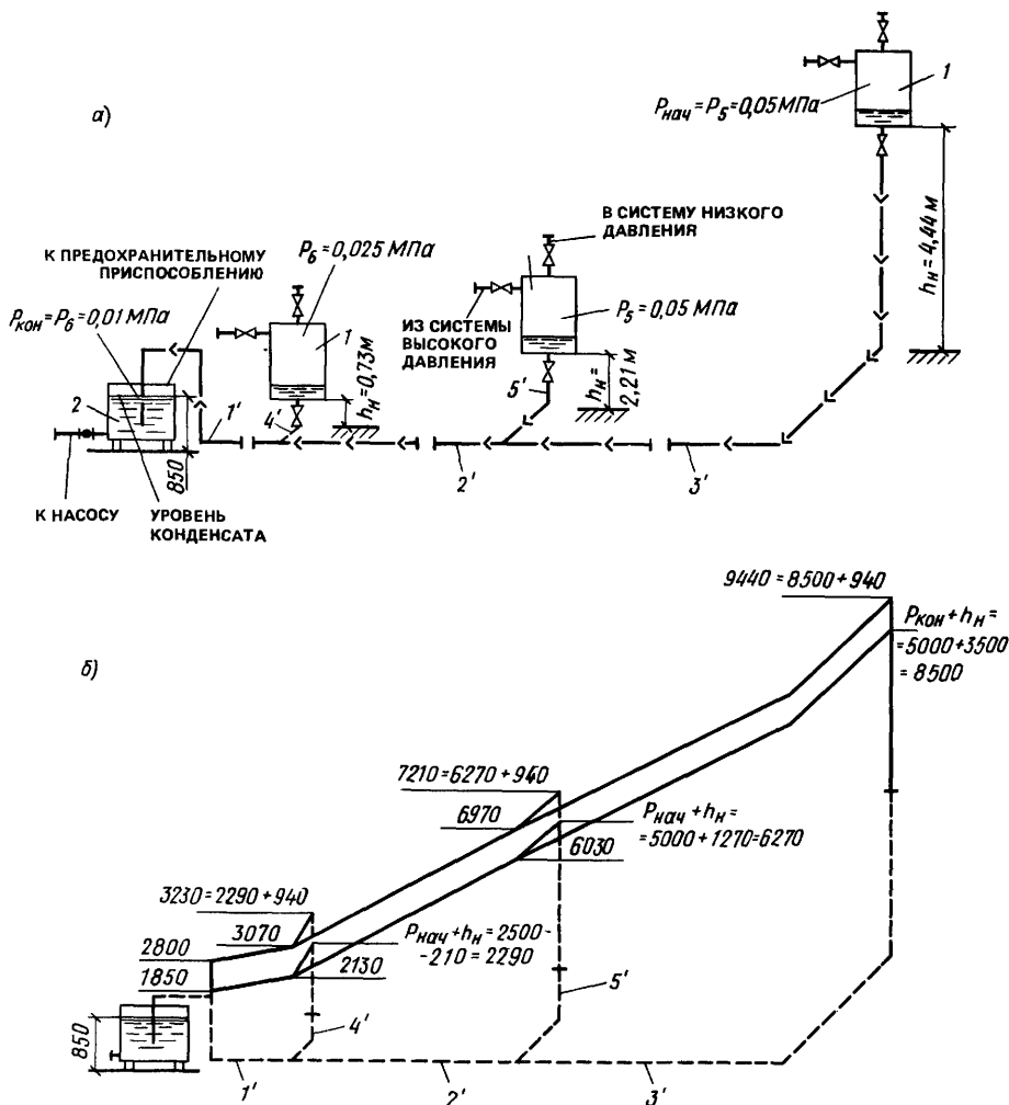
Рис. 11.10. Схема напорного конденсатопровода (а) от параллельно работающих расширительных баков и пьезометрический график (б) 1 — расширительный бак, 2 — конденсатный бак
