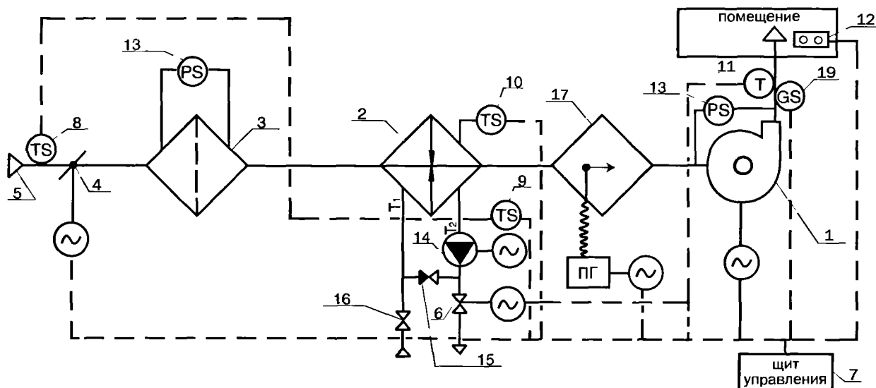
Приточная вентиляционная камера прямоточная с парогенератором
