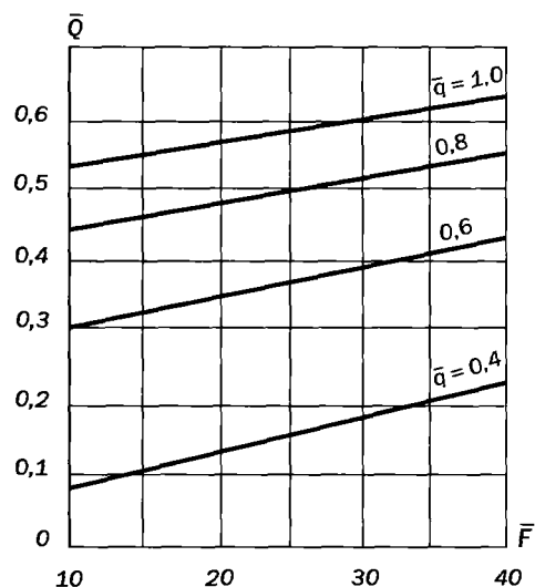
Рис. 7.4. График для определения потерь тепла с части струи завесы шибрующего типа, уходящей наружу: а — для боковой завесы; б — для нижней завесы
