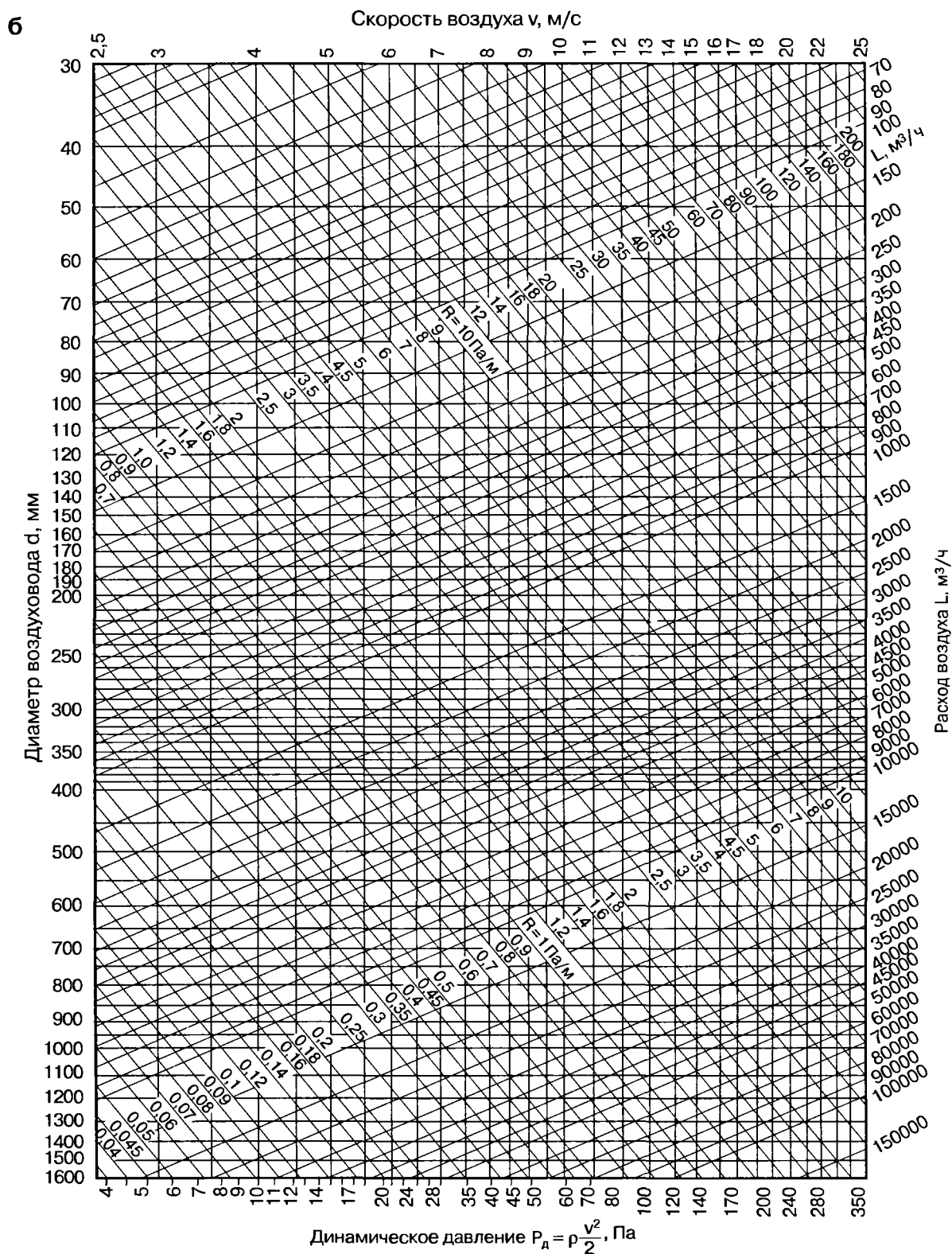
Рис. 8.6. Номограмма для определения потерь давления на трение в круглых воздуховодах механической вентиляции
