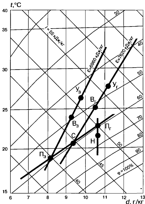
Рис. 6.2. Пример построения процессов на t - d диаграмме
