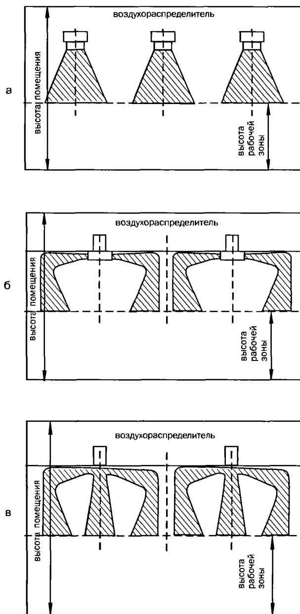
Рис. 9.4. Веерные струи:
