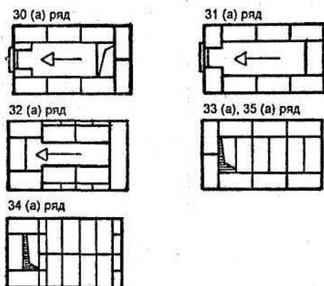
Рис. 3. Кладка простого камина с горизонтальным газоходом
