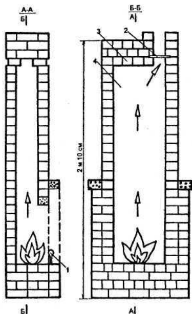
Рис. 1. Простой камин:
