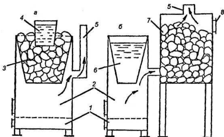
Рис. 4. Компактная печь-каменка:
