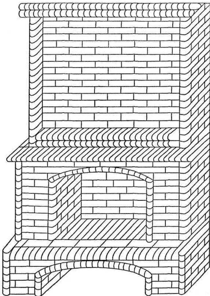
Рис. 7. Камин (конструкции В. В. Селивана)
