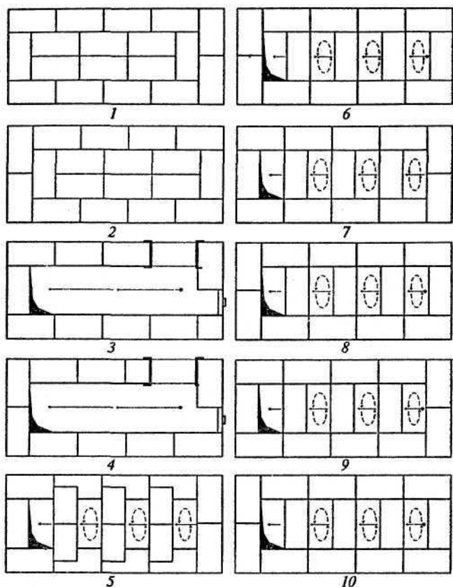
Рис. 3. Порядовка кладки отопительного щитка к банной печи
