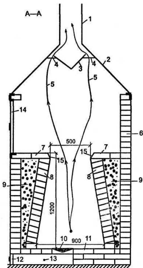
Рис. 12. Устройство печи — тандыра, разрез А—А:
