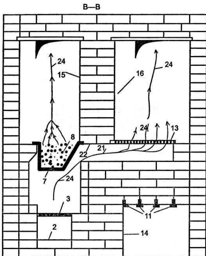
Рис. 20. Устройство двухкамерной коптильни в разрезе В—В (продолжение):
