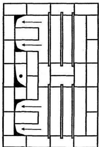
Рис. 22. Схемы кладки двухкамерной коптильни (окончание)
