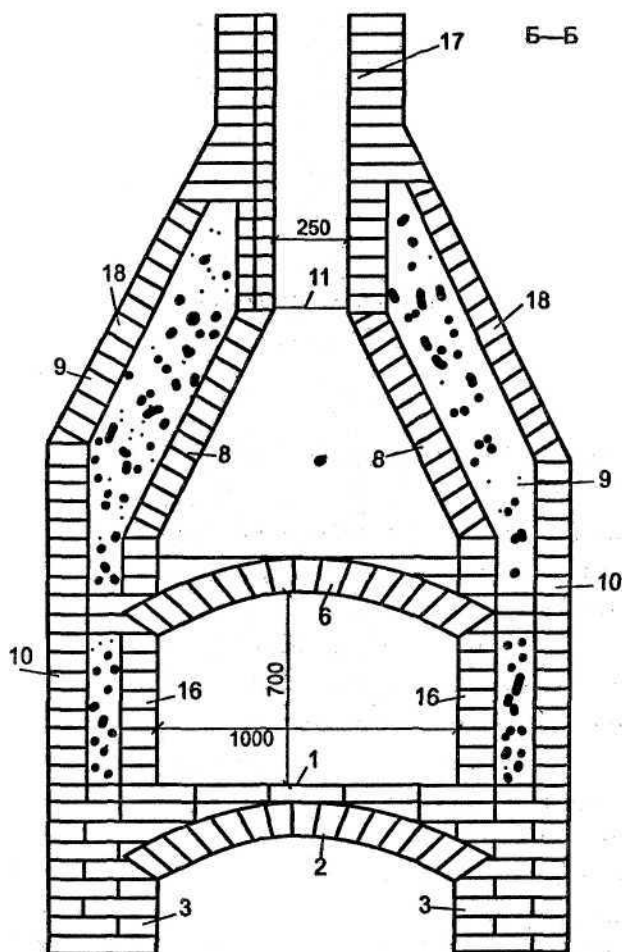
Рис. 29. Устройство уличного камина в разрезе Б — Б (продолжение):
