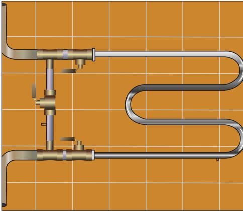
Рис. 12.72. Установленный байпас
