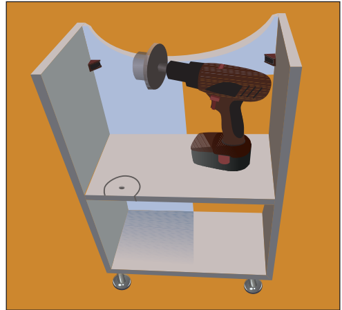
Рис. 10.60. Просверливаем отверстия под сифон и подводящие шланги воды (если они не были предусмотрены заранее)
