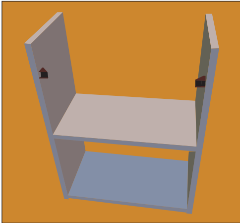
Рис. 10.58. Несобранная тумба
