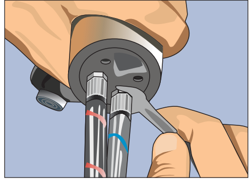
Рис. 10.25. Подсоединяем второй шланг гибкой подводки к смесителю (шланги подводки не затягиваем ключом туго)
