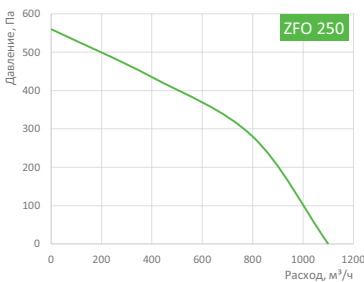
Условия испытаний L = 1050 м³/ч, Рст. = 30 Па
