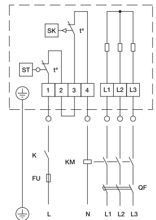
Схема 4 (400 В, 3 ф.)
