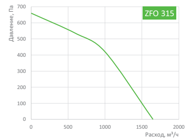
Условия испытаний L = 1500 м³/ч, Рст. = 60 Па
