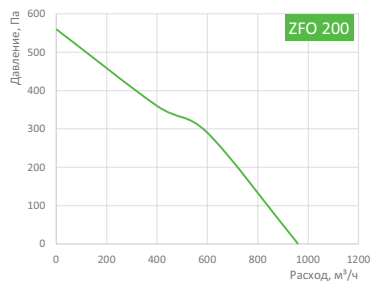
Условия испытаний L = 900 м³/ч, Рст. = 35 Па
