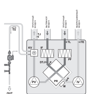
ZPVP 1000 VW, ZPVP 1500 VW, ZPVP 2000 VW
