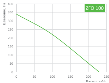
Условия испытаний L = 210 м³/ч, Рст. = 30 Па
