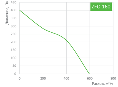
Условия испытаний L = 560 м³/ч, Рст. = 50 Па
