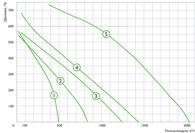
Условия испытаний 400 м³/ч, 250 Па ZPVP 450 HW
