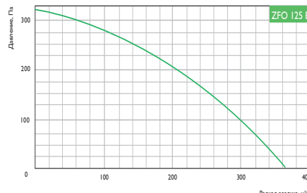
Условия испытаний 150 м³/ч, 210 Па
