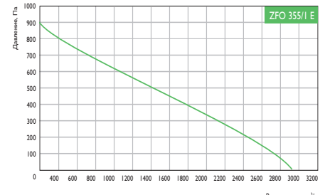
Условия испытаний 2230 м³/ч, 240 Па
