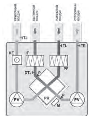
Модели: ZPVP 1000 VE, ZPVP 1500 VE, ZPVP 2000 VE
