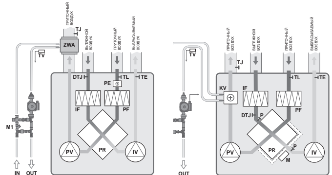
Модели: ZPVP 450 VW, ZPVP 800 VW
