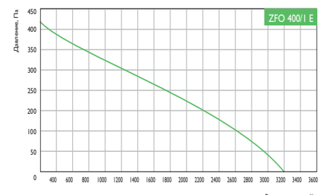
Условия испытаний 2200 м³/ч, 200 Па
