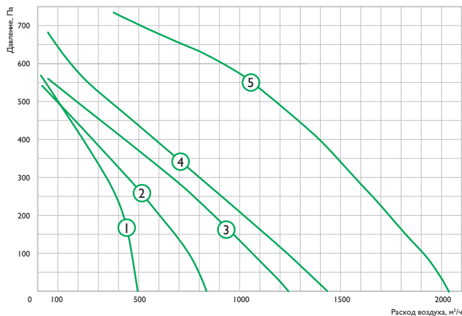
ZPVP 450 HW
