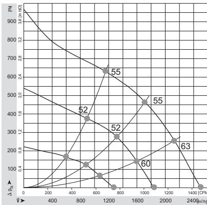
Характеристика вентилятора YMR-1-A (N=420 Вт/ 220/1/50)
