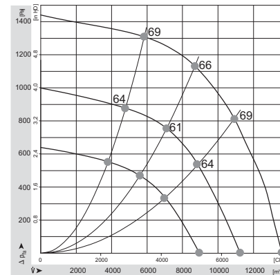
Характеристика вентилятора YMR-3-C (N=4300 Вт/ 380/3/50)
