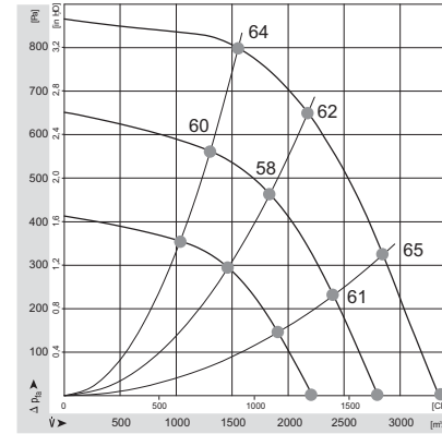
Характеристика вентилятора YMR-1-C (N=940 Вт/ 380/3/50)
