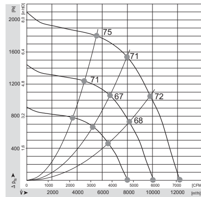
Характеристика вентилятора YMR-2-C (N=1850 Вт/ 380/3/50)
