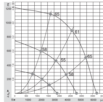
Характеристика вентилятора YMR-1-E (N=1700 Вт/ 380/3/50)
