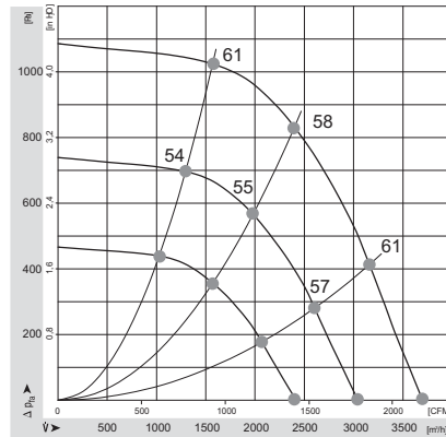
Характеристика вентилятора YMR-1-B (N=670 Вт/ 220/1/50)
