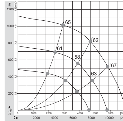
Характеристика вентилятора YMR-3-A (N=2825 Вт/ 380/3/50)
