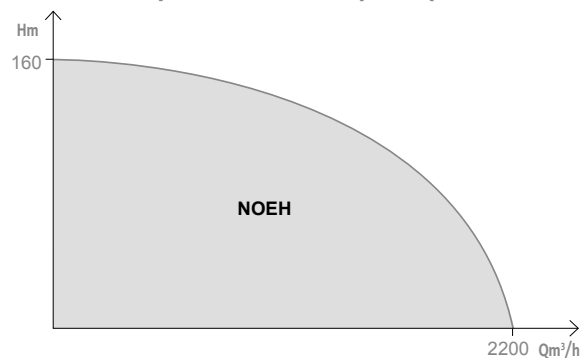
Гидравлические характеристики
