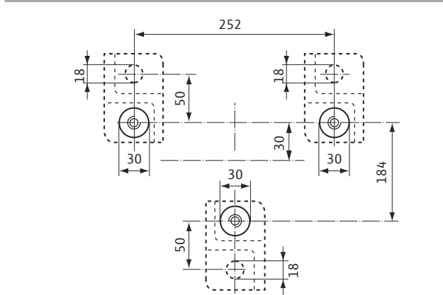
Схема консоли
