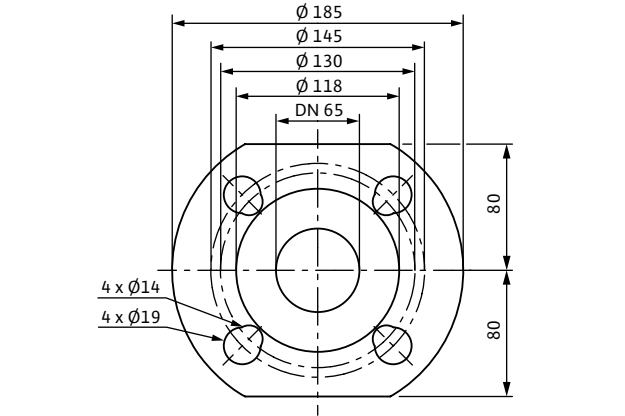
Габаритный чертеж фланца
