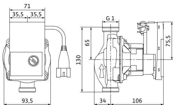
Габаритный чертеж Yonos PICO STG 25/1-7.5 180
