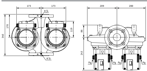
Габаритный чертеж TOP-SD 50/15 (3~400 В)
