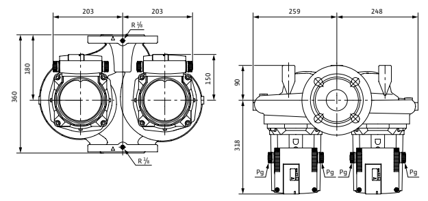
Габаритный чертеж TOP-SD 80/15 (3~400 В)
