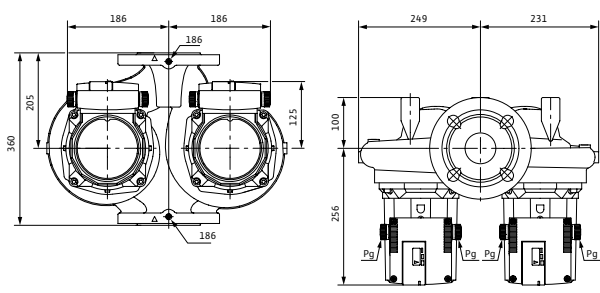
Габаритный чертеж TOP-SD 80/10 (3~400 В)
