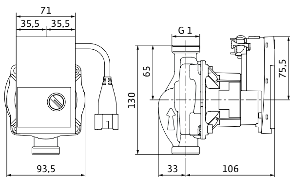
Габаритный чертеж Yonos PICO STG 15/1-13 180
