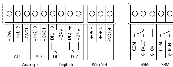
Схема подключения
