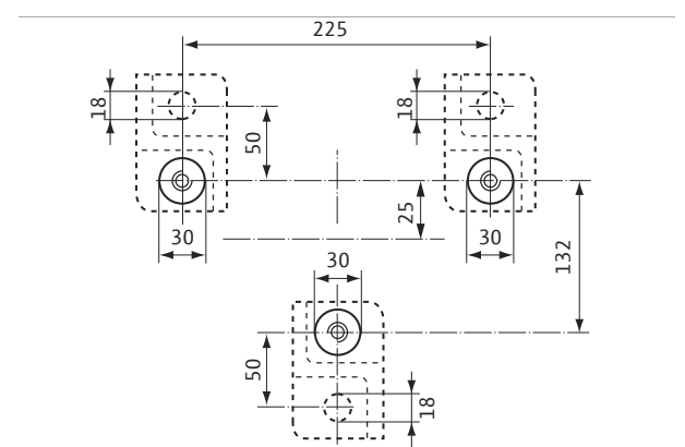
Схема консоли
