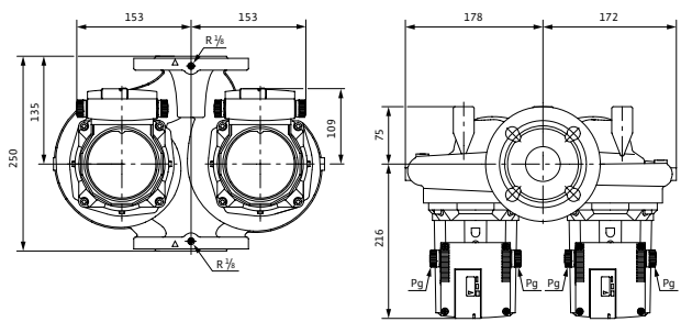
Габаритный чертеж TOP-SD 40/7 (3~400 В)
