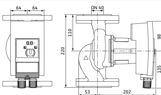
Габаритный чертеж Yonos MAXO-Z 40/0,5-8
