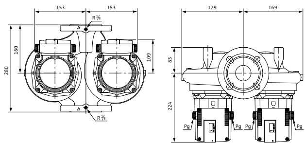
Габаритный чертеж TOP-SD 50/7 (3~400 В)
