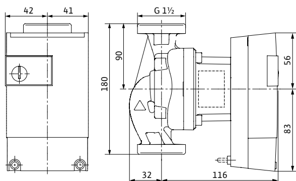
Габаритный чертеж Yonos ECO 25/1-5 BMS
