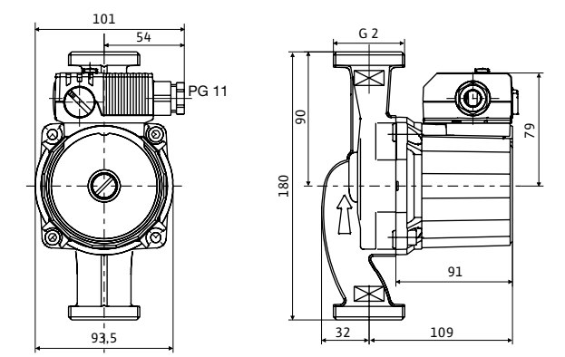
Электродвигатель в горизонтальном положении. Возможные положения клеммной коробки: 3,6,9 и 12 часов.
