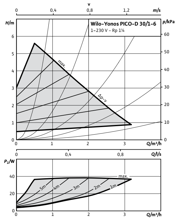
Характеристика \Delta p -v (перемен.)
