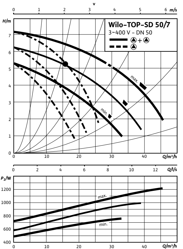
Характеристика. Трехфазный ток – работа двух насосов
