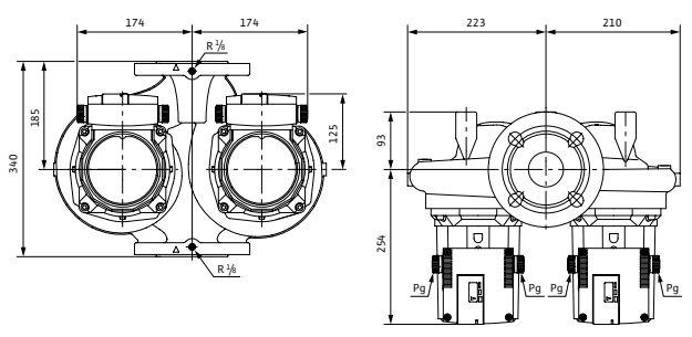
Габаритный чертеж TOP-SD 65/15 (3~400 В)
