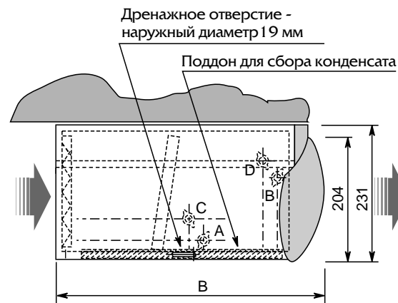
ВИД СБОКУ
