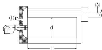
Реверсивный котел
