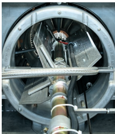
Смесительное устройство
