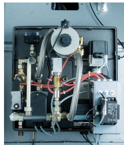
Управляющий агрегат
