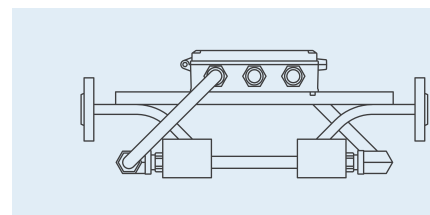
ИУ-х32 – U-образный измерительный участок с врезными датчиками
