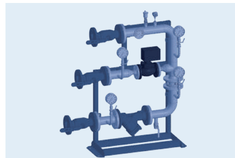
Модуль ГВС для открытой системы теплоснабжения с регулирующим клапаном и линией циркуляции
