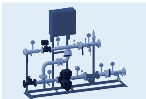
Модуль отопления – зависимая схема со сдвоенным насосом в обратном трубопроводе
