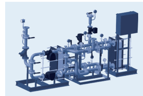
Модуль отопления – независимая схема с двумя ТО и двумя насосами циркуляции отопления
