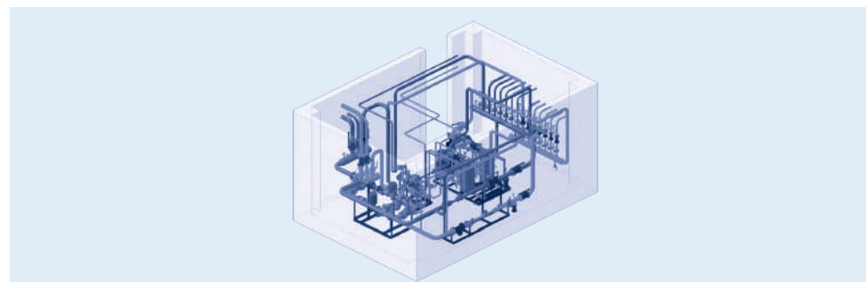
Тепловой пункт здания с узлом учета тепловой энергии и обвязкой модулей отопления и ГВС
