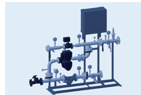
Модуль отопления – зависимая схема со сдвоенным насосом на перемычке
