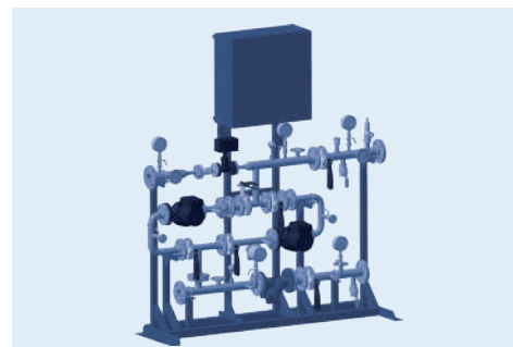
Модуль отопления – зависимая схема с двумя насосами на перемычке
