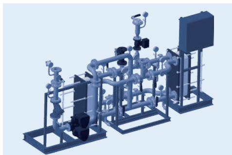
Модуль отопления – независимая схема с двумя ТО и сдвоенным насосом (вариант исполнения)
