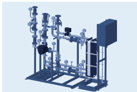
Модуль ГВС для закрытой системы теплоснабжения с одним ТО и циркуляционным насосом
