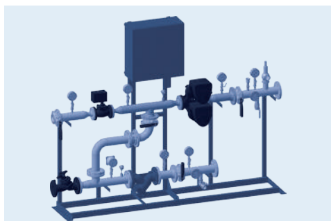
Модуль отопления – зависимая схема со сдвоенным насосом в подающем трубопроводе
