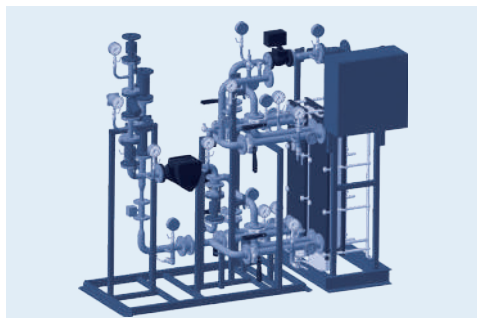
Модуль ГВС для закрытой системы теплоснабжения с двумя теплообменниками (ТО)
