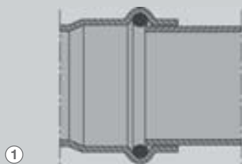
1 Фитинг Viega с цилиндрической направляющей.
