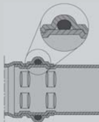
3 Опрессованный фитинг Viega в разрезе.
