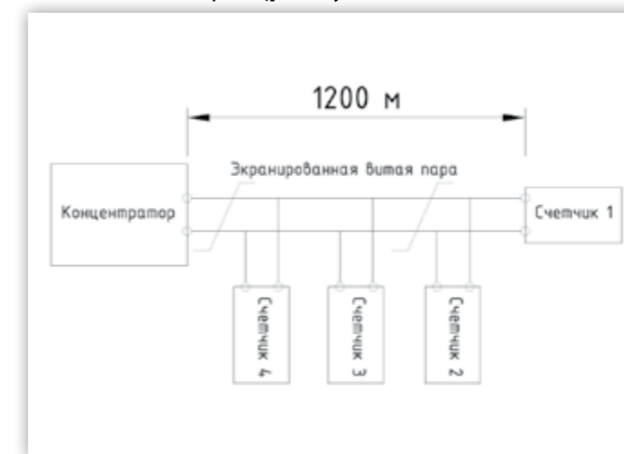
Рис. 2. Предельная длина проводной сети
