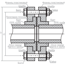
Схема фланцевого соединения
