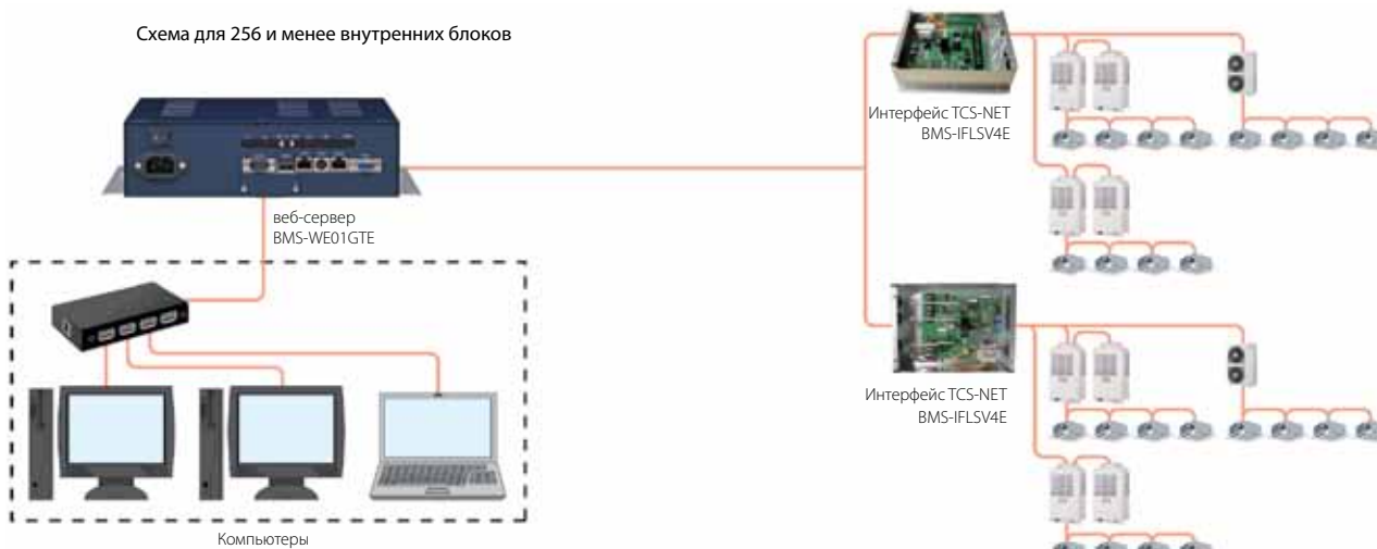
Схема для 256 и менее внутренних блоков
