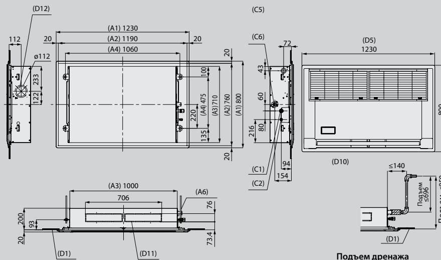
(размеры: мм)
