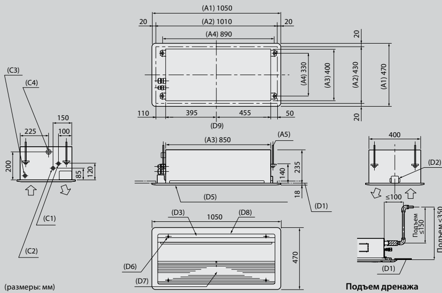
(размеры: мм)
