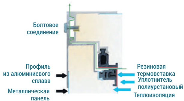
Лабиринтное уплотнение
