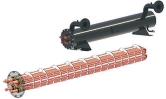
Кожухотрубный испаритель
