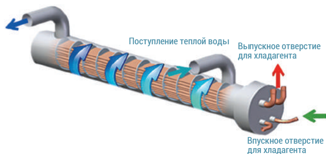
Кожухотрубный испаритель
