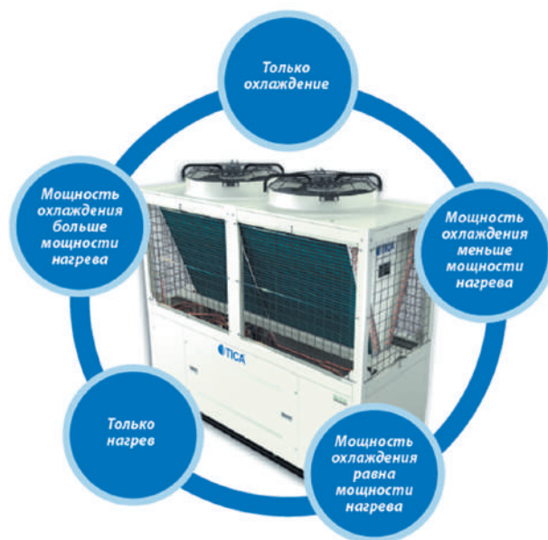
Варианты работы четырехтрубного чиллера
