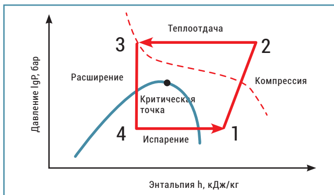
Транскритический цикл CO_2
