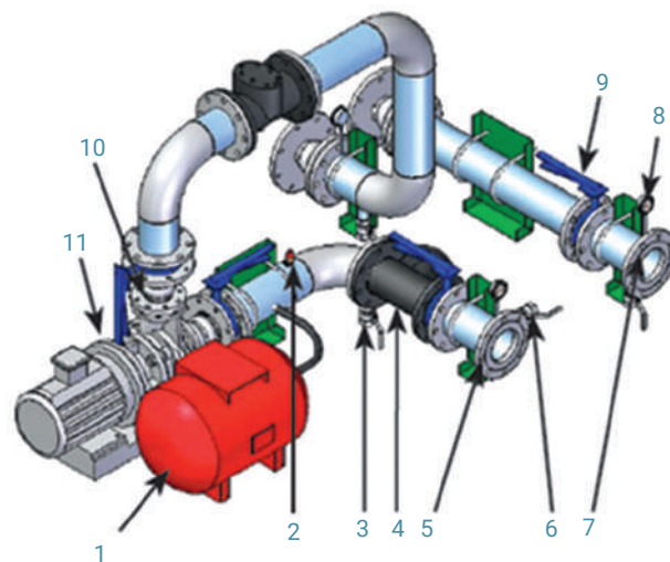
Гидравлический модуль
