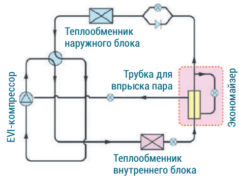
Схема теплового насоса (чиллера) с технологией EVI
